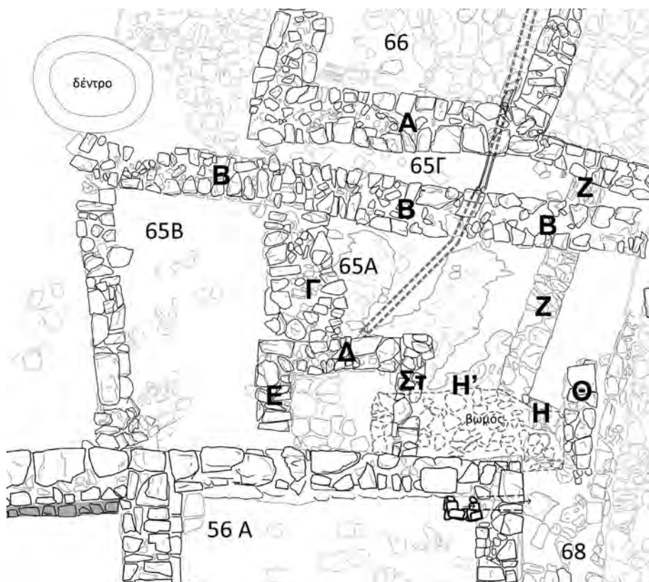
Σχ. 3. Κάτοψη του Χώρου 65.
