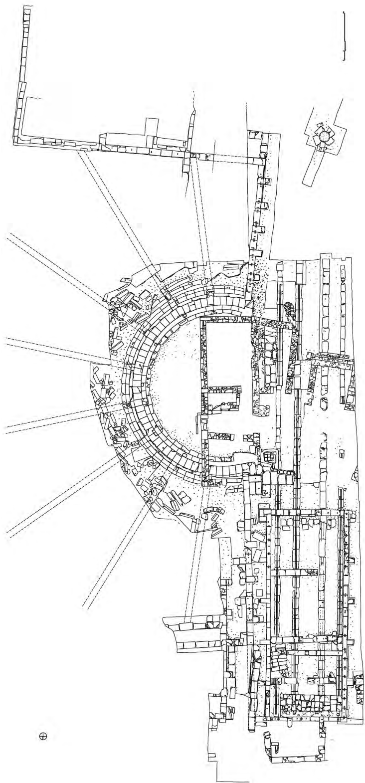
Σχ. 1. Σχεδιαστική κάτοψη του αρχαίου θεάτρου (αρχιτέκτων Γ. Νίνος).
