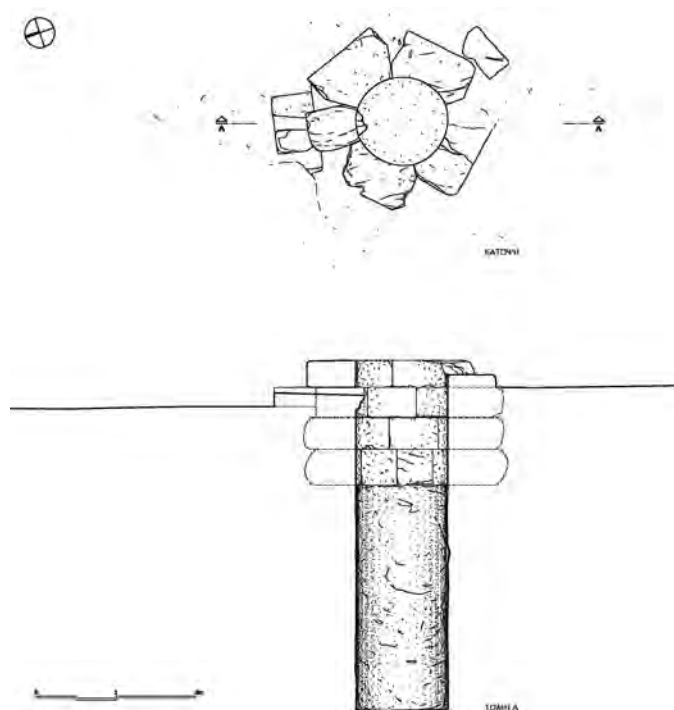
Σχ. 3. Κάτοψη και τομή του φρέατος (ἀρχιτέκτων Γ. Νίνος).
