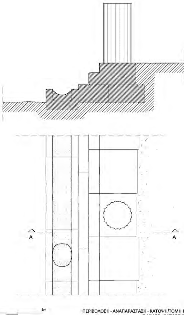
Σχ. 6. Αναπαράσταση «Περιβόλου II», κάτοψη και τομή (ἀρχιτέκτων Γ. Νίνος).
