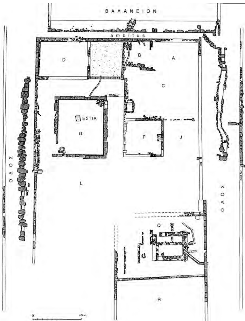
Εἰκ. 4. Κάτοψη τοῦ Ἱεροθύσιου.
