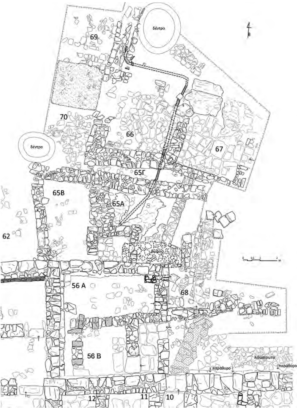
Σχ. 2. Κάτοψη των ανασκαφέντων κατά τὸ 2020 χώρων.
