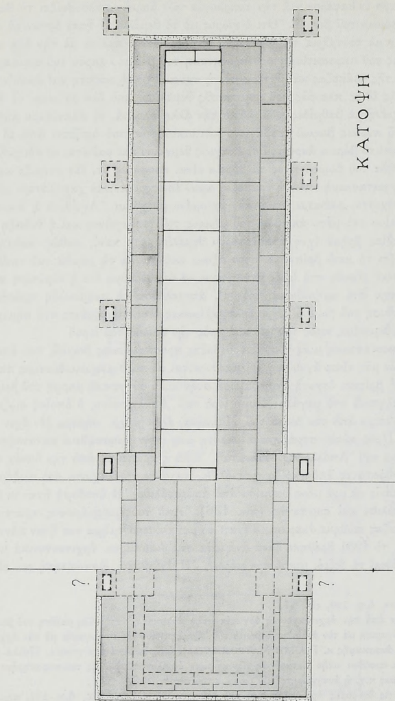
Εικ. 9. Σχέδιο ἐργασίας γιὰ τὴν ἀποκατάσταση τῆς κατόψεως τοῦ βωμοῦ τοῦ Ἀπόλλωνος.
