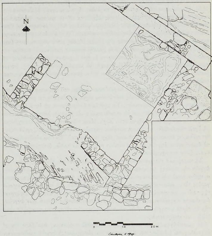
Εἰκ. 4. Σχέδιον δωματίου οἰκίας ἀνασκαφείσης εἰς τὴν «Κάτω Πόλιν» χρονολογουμένης εἰς τὸν 4ον π.Χ. αἰῶνα.
