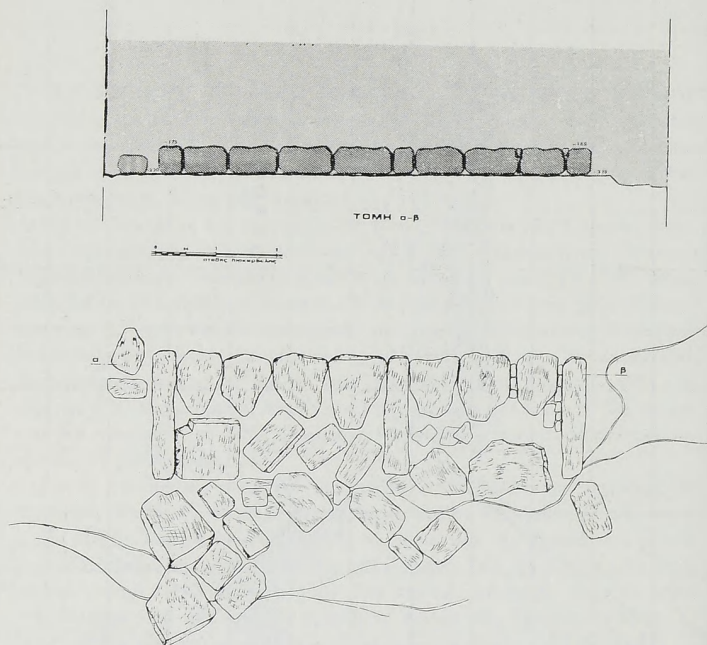
Εἰκ. 2. Κάτοψη καὶ τομὴ τμήματος κτιριακῆς κατασκευῆς τοῦ τομέα Α, στὴ θέση Ι, τῆς εἰκ. 1.
