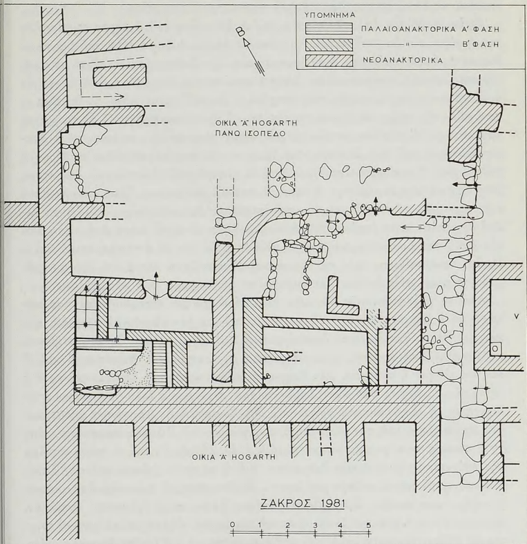
Εἰκ. 3. Ὑψώϊσπεδο Οἰκίας Α Hogarth.
