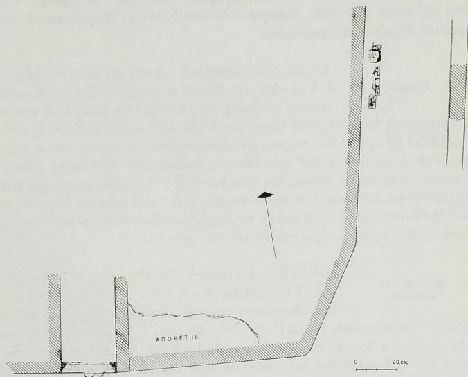
Εἰκ. 11. Τὸ πρότυπο τοῦ γυμνασίου Ραμνοῦντος, ὁ ἀποθέτης καὶ ὁ ἀνατολικὸς δρόμος μετὰ βάθρα (σχ. Ἀπ. Θωμοπούλου).
