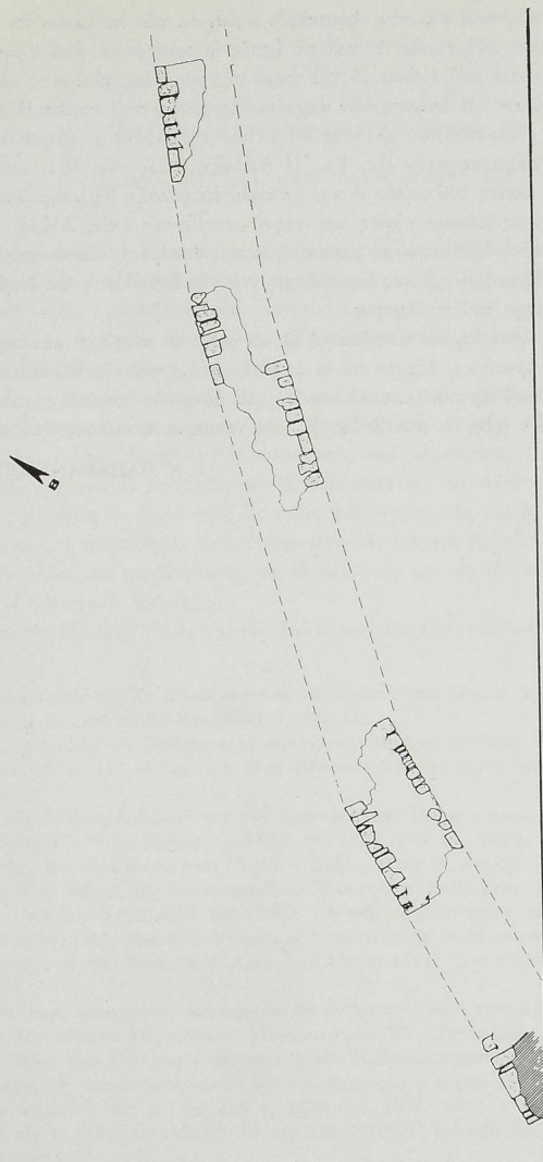
Εικ. 3. Κάτοψη τών όρίων καί τών όρατῶν, πάνω ἀπό τήν ἐπιφάνεια τῆς θάλασσας, τμημάτων τοῦ μεταγενέστερου (μεσαιωνικοῦ) λιμενικοῦ ἔργου στὸν τομέα Β τῆς εἰκ. 1.
