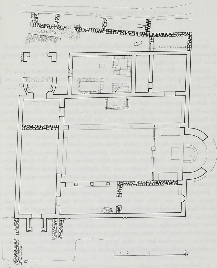
Εἰκ. 1. Κάτοψη τῆς βασιλικῆς Ἀγίας Σοφίας Μύτιμα.
