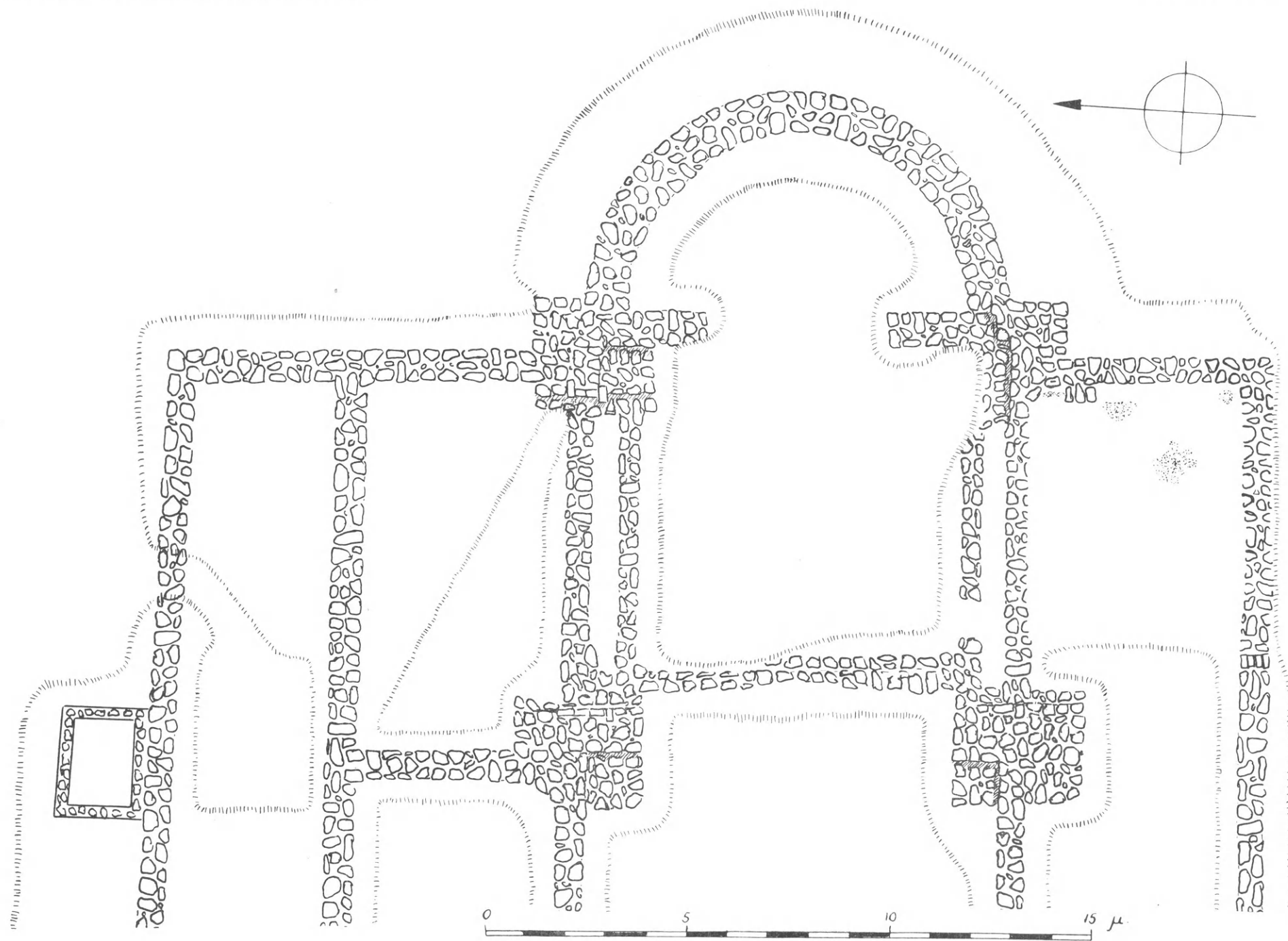
Κάτοψις τοῦ Α τμήματος τῆς βασιλικῆς τοῦ Ἰλίουσοῦ μετὰ τὰς ἐργασίας τοῦ 1948.
