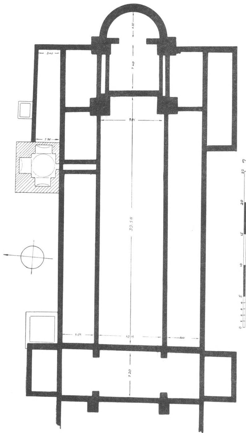
Εἰκ. 9. Κάτοπις τῶν θεμελίων τῆς βασιλικῆς (1948) συμπληρωμένη κατὰ τὴν κάτοπιν ΑΕ 1919, εἰκ. 3, καὶ Γ. Σωτηρίου, Χριστ. καὶ Βυζ. Ἀρχαιολ., εἰκ. 180.
