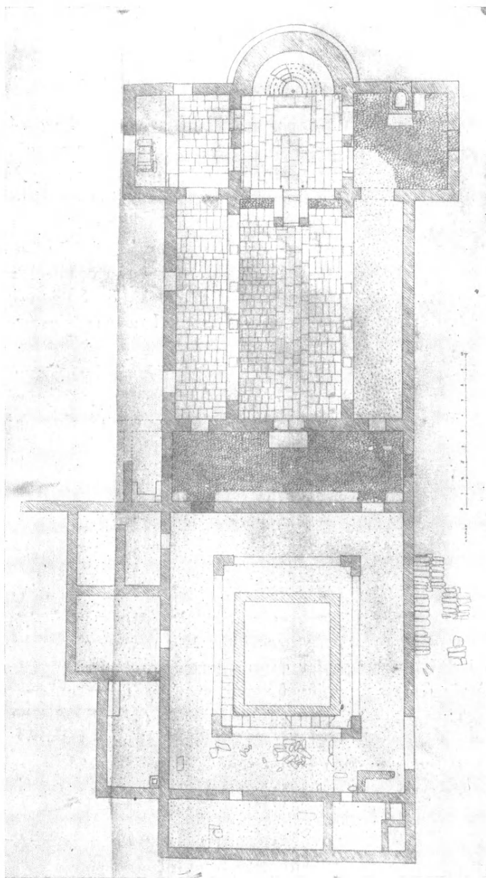
Εἰκ. 1. Κάτοψις τῆς παλαιοχριστιανικῆς βασιλικῆς Πανόρημου.
