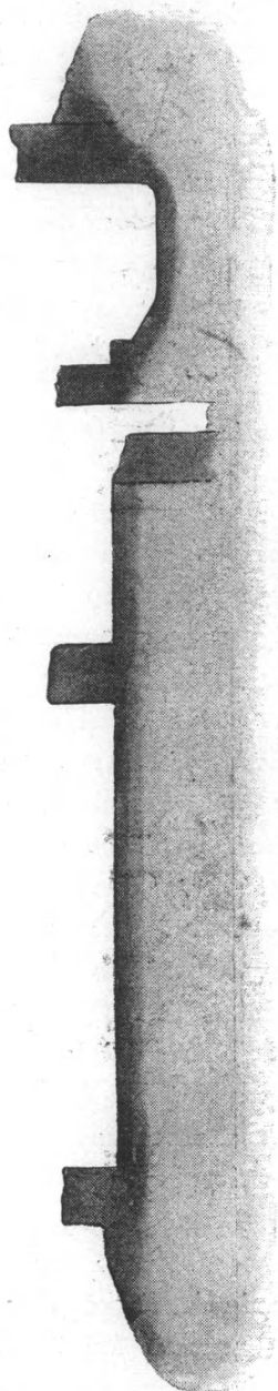
ΤΟΜΗ Α - Β
