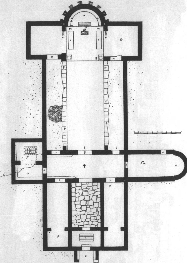
Πίν. I. Κάτοψις Χριστιαν. Βασιλικῆς Δομειτίου ἐν Νικοπόλει.
