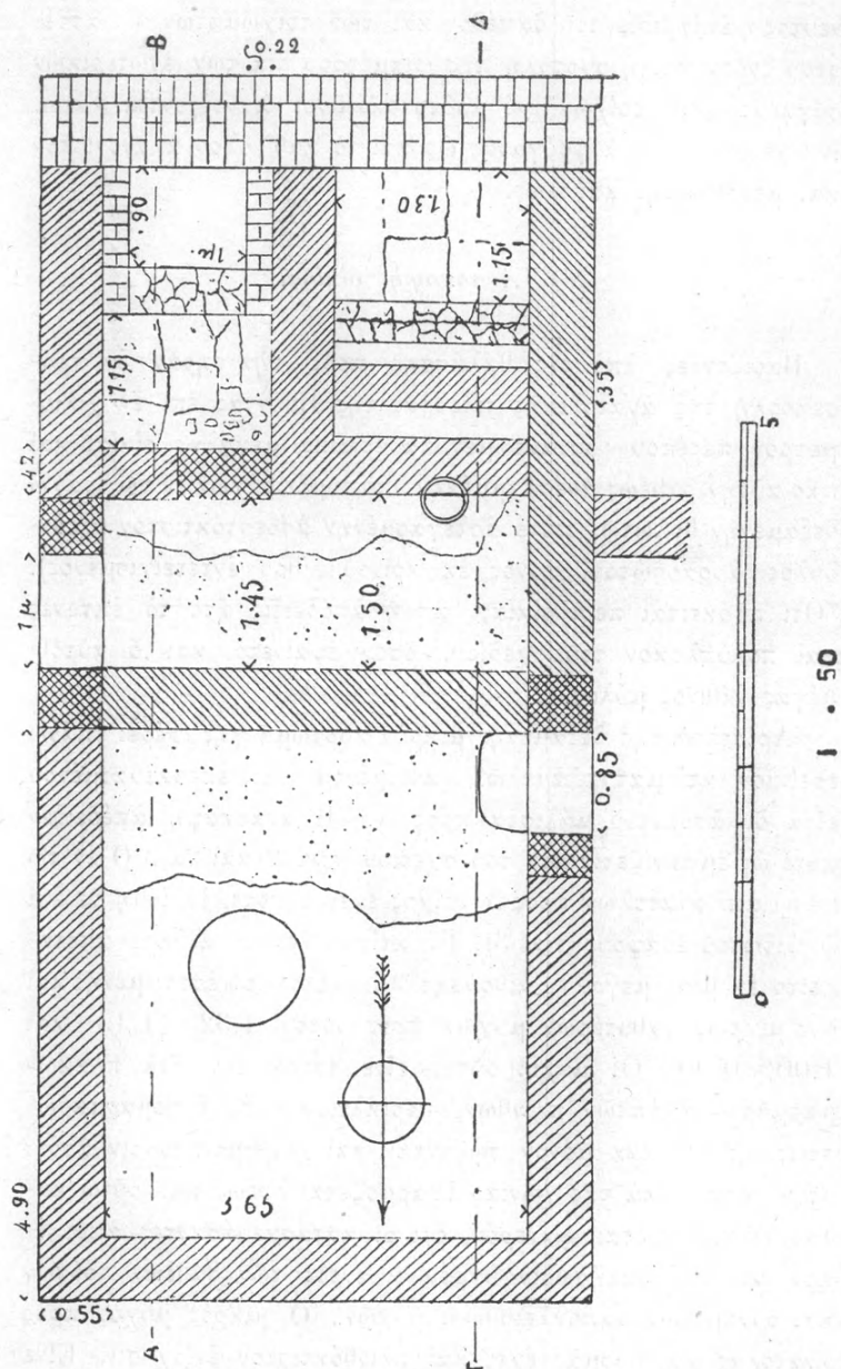
Εἰκ. 2. Κάτοψις μέρους οἰκίας ἐν Λιξωνίᾳ Ἀττικῆς.
