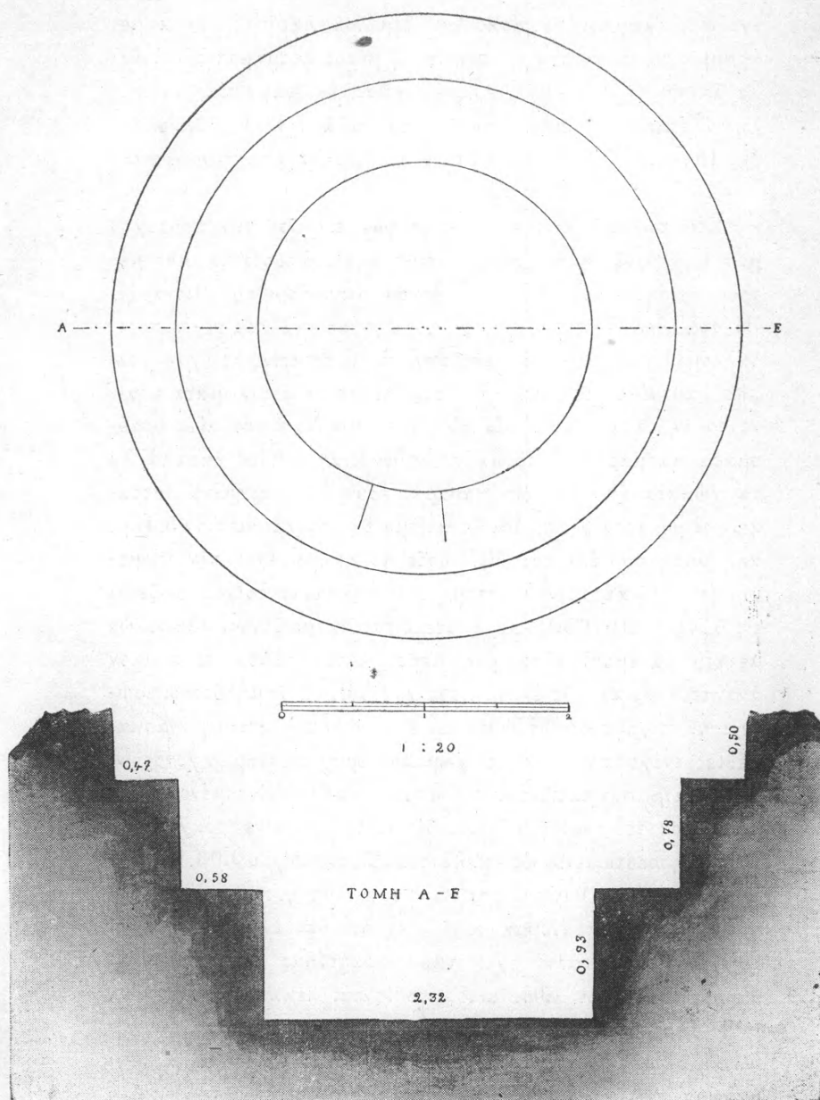
Εἰν. 1 Κάτοψη καὶ τομὴ περιφεροῦς κτίσματος Αἰξωνῆς
