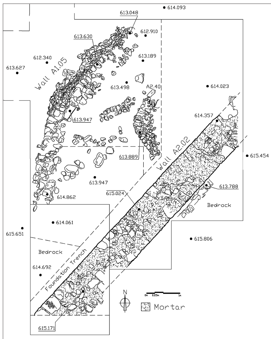
Λύκτος Ηρακλείου Κρήτης. Τοπογραφικό σχέδιο του τομέα Α.
