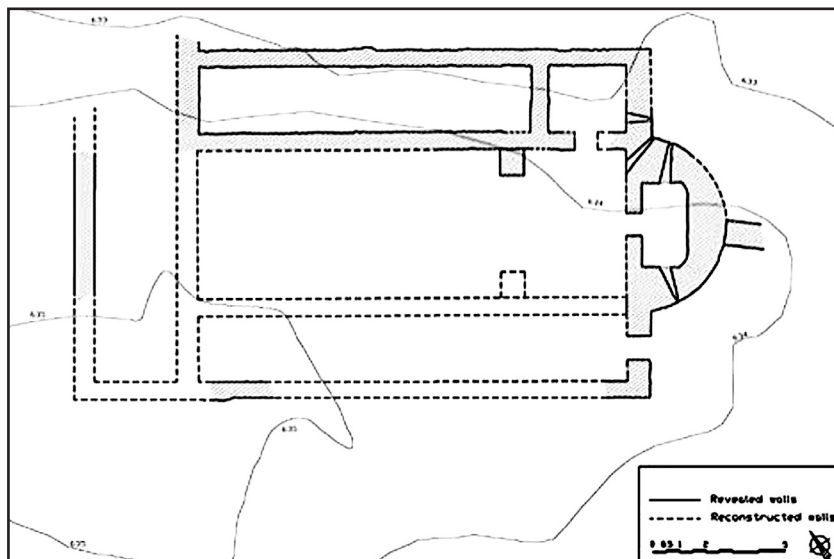
Λύκτος Ἡρακλείου Κρήτης. Κάτοψη τῆς πρωτοβυζαντινῆς βασιλικῆς τοῦ τομέα Γ.
