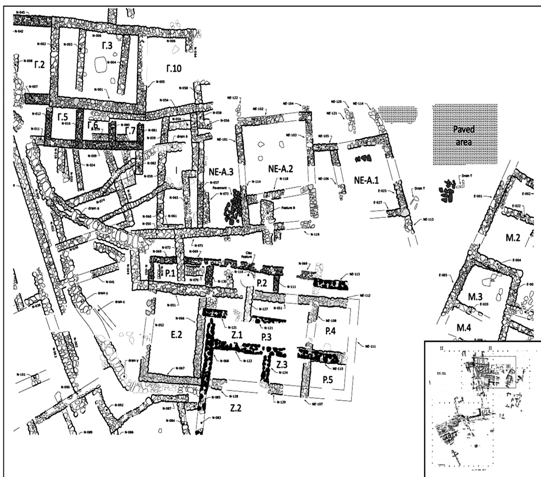
Τελαινα Μεσσηνίας. Κάτοψη των κτισμάτων που ανασκάφηκαν το 2022 (Michael Nelson). Πιο έντονα δηλώνονται τα κτίσματα της YE IIIB, ενώ τα υπόλοιπα είναι της YE IIIA2.
