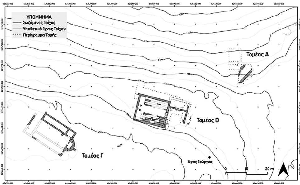
Λύκτος Ήρακλείου Κρήτης. Τοπογραφικό σχέδιο της ακρόπολης με τούς τομείς Α, Β, Γ.
