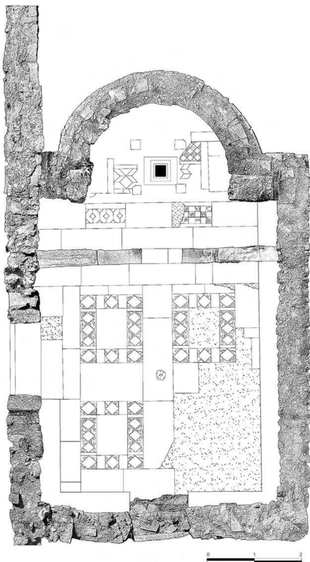
Σικυνῶν (Κιάτο). Τὸ νοτιοανατολικὸ παρεκκλήσιο, κάτοψη.
