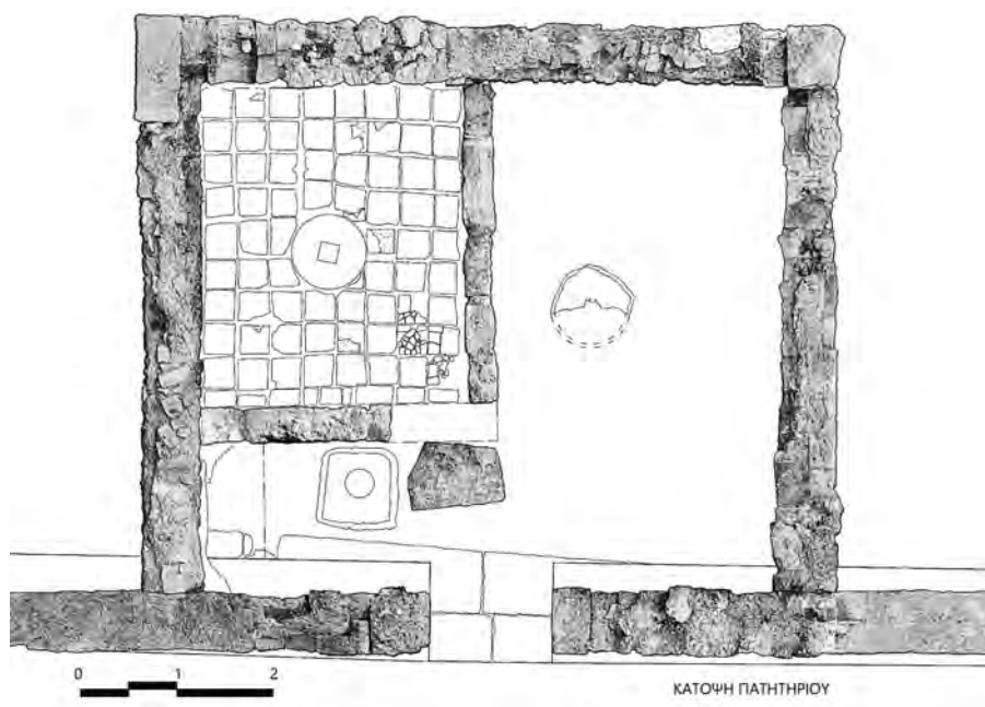
Σικυνών (Κιάτο). Τὸ βόρειο πρόσκτισμα τοῦ κυρίως ναοῦ, κάτοψη.
