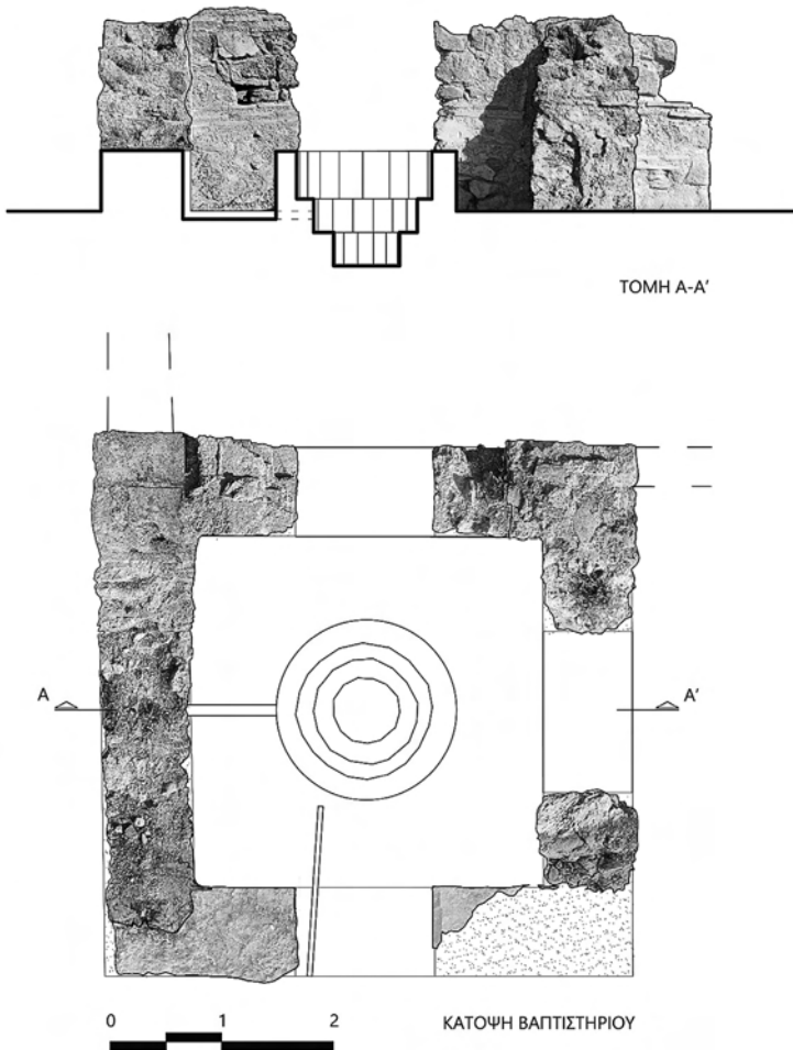
Σικυῶν (Κιάτο). Τὸ φωτιστήριον τῆς βασιλικῆς, κάτοψη καὶ τομή.
