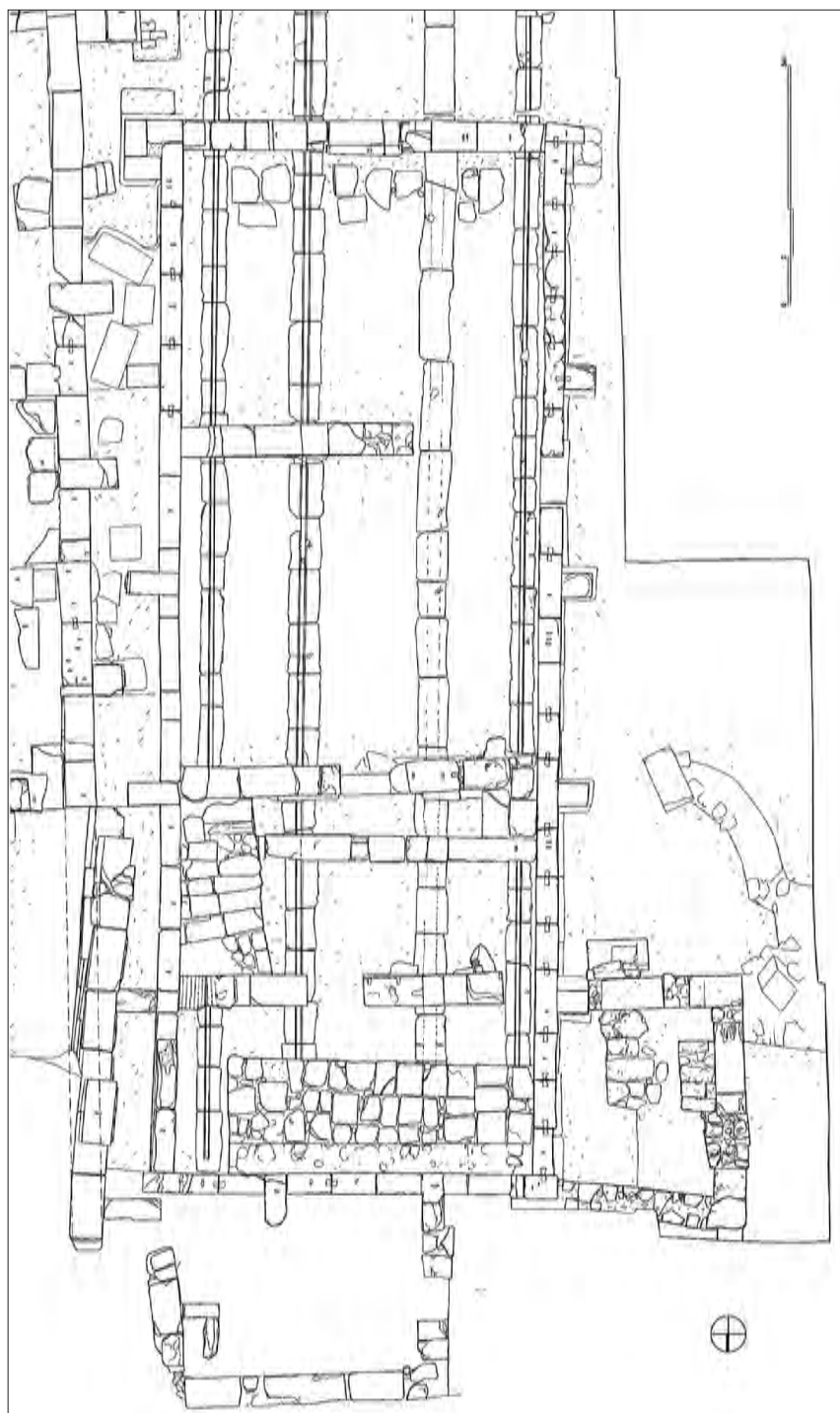
Θουρία. Κάτοψη της σκηνοθήκης του αρχαίου θεάτρου, 2021 (ἀρχιτέκτων Γ. Νίνος).
