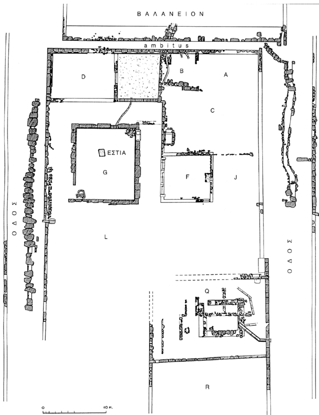
Μεσσήνη. Κάτοψη του ἱεροθύσιου.
