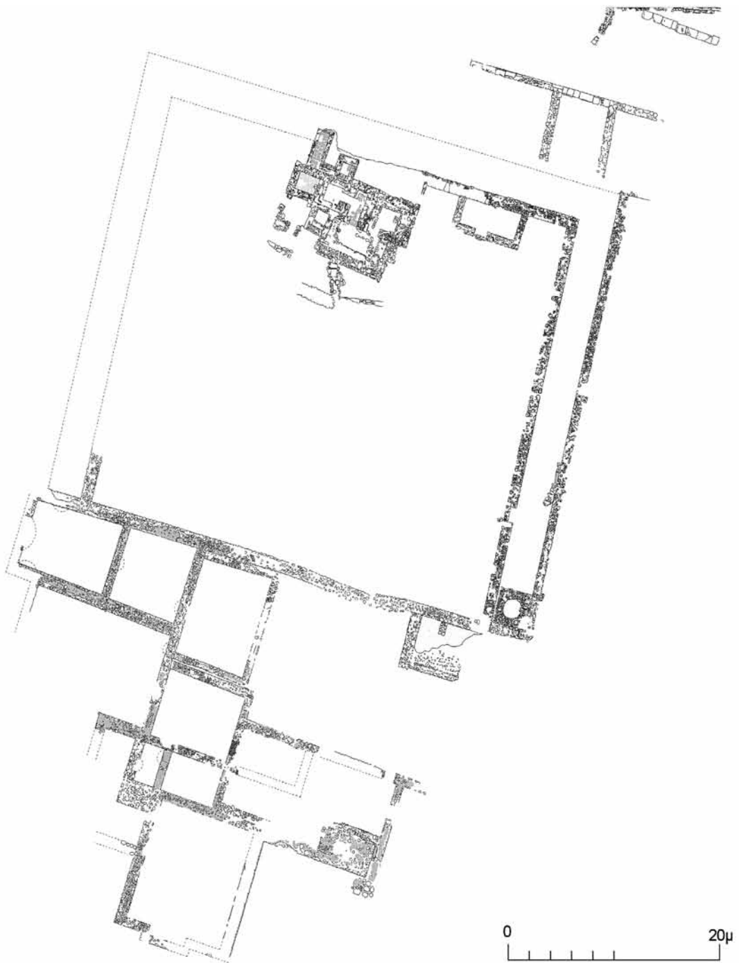
Μεσσήνη. Κάτοψη του ἱεροῦ τῆς Ἰσιδος.
