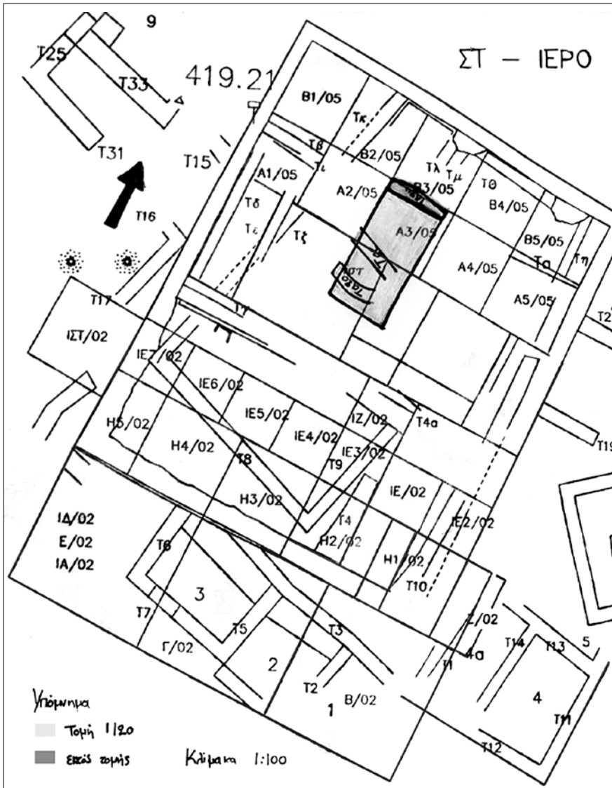
Άγ. Ανδρέας Σίφνου. Απόσπασμα τοπογραφικού διαγράμματος του Τερού με την Τομή 1/20 (αποτύπωση-σχεδίαση: Θ. Χατζηθεοδώρον, Μαρία Μπία, Γ. Γαβαλάς).
