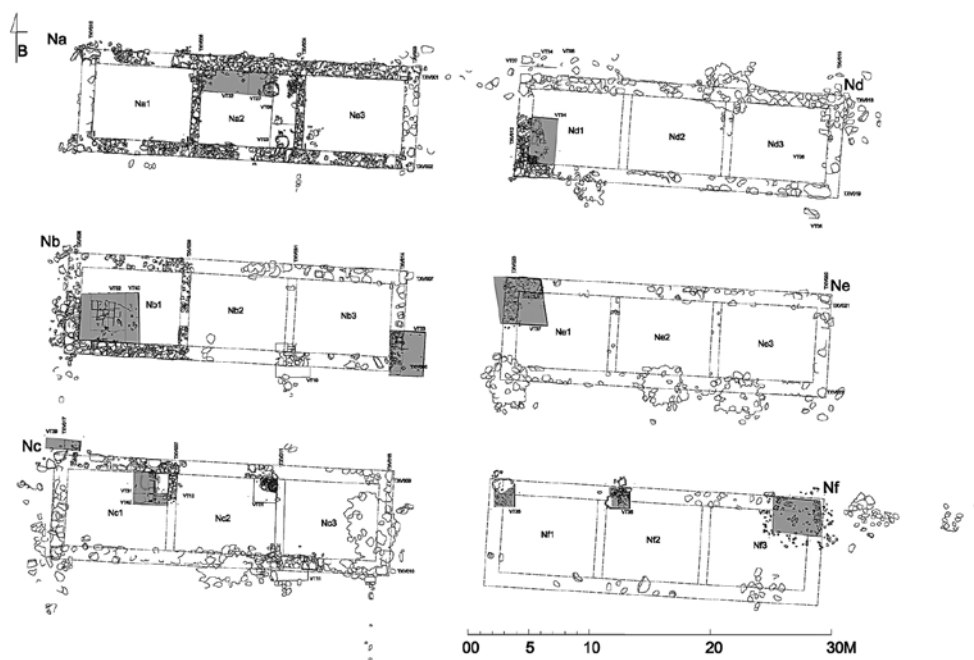
Μυκηναϊκή ἀκρόπολη Γλᾶ. Κάτοψη τοῦ Κτιριακοῦ Συγκροτήματος Ν με ἐνσωματωμένες τὲς ἀνασκαφικὲς τομὲς τοῦ 2020.
