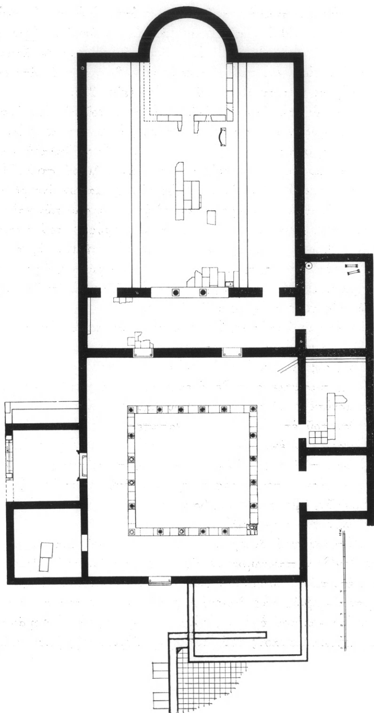
Εἰκ. 24. Χρυστ. Ἀμφίπολις. Κάτοψις τῆς βασιλικῆς Δ.
