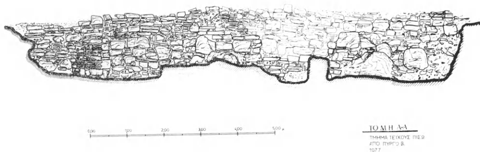
Εἰκ. 90. Σίφνος. Τομὴ τείχους πίσω ἀπὸ τὸν πύργο β.
