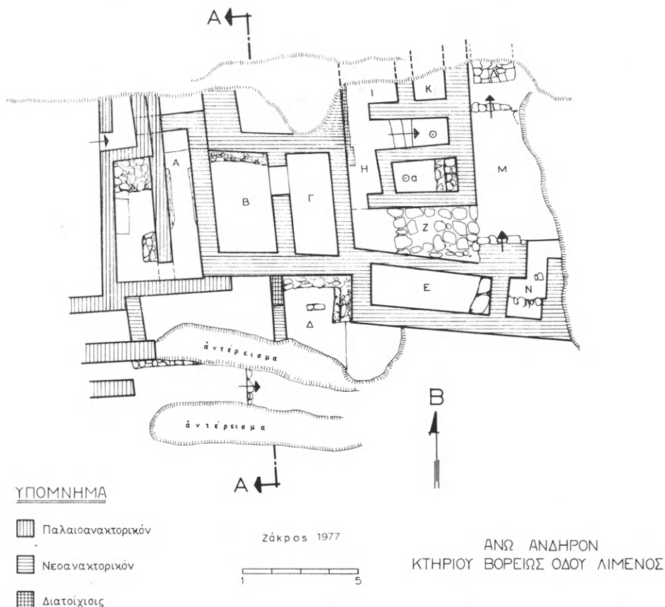
Εἰκ. 133. Ζάκρος. Κάτοψις τοῦ Κτηρίου βορείως τῆς Ὁδοῦ λιμένος. Μεσαῖον ἀνδῆρον.
