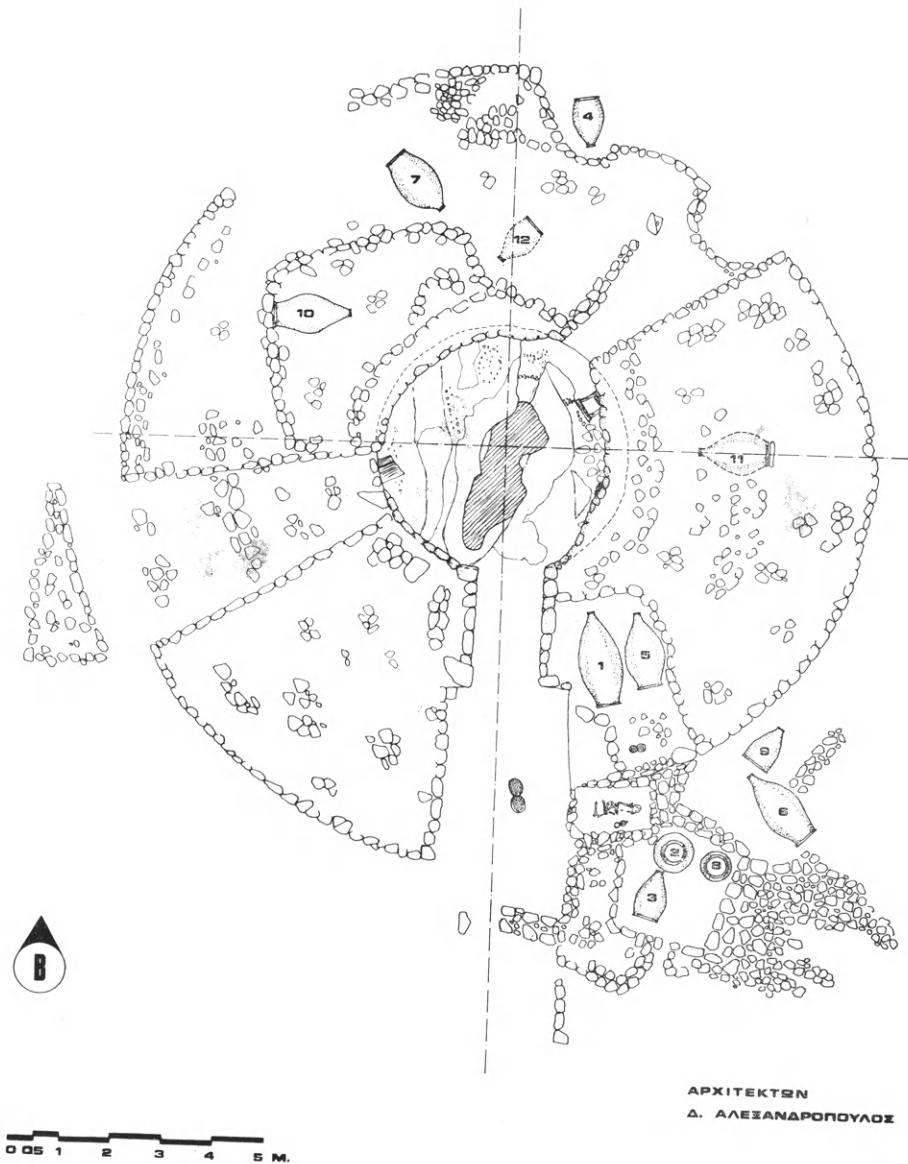
Είχ. 83. Βοῦδοκοιλιά. Κάτοψις τοῦ τύμβου (σκαρίφημα).
