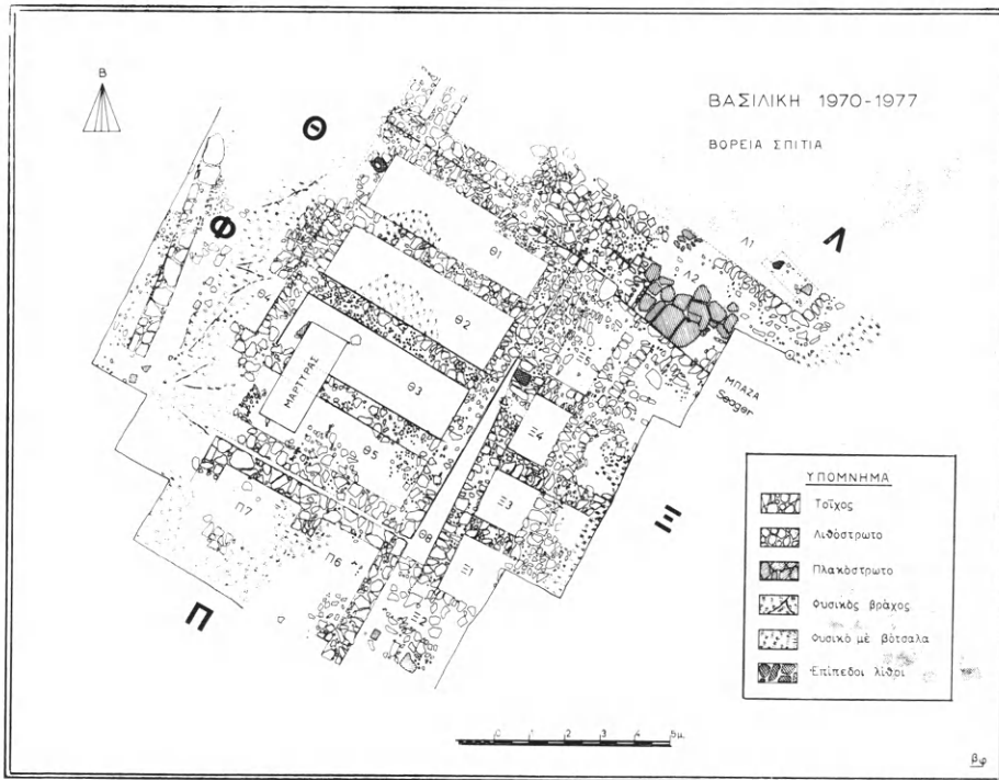
Εἰκ. 137. Σχέδιον τῆς ἀνασκαφῆς εἰς τὴν περιοχὴν τῶν ΠΜ ΙΑ Βορείων Οἰκιῶν.
