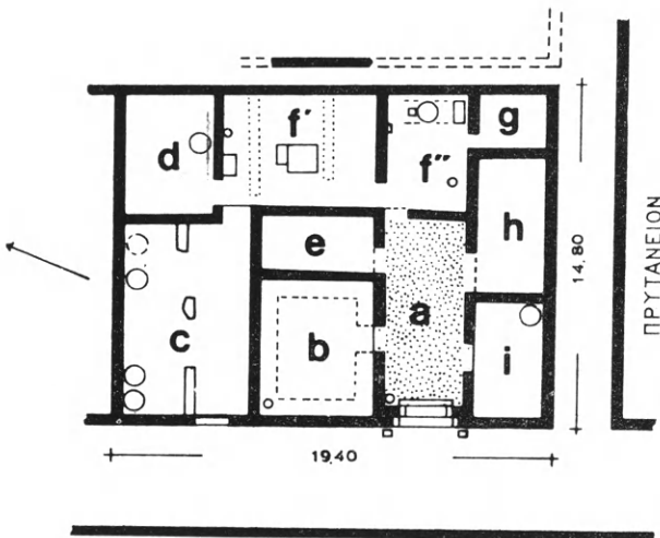
Εἰκ. 43. Κασσώπη. Κάτοψη τοῦ σπιτιοῦ.
