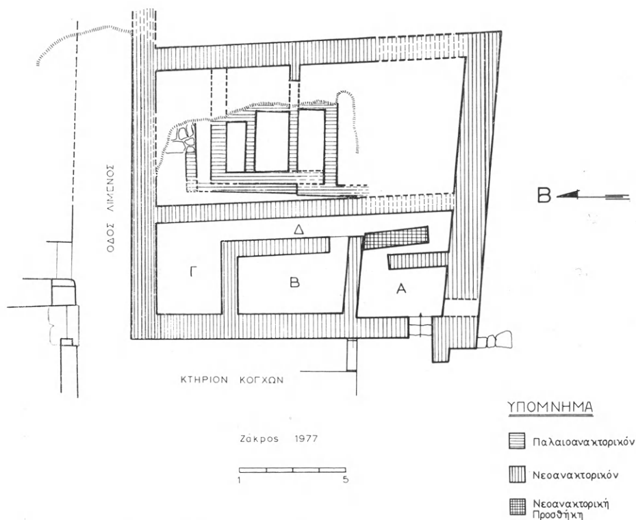
Εἰκ. 126. Ζάκρος. Τὸ Ἀνατολικὸν κτήριον. Κάτοψις.
