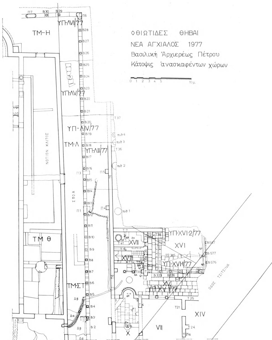
Εἰκ. 29. Κάτοψις τῆς βασιλικῆς ἀρχιερέως Πέτρου.
