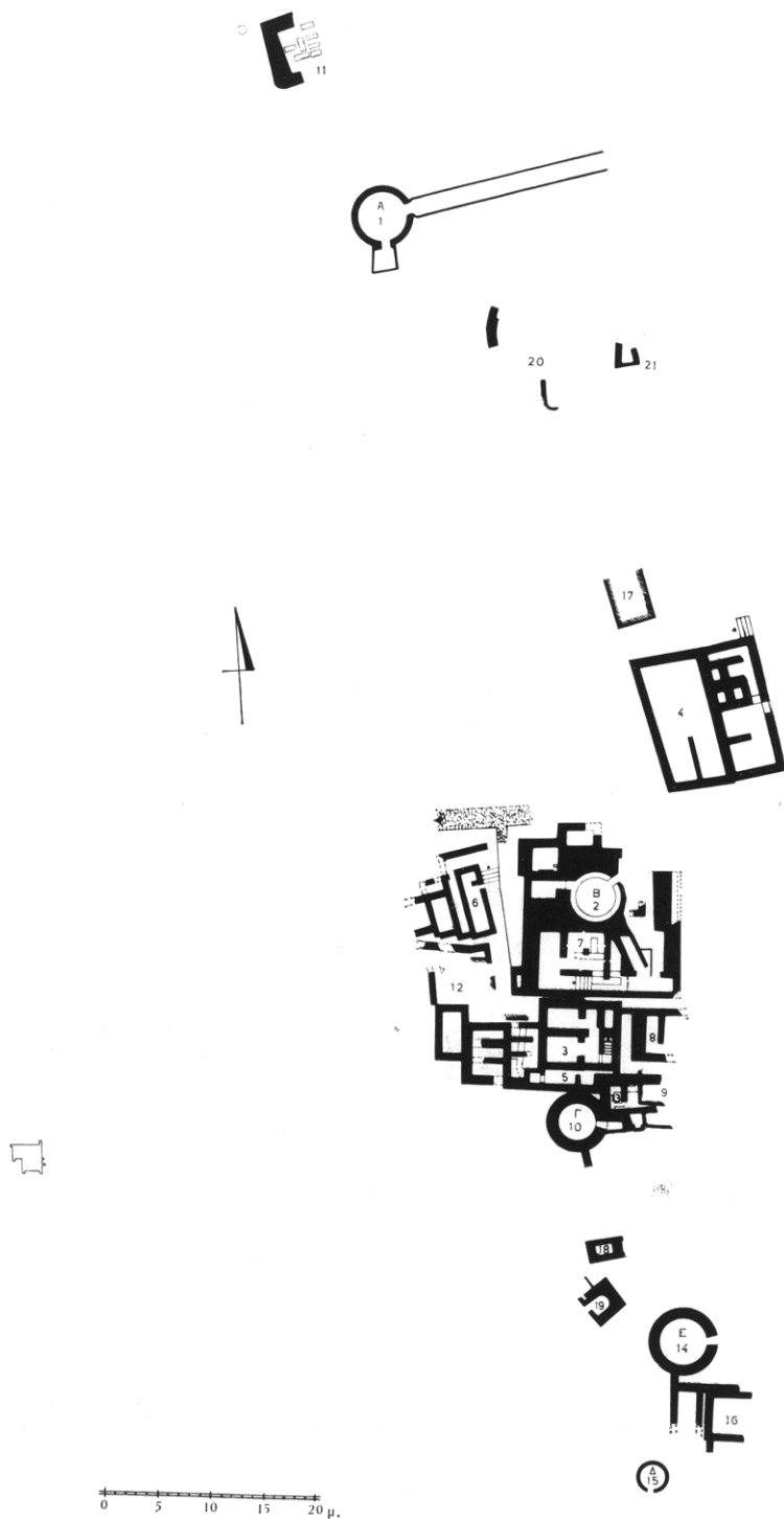
Εἰκ. 111. Ἀρχάνες. Κάτοψις τοῦ μινωικοῦ νεκροταφείου εἰς Φουρνί.
