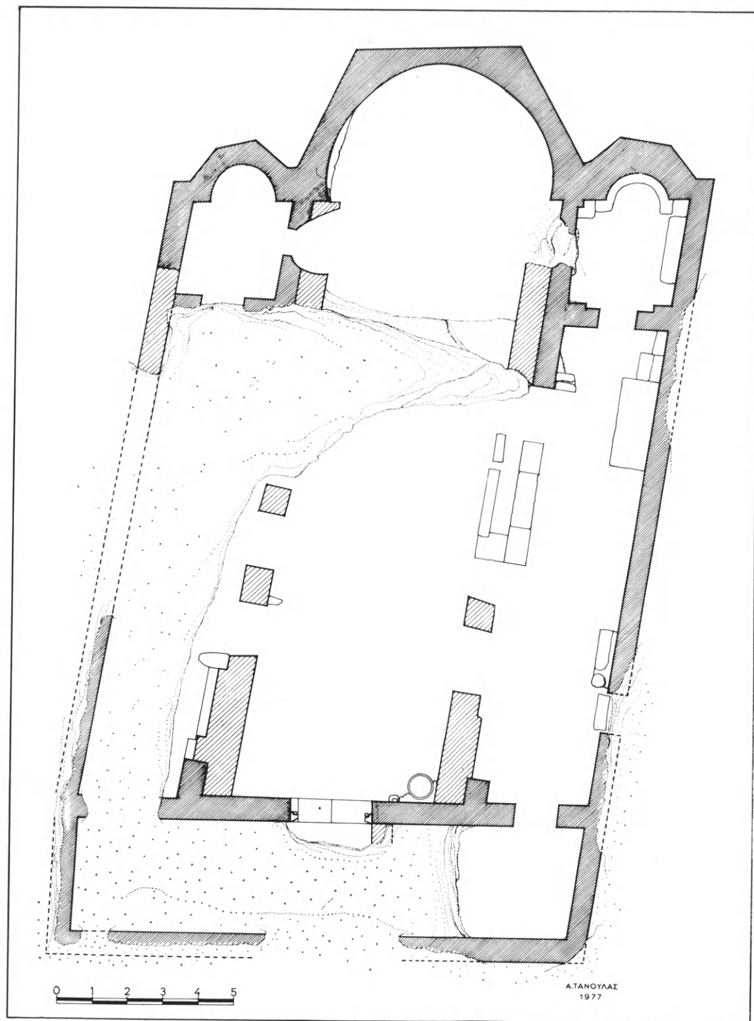
Εικ. 71. Μόνη. Κάτοψις τῆς βασιλικῆς εἰς τὸ ἀκρωτήριο Τηγάνι.
