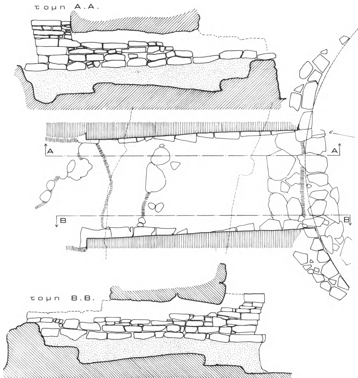
Είχ. 79. Περιστεριά. Κάτοψις και τομή τοῦ ἐρευνηθέντος στομίου τοῦ τάφου.
