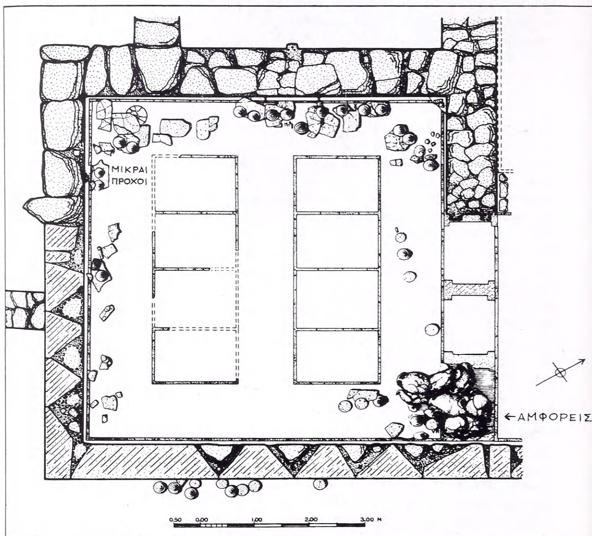
96. Κάτοψις τῆς αἰθούσης συμποσίων μὲ τὴν σκευὴν καὶ τὰ λείψανα τοῦ διαζώματος τῶν σπειρῶν ἐπὶ τόπον.
