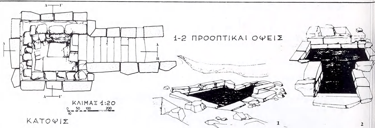
105. Κάτοψις, τομὴ καὶ σκαριφήματα τῆς «τυκτῆς κρήνης».
