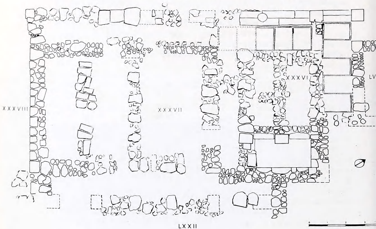
99. Κάτωσις τῶν βασιλικῶν διαμερισμάτων, δεικνύουσα τὰ ἀνευρεθέντα λείψανα.
