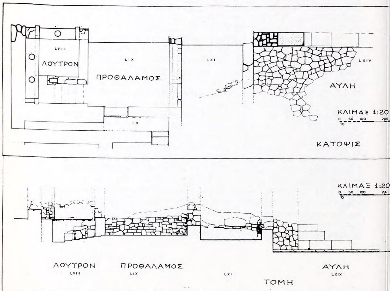
101. Κάτοψις καὶ τομὴ τοῦ λουτροῦ καὶ τῶν συνεχομένων διαμερισμάτων.
