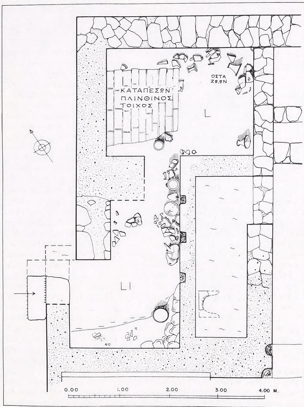
109. Κάτωφλι των βοηθητικών δωματίων τοῦ μαγειρείου, ἔνθα ἐσημειώθη ἡ θέσις τῶν ἀνευρεθέντων σκευῶν καὶ ὁ καταρρεύσας ἐξ ὀπτοπλίνθων τοίχος.
