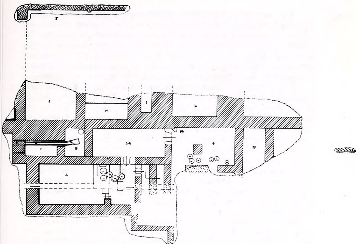
31. Κάτοψις τῆς μινωικῆς ἀγροικίας παρὰ τὴν Ἐπάνω Ζάκρον.
