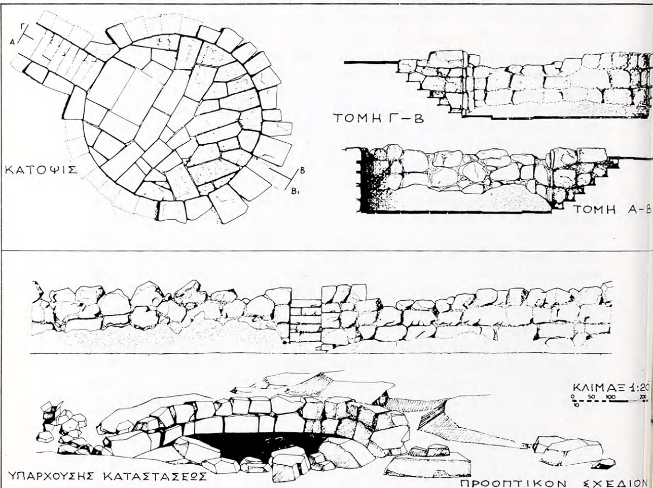
103. Κάτοψις, τομή, ἀνάπτυγμα καὶ σκαρίφημα τῆς κυκλικῆς δεξαμενῆς τῆς μεγάλης τετραγωνικῆς αἰθούσης.
