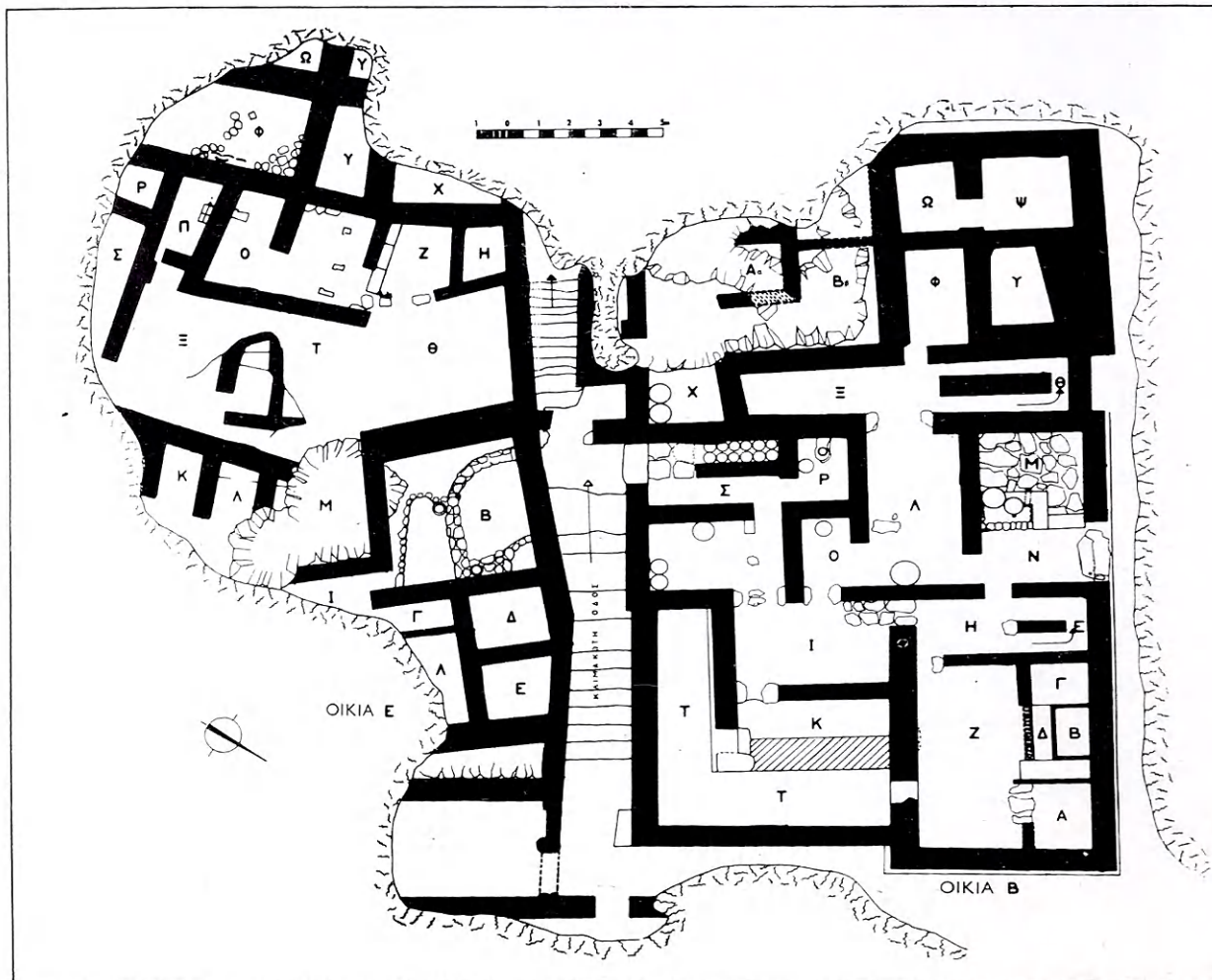
26. Κάτωψις τῶν οἰκιῶν Β καὶ Ε ἐπὶ τῆς κλιτῶς τοῦ νοτιοδυτικοῦ λόφου.
