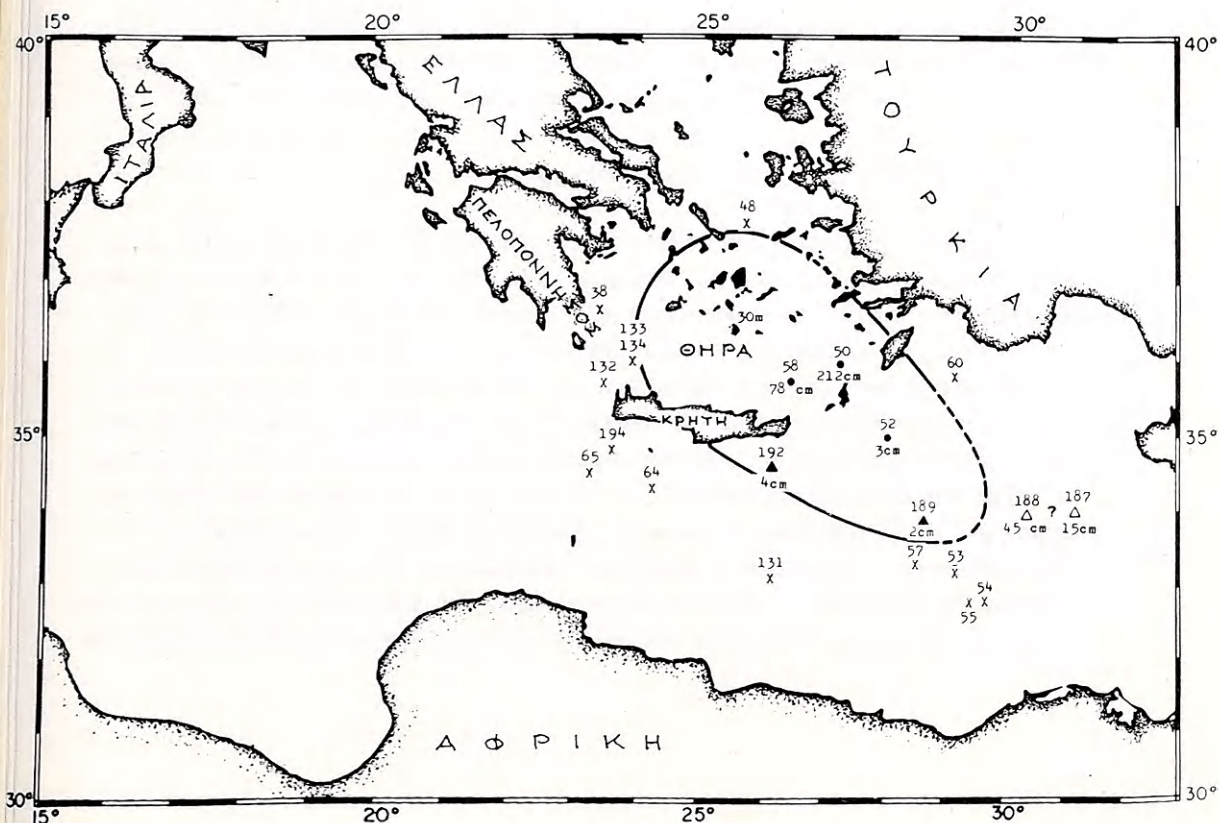
135. Διασπορὰ τῆς ἡφαιστειακῆς τέφρας κατὰ τὴν ἔκρηξιν τοῦ ἡφαιστείου τῆς Θήρας περὶ τὸ 1450 π.Χ.
