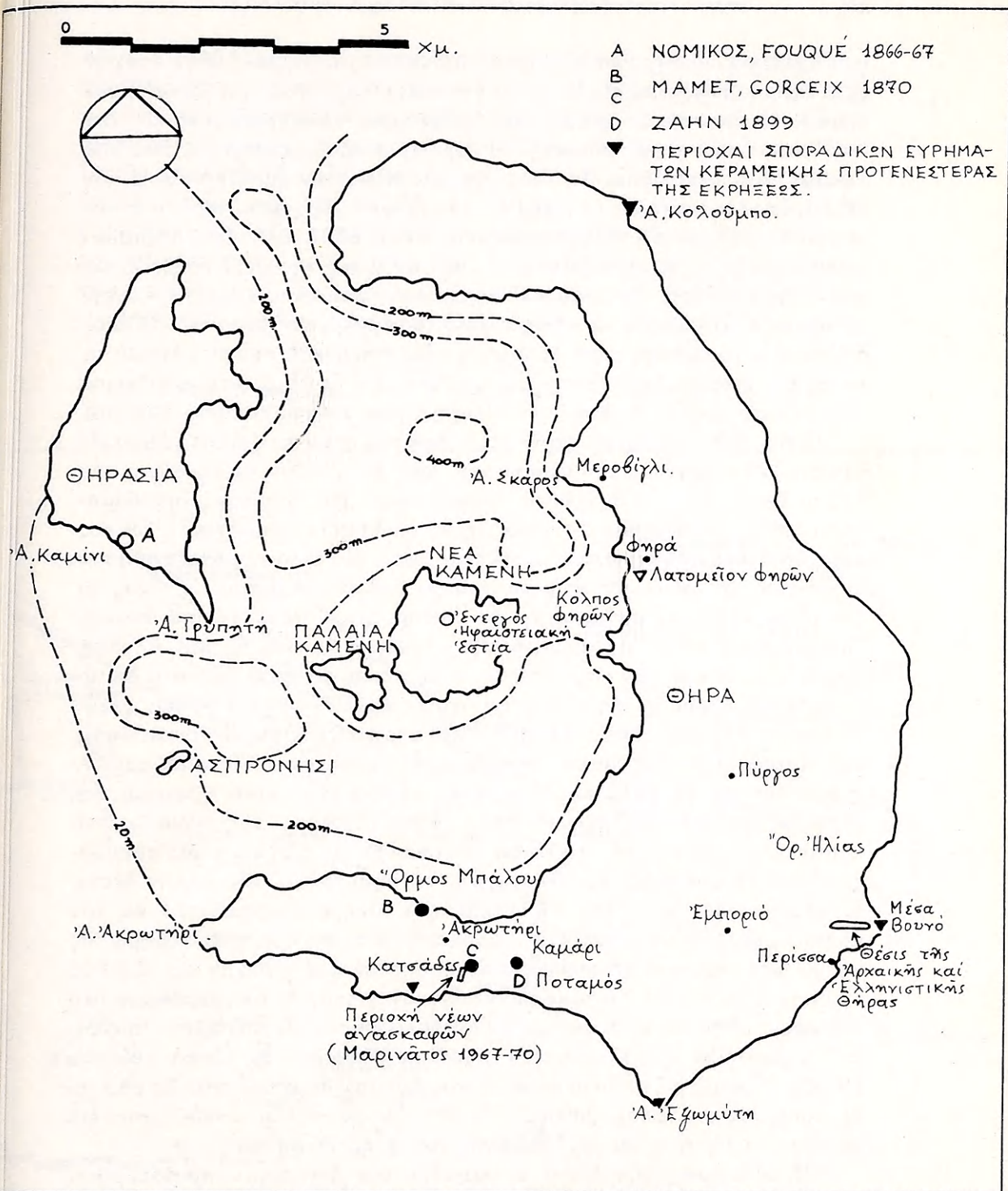
130. Θήρα, Θηρασία καὶ Καμένη, με ἔνδειξιν τῶν ἀνασκαφεισῶν θέσεων (ἡ Παλαιὰ Καμένη ἀνεδύθη ἐκ τῆς θαλάσσης μεταξὺ τῶν ἐτῶν 196 καὶ 157 π.Χ.: ἡ Νέα Καμένη μεταξὺ τῶν ἐτῶν 1701 καὶ 1711 μ.Χ.).
