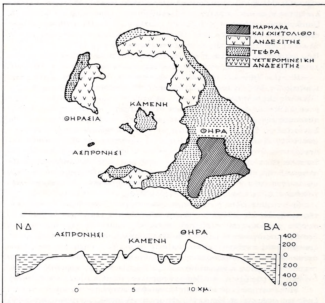
129. Γεωλογικὸς χάρτης τῆς Θήρας.
