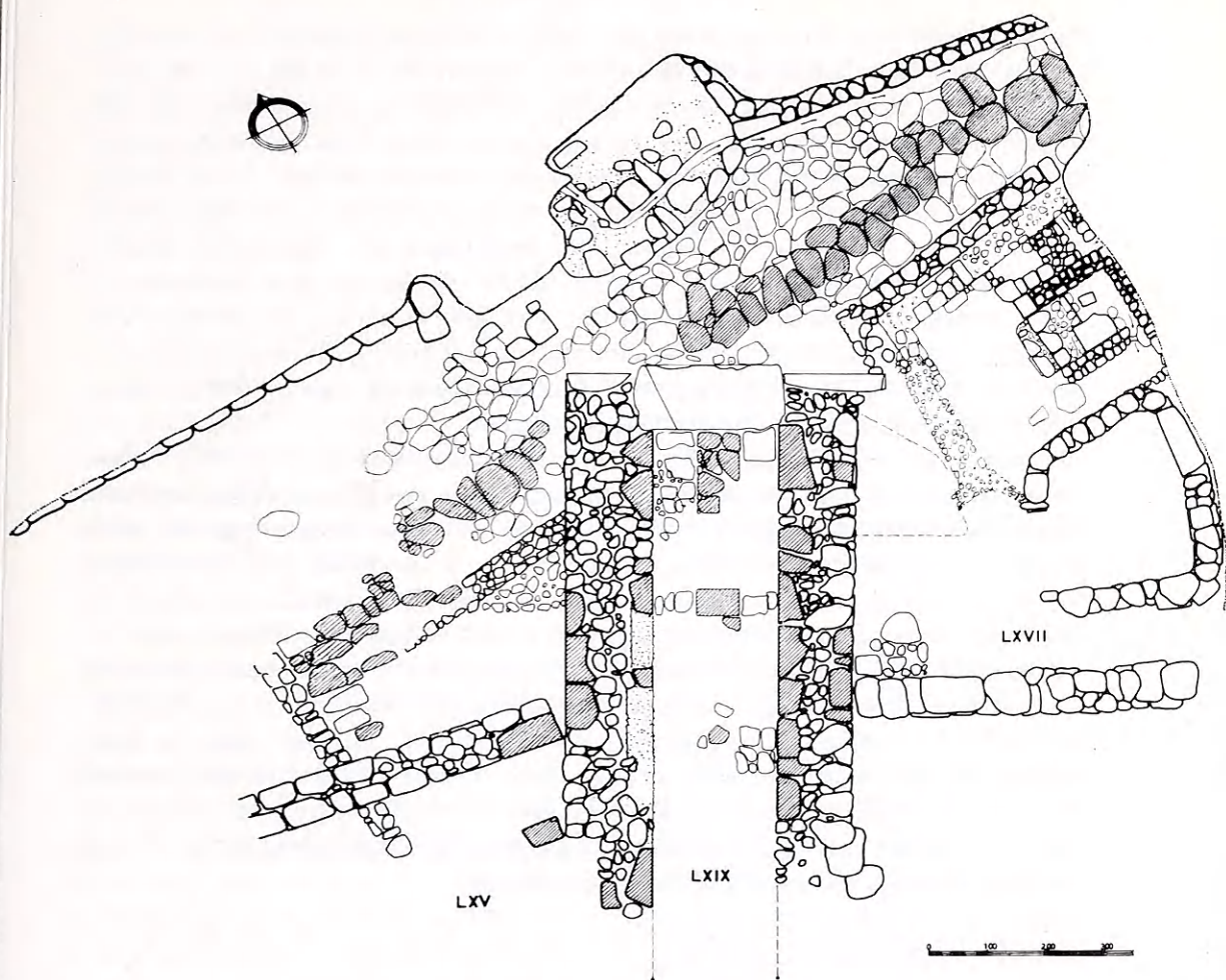
38. Κάτωρις τῆς βορειοανατολικῆς πύλης καὶ τοῦ τέρματος τῆς Ὁδοῦ λιμένος. LXV Βαθμιδωτὰ ἄνθηρα. LXVII Χῶροι κοινόχρηστοι. LXIX ΒΑ. εἴσοδος καὶ δίοδος.
