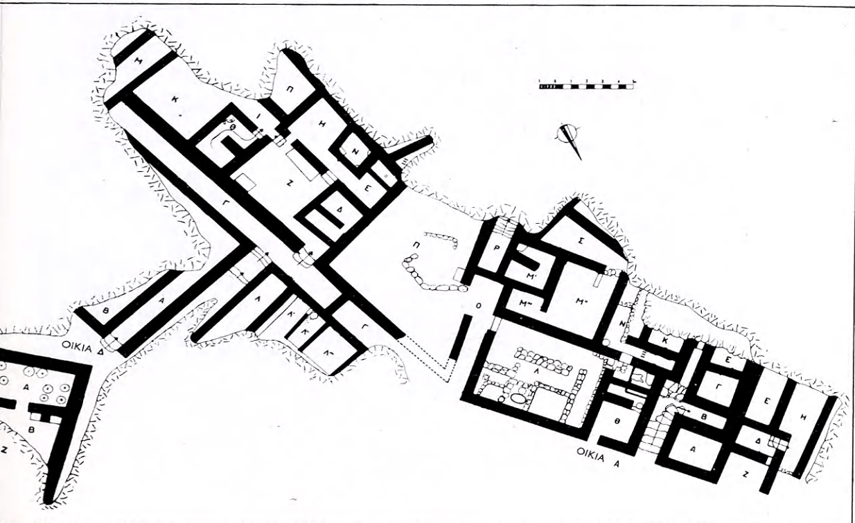
27. Κάτωψις τῶν οἰκιῶν Α, Γ, Δ καὶ Ζ ἐπὶ τῆς κλιτύος τοῦ νοτιοδυτικοῦ λόφου.
