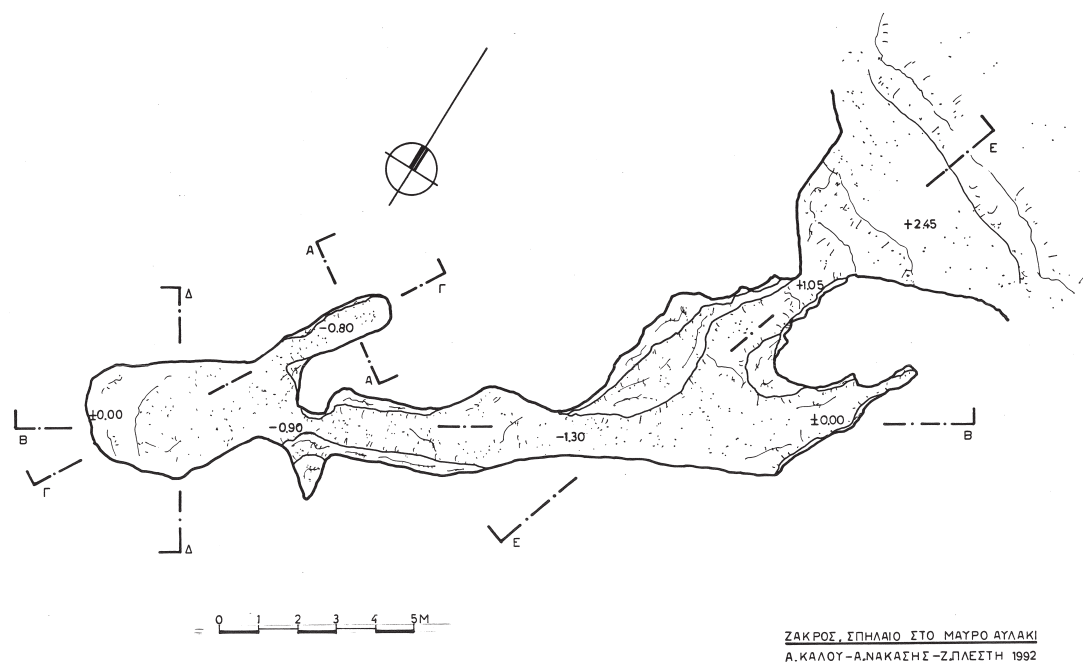
α. Τò σπήλαιο στο Μαύρο Αύλακι. Κάτοψη.
