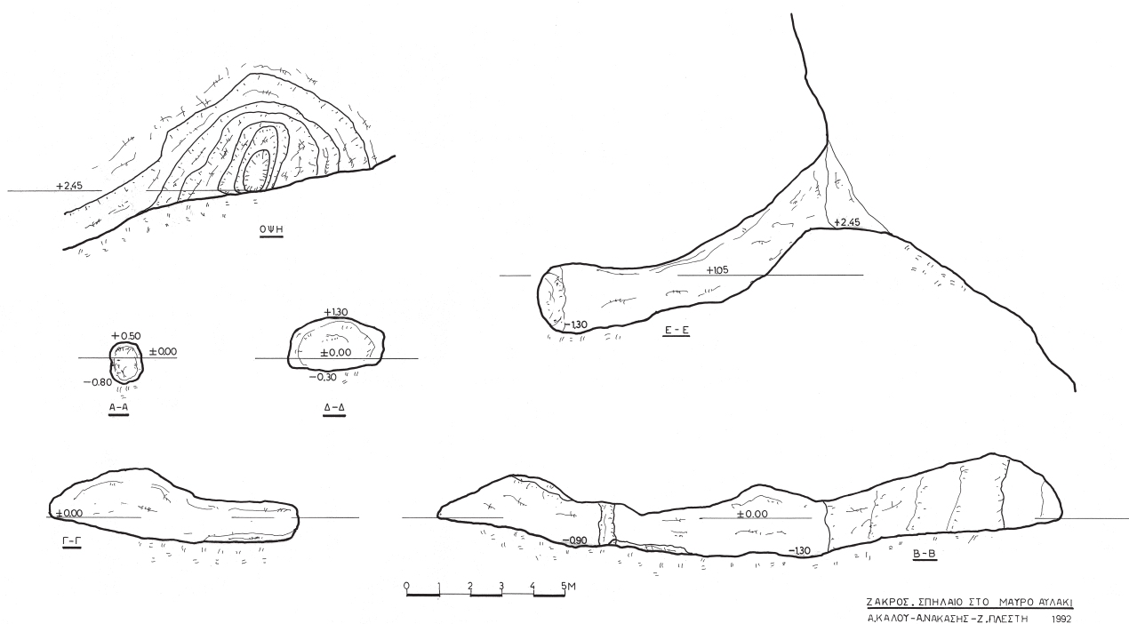
β. Τò σπήλαιο στο Μαύρο Αύλακι. Όψη της εισόδου και σχεδιαστικές, ἐγκάρσιες καὶ κατὰ μῆκος, τομές.
