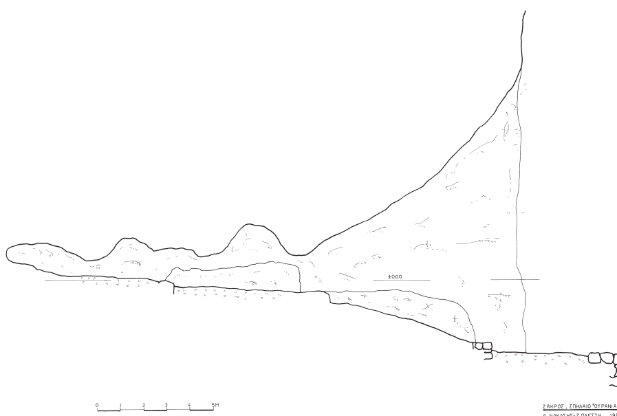
β. Ἐγκάρσια τομὴ τοῦ σπηλαίου.
