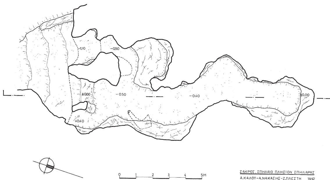
β. Θέση «Σπηλιάρα». Κάτοψη τοῦ Σπηλαίου Α.
