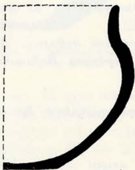
Εἰκ. 22. Κάθετος τομή τοῦ ὑπ' ἀριθ. 86 ὑψιλαίμου κυπέλλου (1:2).
