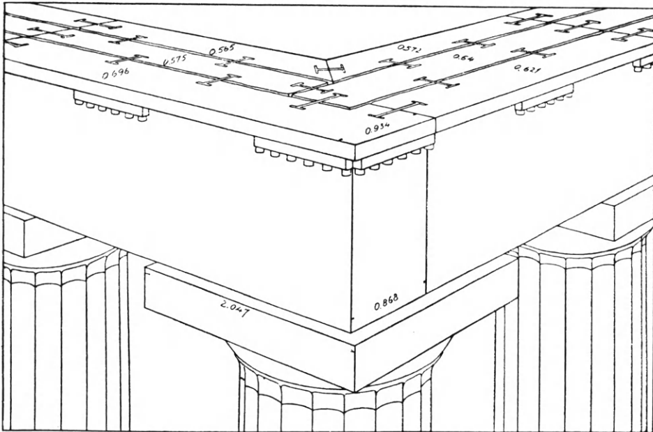
Εἰκ. 195. Συνάντησις τῶν γωνιαίων ἐπιστυλίων τοῦ Παρθενῶνος (Ὁρλάνδος).
