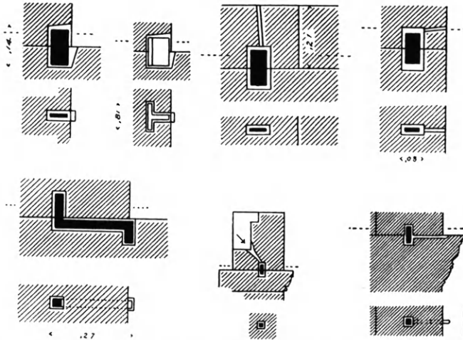
Εἰκ. 143. Συστήματα γομφώσεως καὶ μολυβδοχοΐας (Stevens παρὰ Fowler - Wheeler).
