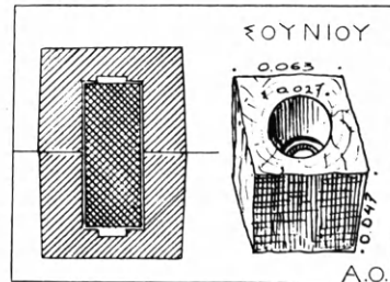
Εἰκ. 148. Ἐμπόλιον καὶ πόλος τοῦ ναοῦ Ποσειδῶνος Σουνίου (Ὁρλάνδος).
