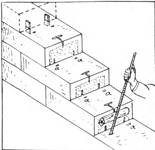
Εἰκ. 155. Γόμφοι καὶ μοχλοβόθρια.
