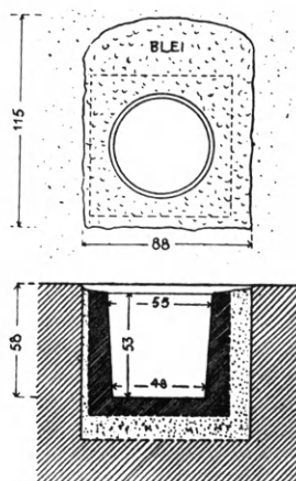
Εἰκ. 160. Χοινικὶς στρογγύλου γόμφου τοῦ Διδυμείου τῆς Μιλήτου (Knackfuss).
