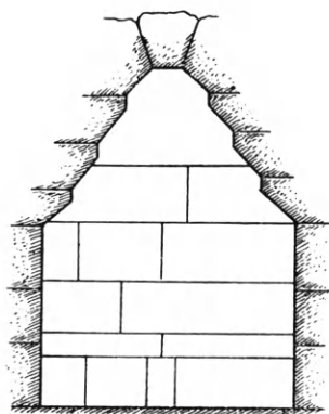
Εἰκ. 279. Τομὴ τάφου τοῦ Orvieto (Durm).
