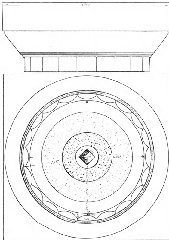
Εἰκ. 133. Κυκλικὴ ἀναθύρωσις τῆς κάτω ἐπιφανείας τοῦ ὑποτραχηλίου κίονος τοῦ Παρθενῶνος (Ὁρλάνδος).
