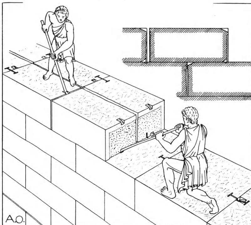
Εἰκ. 70. Χρησις σιδηρῶν μοχλῶν πρὸς μετακίνησιν τῶν λίθων τῇ βοηθείᾳ καὶ λοξῶν ἐγκοπῶν ἀνοιγομένων εἰς τὰς ἄνω καὶ τὰς κάτω κόψεις τῶν λίθων (Ὁρλάνδος).
