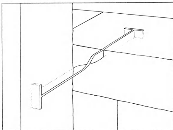
Εἰκ. 138. Λεπτομέρεια τῶν συνδέσμων τῆς εἰκόνης 137.
