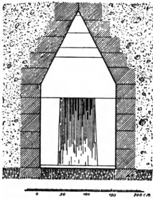
Εἰκ. 289. Ἐγκαρσία τομὴ τοῦ προθαλάμου τοῦ τάφου τοῦ Μάλ - Τεπέ (Filow).
