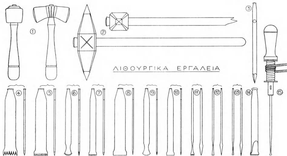
Εἰκ. 56. Σύγχρονα λιθουργικὰ ἐργαλεῖα : 1 μαντρακάς 2 πικούνι 3 βελόνι 4 φαγὰνα 5 ντισιλίδικο 6 λουκλούδικο ντισιλίδικο (διὰ κοιλότητος) 7 ντισιλιδάκι 8 λάμα 9 λαμάκι λουκλούδικο (διὰ γλυφάς) 10 λαμάκι 11 καὶ 12 γλώσσα 13 ποντίλι 14 κοπίδι 15 ἀρίδα.
