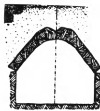
Εἰκ. 333. Τομὴ τάφου τοῦ Τράχωνα τῆς Κύπρου. (Σουηδικὴ Ἀποστολή)
