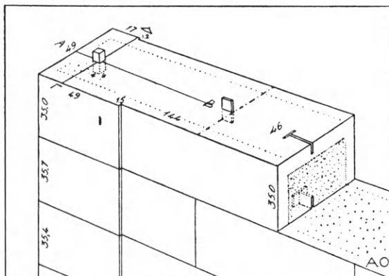
Εἰκ. 102. Καθέτως διασταυρούμεναι χαραγαί (σημεῖαι) ὀρίζουσαι τήν θέσιν τῶν γόμφων τῶν παραστάδων τοῦ ναοῦ τῆς Ἀθηνᾶς Νίκης. (Ὁρλάνδος)
