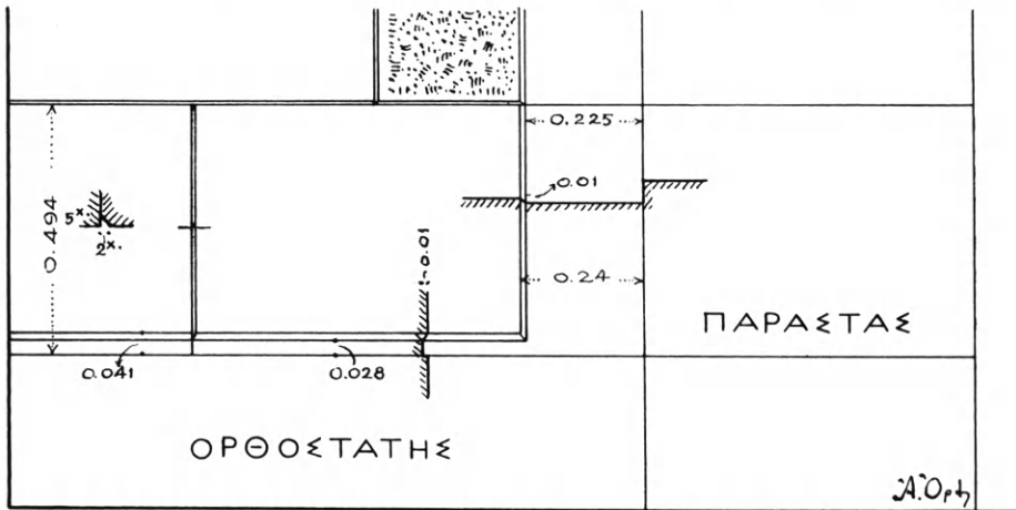
Εἰκ. 88. Τμήμα τοῦ ἡμιλαξευμένου τοίχου τοῦ κυρίου σώματος τῶν Προπυλαίων (ΝΔ. γωνία) δεικνύον τοὺς ὁδηγοὺς (κάτω καὶ πλαγίως) καὶ τοὺς χάσκοντας (χάριν προφυλάξεως τῶν ἀκμῶν) ἄρμους τῶν δόμων ('Ορλάνδος).
