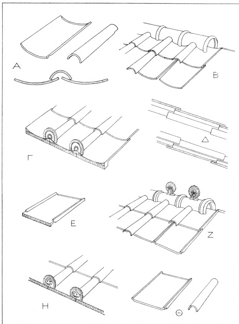
Εἰκ. 56. Πήλιναι λακωνικοῦ τύπου κεραμίδες (Α ἀγέλαιαι, Β κορυφαῖαι, καὶ Γ ἡγεμόνες) καὶ σικελικὴ παραλλαγή αὐτῶν (Ε, Ζ, Η, Θ).
