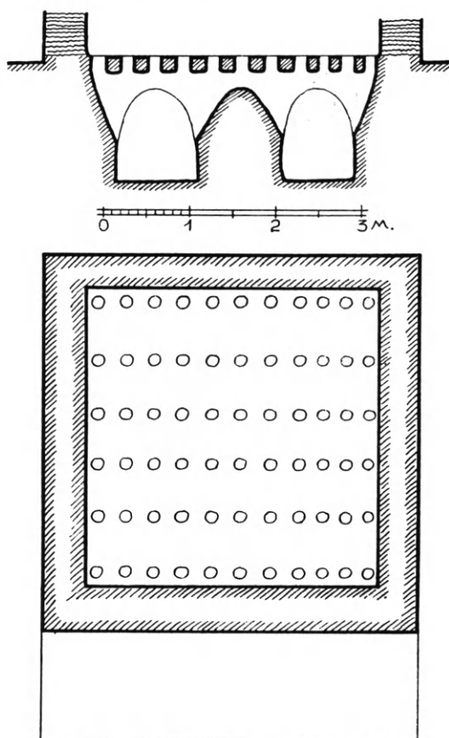
Εἰκ. 43. Κάτοψις καὶ ἐγκαρσία τομὴ τοῦ ἐλληνικοῦ κεραμικοῦ κλιβάνου τῆς Ὀλυμπίας (Schleif).
