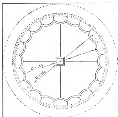
Εἰκ. 99. Σημεῖται δηλοῦσαι τοὺς ἀξονας ἐπὶ τοῦ ὑποτραχηλίου τοῦ ἐν Δελφοῖς δευτέρου ναοῦ τοῦ Ἀπόλλωνος (Courby).
