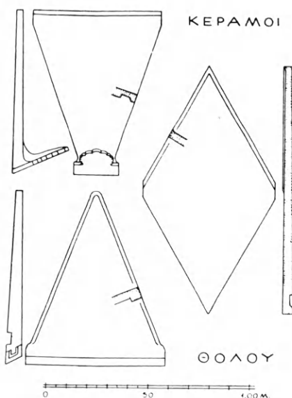
Εἰκ. 62. Τριγωνικαὶ καὶ ρομβόσχημοι κέραμοι ἐκ τῆς Ἀθηναϊκῆς Θόλου (Thompson).
