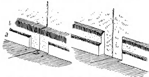
Εἰκ. 237. Πλευρική ἀπόληξις τῶν ὑποτομῶν εἰς προστατευτικὸν ἄπεργον τῶν ἀρμῶν. (Koldewey - Puchstein)
