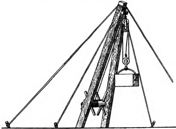
Εἰκ. 45. Ἀναπαράστασις δικώλου μηχανῆς κατὰ Βιτρούβιον (Beck).
