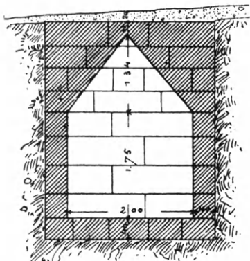
Εἰκ. 280. Ἀρχαῖος τάφος τοῦ Σελινούντος μετὰ τριγωνικὴν ἐκφορικὴν θόλον (Cavallari).
