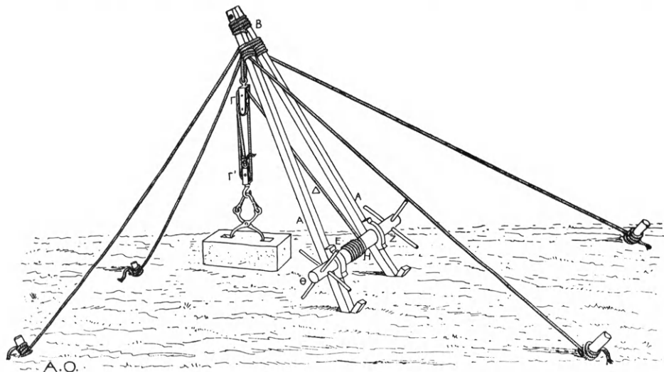
Εἰκ. 44. Ἀναπαράστασις δικώλου (τρισπᾶστου) μηχανῆς κατὰ Βιτρούβιον (Blümner: Ὁρλάνδος).
