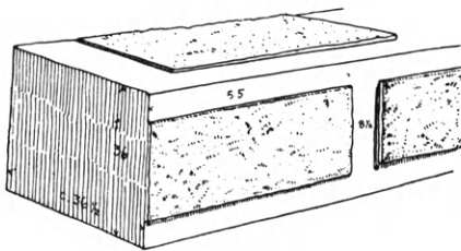
Εἰκ. 89. Λίθος τοῦ ἀρχαιότερου ναοῦ τῆς Ἀφαιῆς μετ' ἀπέργων καὶ περιτενεῶν (Furtwängler).
