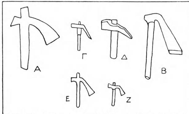
Εἰκ. 19. Σκέπαρνα ἐπὶ ἐπιτυμβίων ἀναγλύφων ρωμαϊκῶν καὶ παλαιοχριστιανικῶν χρόνων τῆς Ν. Γαλλίας (Deonna καὶ Espérandieu). Α. Escuelles, Β. Ἀρελάτου (Arles), Γ. Vaison, Δ. Bagnoles, Ε. Igel, Ζ. Μαγεντίας.
