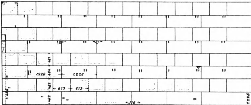
Εἰκ. 231. Σύστημα ἀρμολογίας τοῦ κιμωνεῖου Πύργου τῆς Ἀθηνᾶς Νίκης (Bohn).
