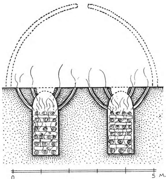
Εἰκ. 42. Κατακόρυφος ἐγκαρσία τομὴ τοῦ κλίβανου τῆς εἰκ. 41 μετ' ἀναπαραστάσεως τοῦ πυρὸς καὶ τοῦ ἄνω μέρους (Ὁρλάνδος).
