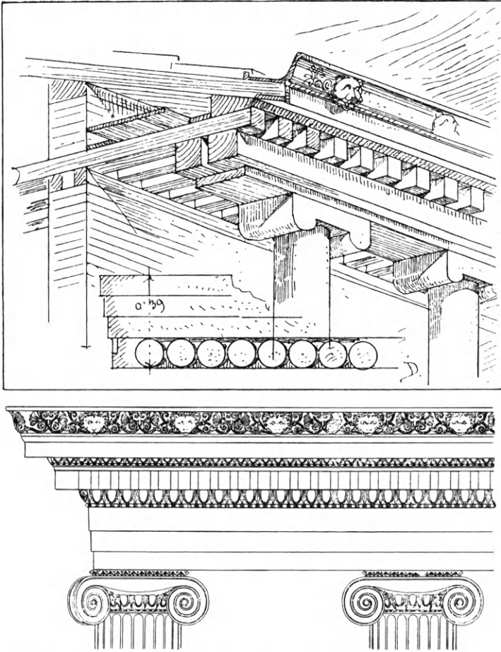
Εἰκ. 8. Κάτω: Λίθινος ἰωνικὸς θριγκός. Ἄνω: Τὸ ξύλινον αὐτοῦ πρότυπον.
