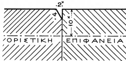
Εἰκ. 90. Ὁριζοντία τομὴ κατακορύφου ἄρμου τῶν Προπυλαίων δεικνύουσα τὴν λοξὴν τομὴν τῶν ἀκμῶν τῶν λίθων μέχρι βάθους 4 χιλιοστῶν καὶ τὴν ὀριστικὴν εἰς βάθος 10 χιλιοστῶν ἐπιφάνειαν εἰς τὴν ὁποίαν θὰ ἔφθανε τελικῶς ἡ λάξευσις τοῦ τοίχου.
