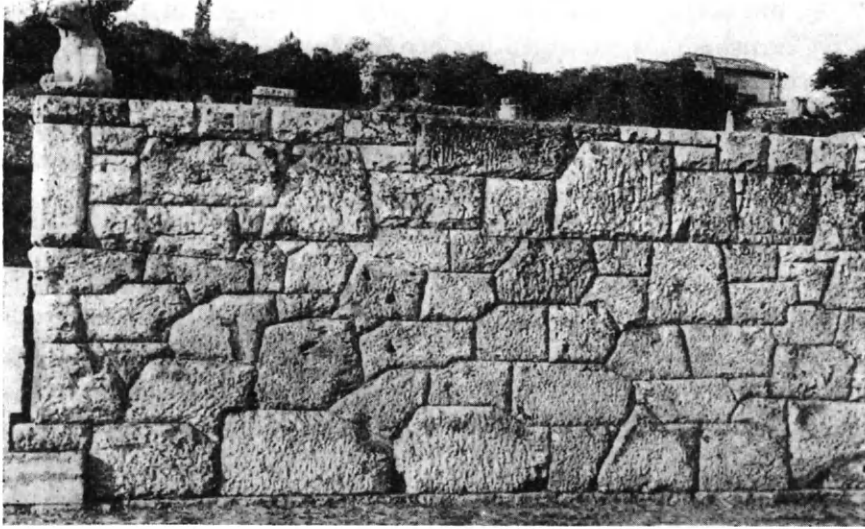
Εἰκ. 173. Ἀνάλημμα τοῦ ἐν τῷ Κεραμεικῷ νεκρικοῦ περιβόλου τοῦ Λυσιμαχίδου (338-317 π.Χ.) με ἐίργασμένην τὴν ἐπιφάνειαν τῶν λίθων καὶ με τονισμένους τοὺς ἄρμους (Wrede).
