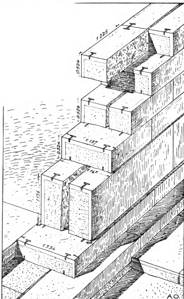
Εἰκ. 183. Σύνδεσις τῶν τοίχων τοῦ σηηκοῦ τοῦ Παρθενῶνος. Κατηγορία 2 εἰκόνας 182 (Ὁρλάνδος).
