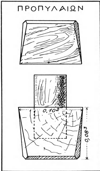
Εἰκ. 146. Ἐμπόλιον καὶ πόλος τῶν Προπυλαίων τῆς Ἀκροπόλεως (Dodwell).
