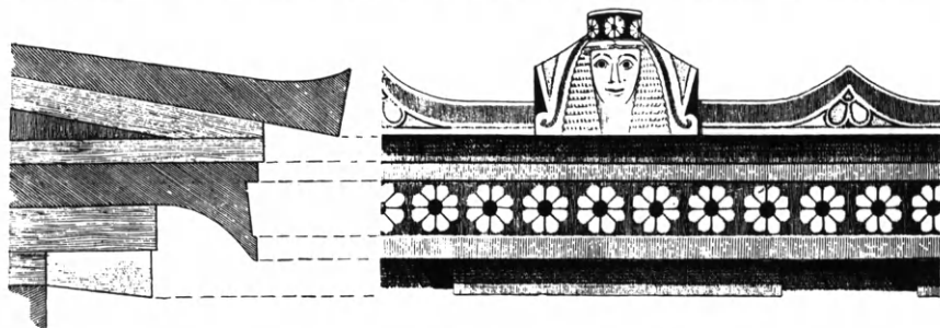
Εἰκ. 46. Κορινθιακὰ πῆλινα γείσα καὶ ἡγεμόνες κέραμοι μετὰ γυναικείων κεφαλῶν δαιδαλικοῦ τύπου ἐκ τοῦ Λαφρναίου τῆς Καλυδῶνος (Ρωμαῖος).
