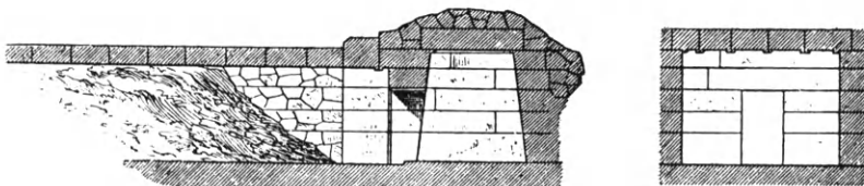
Εἰκ. 243. Κατὰ μῆκος καὶ κατὰ πλάτος τομὴ λυδικοῦ τάφου παρὰ τὰς Σάρδεϊς (Choisy).
