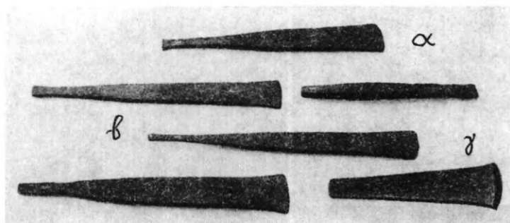
Εἰκ. 62. α, β Λιθουργικὰ ἐργαλεῖα (λείστρια) τῆς ΥΜ 1 περιόδου ἐκ Γουρνιδῶν Κρήτης. Τὸ γ λείστριον (λάμα) τῆς χαλκῆς ἐποχῆς ἐκ Νισύρου (Walters).
