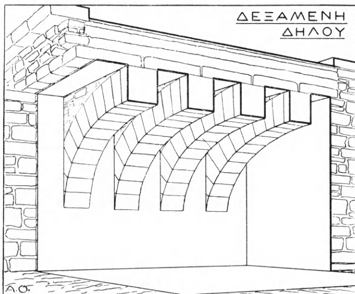
Εἰκ. 366. Προοπτικὴ ἀποψὶς τοῦ ἐσωτερικοῦ τῆς ἐν Δήλῳ δεξαμενῆς τῆς οἰκίας τῆς Τριαίνης (Ὁρλάνδος).
