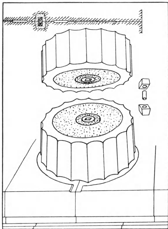
Εἰκ. 149. Σφόνδυλοι μετ' ἐμπολίων τῶν Προπυλαίων (Penrose).
