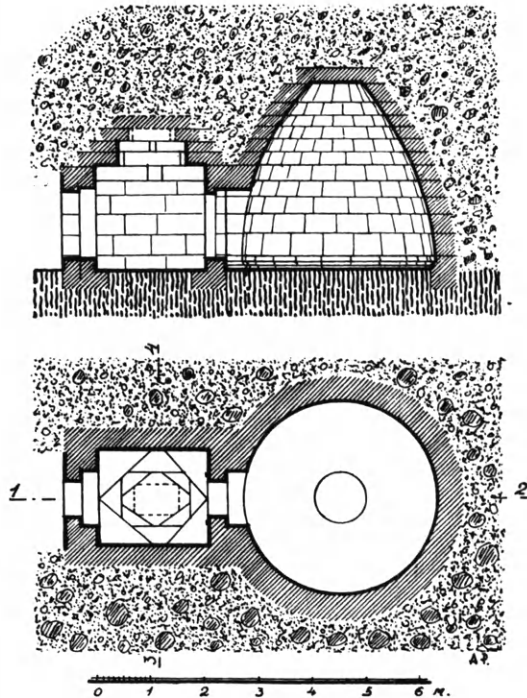
Εἰκ. 290. Κάτοψις καὶ τομὴ τοῦ θολωτοῦ τάφου τοῦ Κούρτ - Καλέ τῆς Θράκης (Filow).
