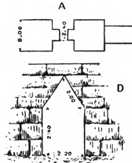
Εἰκ. 316. Πύλη τοῦ τείχους τῆς ἐν Μ. Ἀσίᾳ πόλεως Καύνου (Maiuri).
