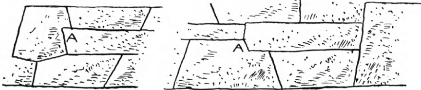
Εἰκ. 175. Ἀκανόνιστον τραπεζιοσχῆμον σύστημα μετ' ὀδοντώσεων Α, Α,
