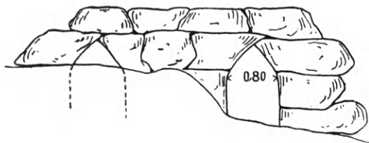
Εἰκ. 317. Πυλίδες μετ' ὀξυκορυφῶν ἐκφορικῶν τόξων τοῦ τείχους τοῦ Μαρμαρᾶ (Holbach).
