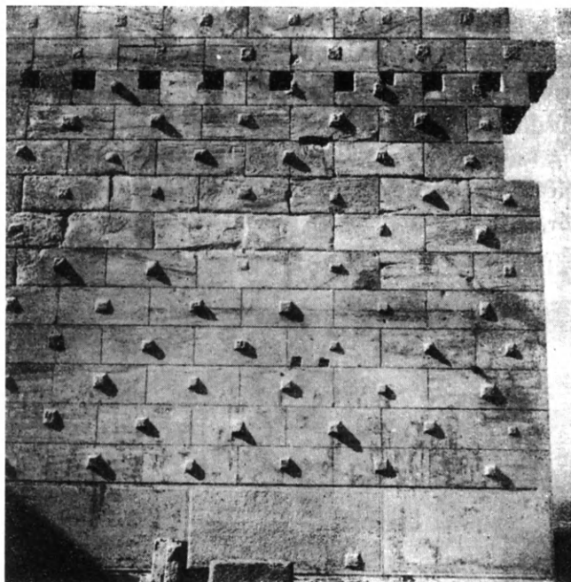
Εικ. 116. Ὁ ἀνατολικὸς τοῖχος τῆς Πινακοθήκης τῶν Προπυλαίων μετ' ἀγκῶνων ἐφ' ἑκάστου λίθου. (Ὁρλάνδος)
