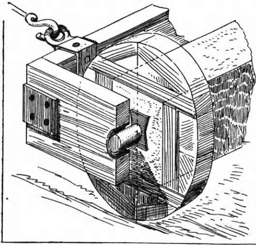
Εἰκ. 36. Λεπτομέρεια τῆς εἰκόνος 35 δεικνύουσα τοὺς κνώδακας (ἀξονίσκους) καὶ τοὺς πελεκίνους (Durm).
