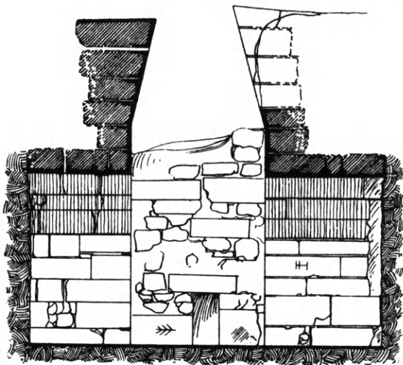
Εἰκ. 256. Τραπεζιόμορφος (;) ἐκφορική κάλυψις τοῦ διαδρόμου τοῦ μεσομινωικοῦ τάφου 'στὰ Σώπατα τῆς Κρήτης (Evans).
