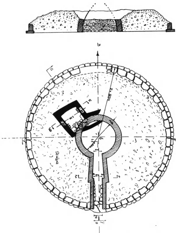
Εἰκ. 403. Κάτοψις καὶ τομὴ τοῦ παρὰ τὰ Φάρσαλα ἀρχαίου θολωτοῦ τάφου (Βερδελῆς).
