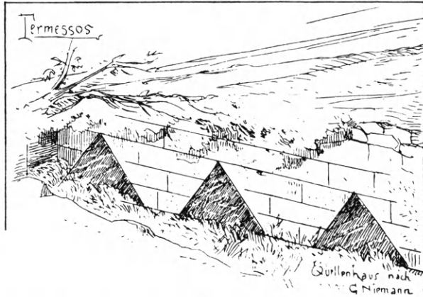
Εἰκ. 327. Κρήνη τῆς ἐν Πισιδίᾳ πόλεως Τελμησοῦ μετὰ τριῶν τριγωνικῶν ἐκφορικῶν τόξων (Durm κατὰ Niemann).
