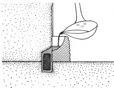
Εἰκ. 14. Μολυβδοχόησις γόμφου (Ὁρλάνδος).
