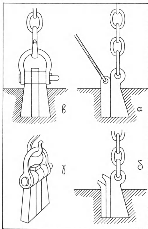
Εἰκ. 128. Σύστημα ἀνυψώσεως τῶν λίθων διὰ λύκου. α, δ ἑλληνικῶν χρόνων β, γ ρωμαϊκῶν.
