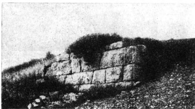
Εικ. 209. Τεῖχος τοῦ ἀρκαδικοῦ Ὀρχομενοῦ τοῦ τραπεζιοσχήμου συστήματος με φυσικὴν τὴν ἐξωτερικὴν ἐπιφάνειαν τῶν λίθων (Lattermann).
