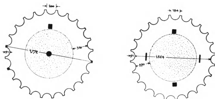
Εἰκ. 158. Γόμφοι μετὰ χοινικίδων εἰς σφονδύλους κίωνων τοῦ Διδυμείου τῆς Μιλήτου (Knackfuss). νείας τοῦ ὑπερκειμένου λίθου. Παραδείγματα τοῦ εἴδους τούτου ἔχομεν
