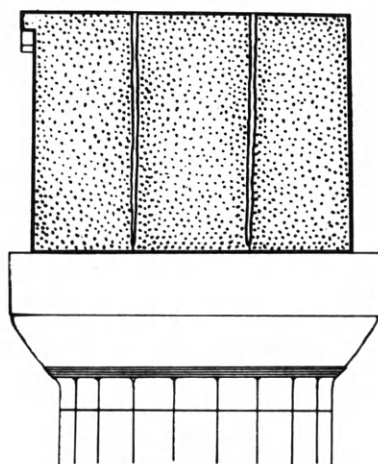
Εἰκ. 85. Τὸ ἐκ τριῶν κατὰ τὸ πάχος τεμαχίων ἐπιστύλιον τοῦ Παρθενῶνος. (Ὁρλάνδος)
