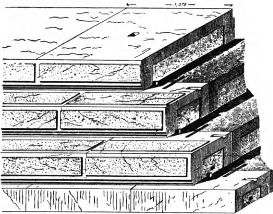
Εἰκ. 218. Ἡ κρητὶς τῆς ἐν Ὀλυμπίᾳ Στοᾶς τῆς Ἡχοῦς. Ἄνω δεξιᾷ (εἰκ. 219) λεπτομέρεια τοῦ ἄκρου τῆς (Dörpfeld).
