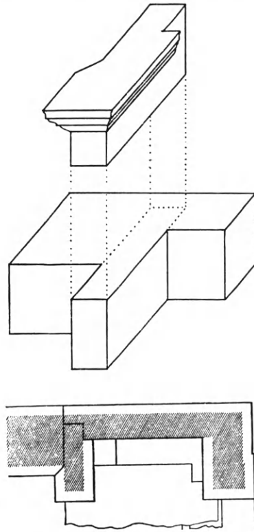
Εἰκ. 200. Μασχαλιαῖα πλίνθος τοῦ Ἑρεχθείου (Stevens).
