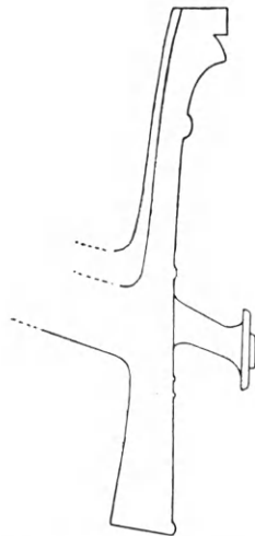
Εἰκ. 47. Πηλίνη σίμα συμφύτης πρὸς ἐπένδυσιν γείσου ἐκ τοῦ ναοῦ τῆς Κερκύρας (Ρωμαῖος)
