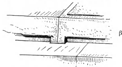
Εἰκ. 103. Προφυλακτικά τῶν ἀκμῶν ἐξογκώματα διακοσμητικῶς λαξευμένα εἰς τήν κρηπίδα τοῦ ἀρχαιότερου Παρθενῶνος (α), και τοῦ ναοῦ τῆς Ποσειδωνίας (β). (Durrm)
