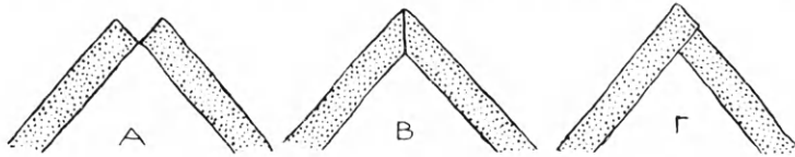
Εἰκ. 329. Συστήματα συνθέσεως τῶν ἀντεριδομένων λίθων στεγάσεως.
