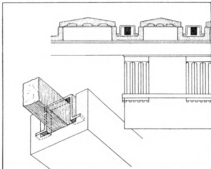
Εἰκ. 12. Δοκοὶ ὀροφῆς τοῦ προνάου τοῦ ναοῦ τῆς Φιγαλείας ἀνηρηγμέναι ἀπὸ σιδηρῶν πυρήνων (Dinsmoor).
