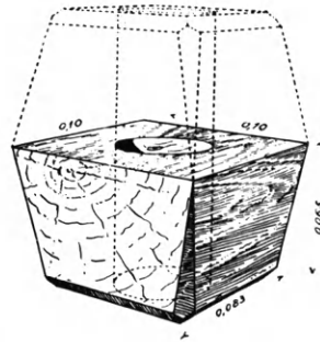
Εἰκ. 147. Ἐμπόλιον ἐκ ξέδρου τοῦ Εὐρεχθείου ἐν τῷ μουσεῖῳ Ἀκροπόλεως (Stevens).
