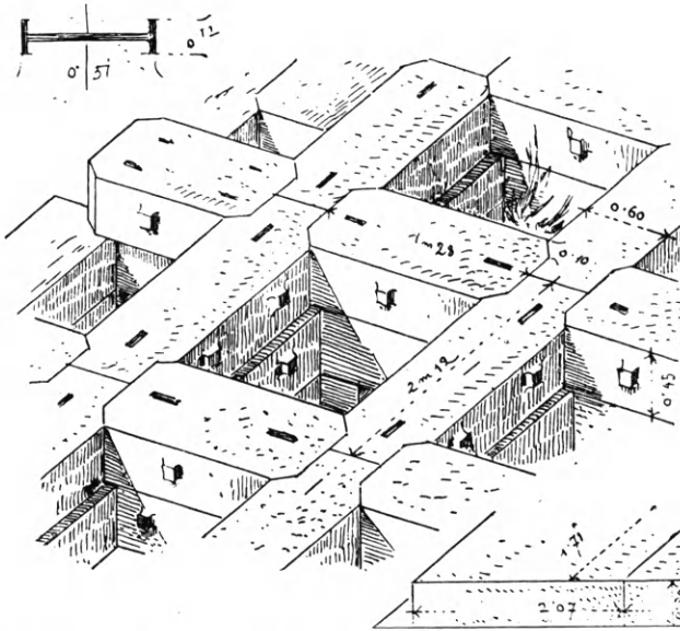
Εἰκ. 191. Κρατευταὶ τοῦ ἐν Δελφοῖς β' ναοῦ τοῦ Ἀπόλλωνος (Durm).
