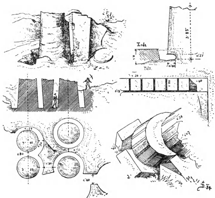
Εἰκ. 30. Λατομῖαι ἐξορύξεως κορμῶν κίωνων τοῦ Σελινούντος.
