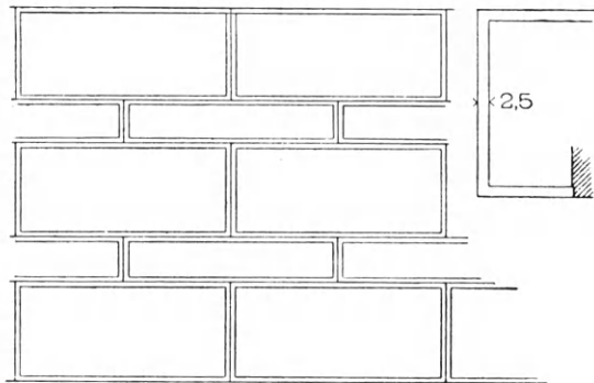
Εἰκ. 238. Τοίχος τοῦ σηκοῦ τοῦ ναοῦ τοῦ Διὸς Σωσιπόλιδος Μαγνησίας τῆς ἐπὶ Μαιάνδρῳ, μὲ τοὺς λίθους φέροντας καὶ κατὰ τὰς τέσσαρας πλευρὰς βαθυσμένην ταινίαν (Kohle).
