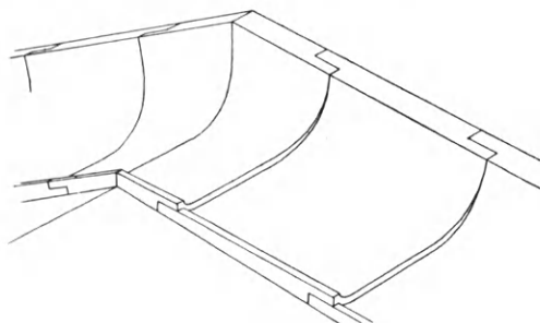
Εἰκ. 58. Κεραμίδες ἐπαιτίδες ἢ παράροι.
