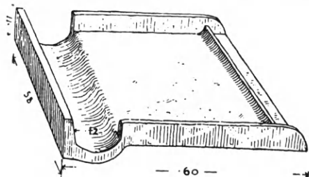
Εἰκ. 59. Κεραμὶς παράρους (;) ἐκ Πριήνης, ἐλληνιστικῶν χρόνων (Wiegand - Schrader).
