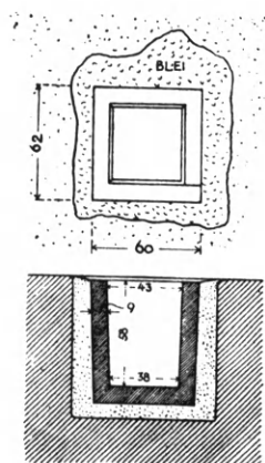
Εἰκ. 159. Τετράγωνος γόμφος μετὰ χοινικίδος τοῦ Διδυμείου τῆς Μιλήτου (Knackfuss).
