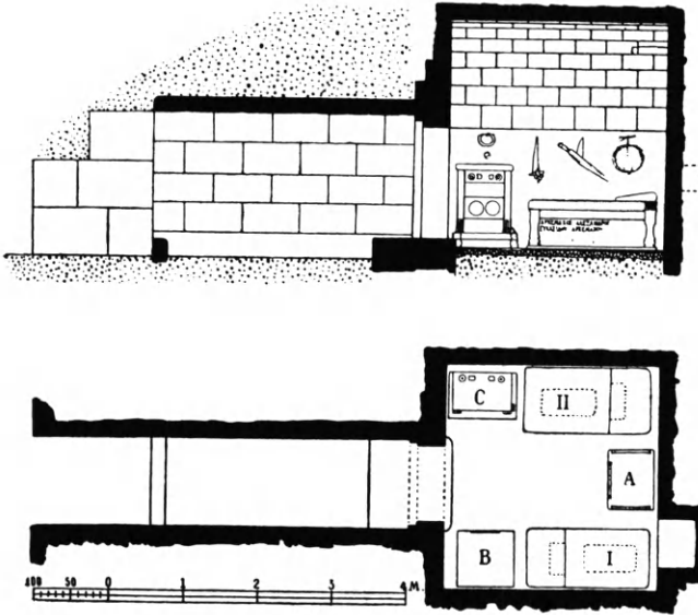
Εἰκ. 371. Κάτοψις καὶ κατὰ μῆκος τομὴ τοῦ θολωτοῦ τάφου τῆς Ἑρετρίας (Vollmöller).
