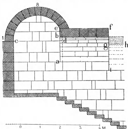
Εἰκ. 368 Τομή τῆς διὰ βαθμιδωτῶν κυλινδρικών θόλων κεκαλυμμένης κλίμακος τοῦ Γυμνασίου τοῦ Περγάμου (Schazmann).
