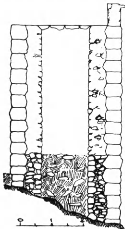
Εἰκ. 164. Τεῖχος τῆς Ἀρχαδικῆς Γόρ- τυνος με ἐσωτερικὴν ἐπέκτασιν διὰ ξη- ρολιθιάς (Martin).
