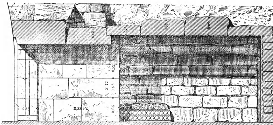
Εἰκ. 242. Κατὰ μῆκος τομὴ τοῦ παραπλεύρου θαλάμου τοῦ ἐν Ὁρχομενῷ τῆς Βοιωτίας θησαυροῦ τοῦ Μινύου.
