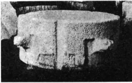
Εἰκ. 115. Ἡμιτελεῖς σφόνδυλοι κιόνων τοῦ Παρθενῶνος μετ' ἀγκῶνων κατὰ τὴν περιφέρειαν.
