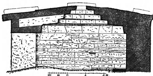
Εἰκ. 312. Ὁρθογώνιον οἶκημα ἐπὶ τῆς κορυφῆς τῆς ἐν Εὐβοίᾳ Ὀχης, καλυπτόμενον διὰ «σκαφοειδοῦς» ἐκφορικῆς θόλου. Τομὴ κατὰ πλάτος (Wiegand).
