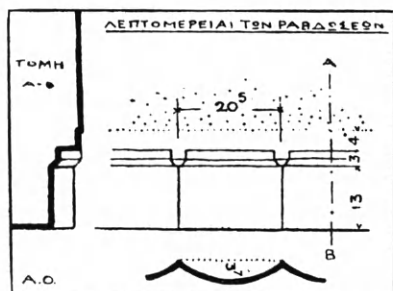
Εἰκ. 93. Ναοῦ Διὸς Στρατίου λεπτομέρειαι τῶν ραβδώσεων.
