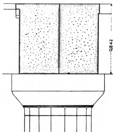
Εἰκ. 84. Τὸ ἐκ δύο κατὰ τὸ πάχος τεμαχίων ἐπιστύλιον τοῦ ἐν Σουνίῳ ναοῦ τοῦ Ποσειδῶνος. (Ὁρλάνδος)
