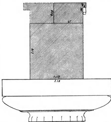
Εἰκ. 86. Τὸ ἐξ ἐνὸς κατὰ τὸ πάχος τεμαχίου ἐπιστύλιον τοῦ ἀρχαίου ναοῦ G τοῦ Σελινοῦντος. (Koldewey)
