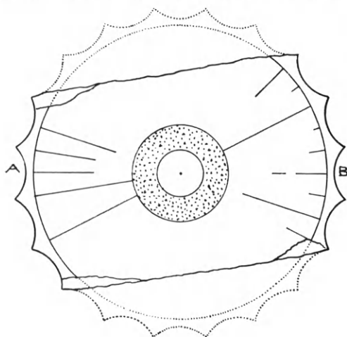
Εἰκ. 97. Σημεῖα δηλωτικὰ τοῦ ἄξονος AB καὶ τῶν ἀκτίνων τῶν ραβδώσεων ἐπὶ σφονδύλων τῆς ΝΔ. πτέρυγος τῶν Προπυλαίων (Ὁρλάνδος).
