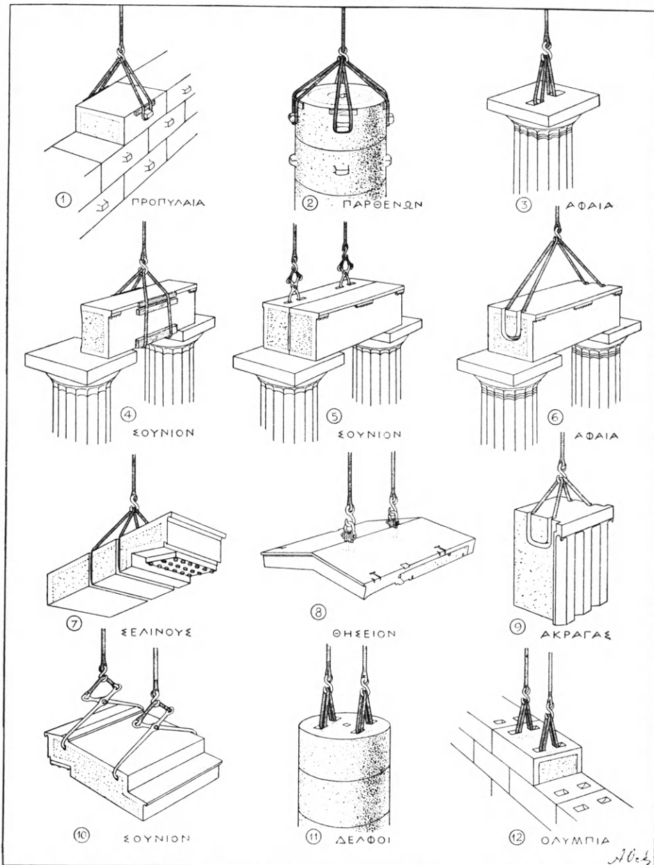
Είχ. 119. Διάφορα συστήματα ανυψώσεως τῶν λίθων.
