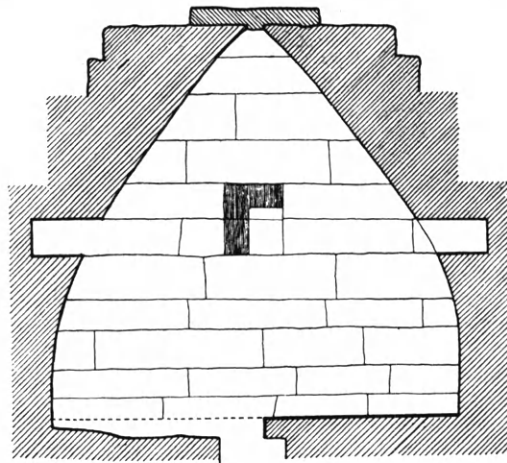
Εἰκ. 270. Κατακόρυφος τομὴ τοῦ ὑπ' ἀριθ. 1 μυκηναϊκοῦ τάφου τῆς Ras Shamra (Schäffer).
