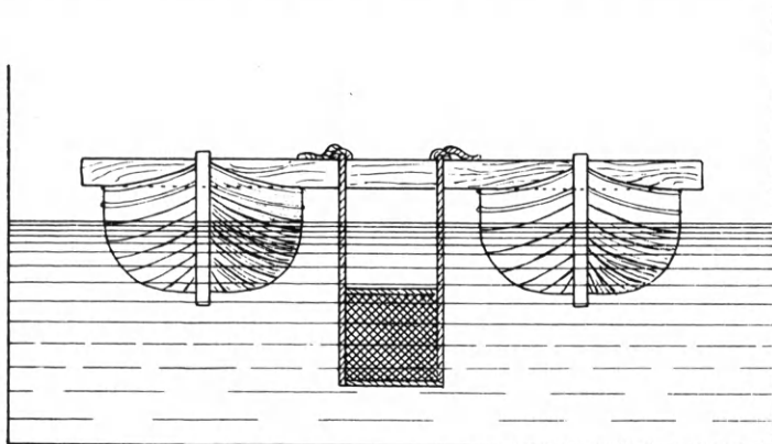
Εἰκ. 39. Μεταφορὰ λίθων δι' ἀμφιπρῦμων φορηγίδων.
