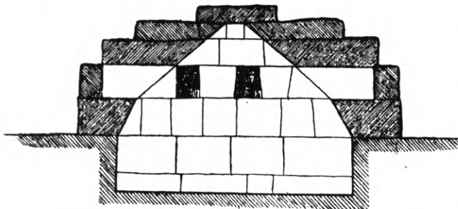
Εἰκ. 267. Τομὴ τῆς σκαφοειδοῦς μυκηναϊκῆς θόλου τοῦ ὑπ' ἀριθ. IV τάφου τῆς Ras Shamra (Schäffer).
