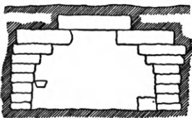
Εἰκ. 259. Τομὴ προμυκηναϊκοῦ τάφου τῆς Σύρου καλυπτομένου διὰ βαθμιδωτῶν ἐκφορικῶν πλακῶν (Bosanquet)
