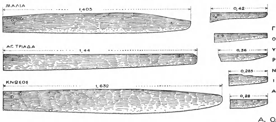
Εἰκ. 20. Πρίονες χαλκοῖ τῆς μινωικῆς ἐποχῆς (ΥΜ Ι περιόδου ἀριστερὰ καὶ ΜΜ δεξιὰ).
