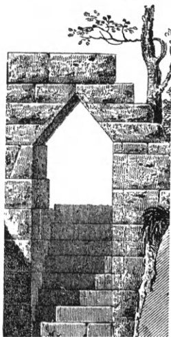
Εἰκ. 302. Πύλη ἐσωτερικοῦ ἀναλήμματος τῆς Μεσσήνης κατὰ Blouet.
