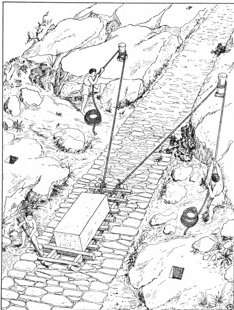
Εἰκ. 37. Ἀναπαράστασις τοῦ τρόπου καταβίβάσεως τῶν ἀρχαίων μαρμάρων ἐκ τοῦ Πεντελικοῦ κατὰ Ἀ. Ὁρλάνδον.
