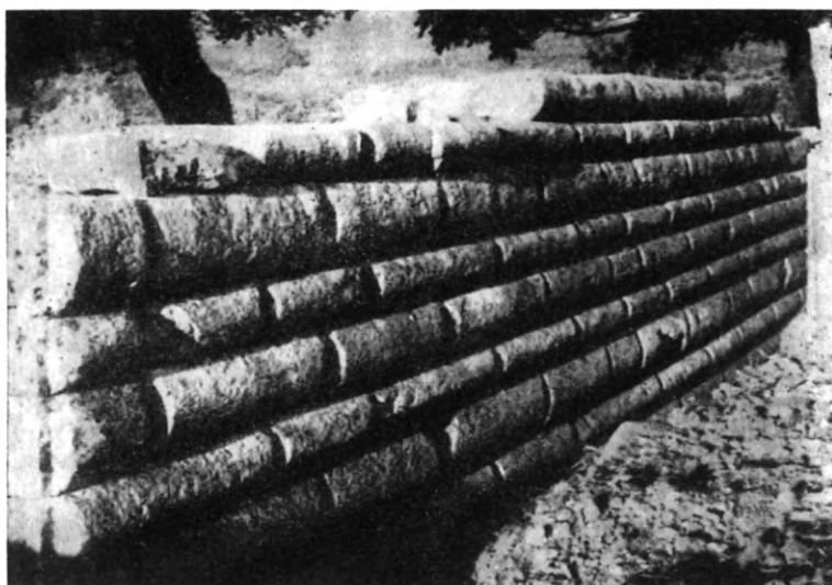
Εἰκ. 227. Τὸ ψευδισόδομον ἀνάλημμα τοῦ θεάτρου τῆς Μεσσήνης μὲ τοὺς λίθους εἰργασμένους ἐν εἵδει προσκεφαλαίου καὶ μὲ λοξὰς τμήσεις ἐκατέρωθεν τῶν κατακορύφων ἀρμῶν (Ὁρλάνδος).
