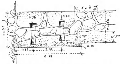
Εἰκ. 134. Πελεκῆνοι τοῦ δυτικοῦ τοίχου ἀνακτόρου τῆς Κνωσοῦ (Durm).
