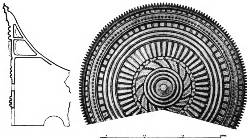
Εἰκ. 55. Τὸ πήλινον μέσον ἀκρωτήριον τοῦ Ἡραίου τῆς Ὀλυμπίας (τομὴ καὶ πρόσοψις).
