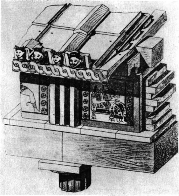
Εἰκ. 45. Ἀναπαράστασις τοῦ θριγκοῦ τοῦ ναοῦ τοῦ Θερμίου Ἀπόλλωνος (Kawerau).
