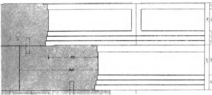
Εἰκ. 216. Ἡ κρητὶς τῆς Νοτίας Στοᾶς τῆς Ὀλυμπίας μετὰ τοὺς λίθους φέροντας περιτένειαν (καθρέπτειν) καὶ ὑποτομὰς (Dörpfeld).
