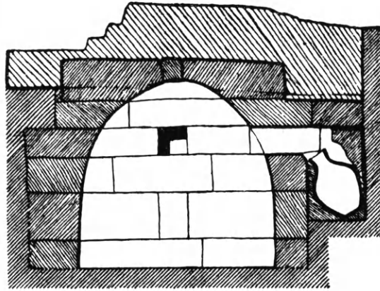
Εἰκ. 272 Κάθετος τομὴ τοῦ ὑπ' ἀριθ. II μυκηναϊκοῦ τάφου τῆς Ras Shamra (Schäffer).
