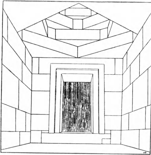
Εἰκ. 248. Προοπτικὴ ὄψις τῆς φατνωματικῆς ὀροφῆς τοῦ προθαλάμου τοῦ τάφου Κούρτ-Καλέ τῆς Θράκης (Filow).
