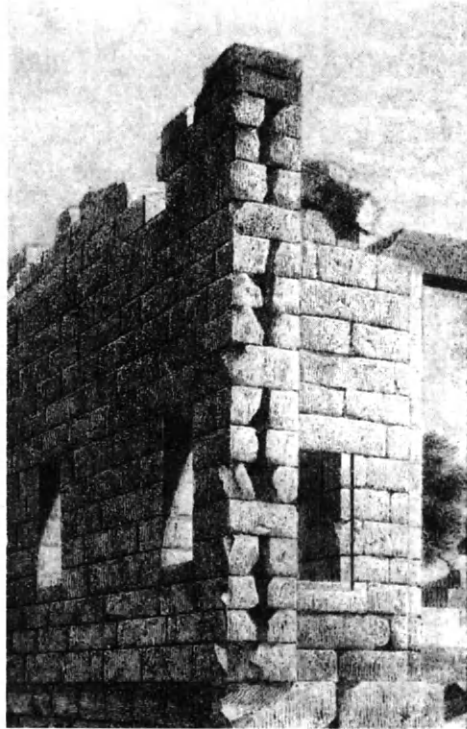
Εἰκ. 186. Ἰσοδόμον σύστημα κατηγορίας 4 τῆς εἰκ. 182, 4 ναοῦ Διὸς Λαβράνδων (1 ου π.Χ. αἰ.) (Le Bas).
