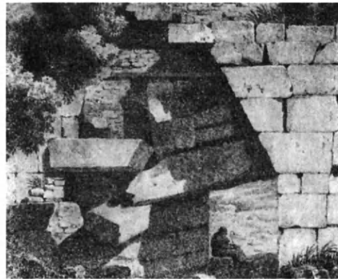
Εἰκ. 305. Ἡμικατεστραμμένη ἀρχαία πύλη τῶν Μεθάνων καλυπτομένη δι' ἐκφορικοῦ τριγωνικοῦ τόξου (Dodwell).
