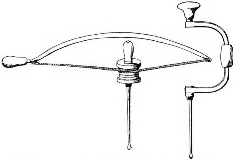
Εἰκ. 66. Σύγχρονα τρύπανα περιστροφικά με ματικάπι· ἀριστερᾷ τὸ δοξάρι.
