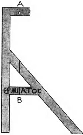
Εἰκ. 75. Γωνία-διαβήτης ἐκ τῶν περιχώρων τῆς Τύρου.
