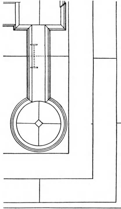
Εἰκ. 101. Καθέτως διασταυρούμεναι χαραγαί (σημεῖαι) ἐπὶ τῆς ἄνω ἐπιφάνειας τῶν βάσεων τοῦ ναοῦ τῆς Ἀθηνᾶς Νίκης ὀρίζουσαι τὸ κέντρον. (Ὁρλάνδος)
