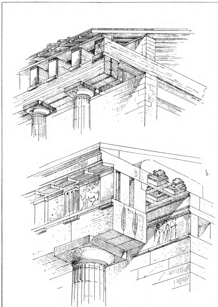
Εικ. 7. Κάτω: λίθινος δωρικός θριγκός. Ἄνω: τὸ ξύλινον αὐτοῦ πρότυπον (Duttm.).
