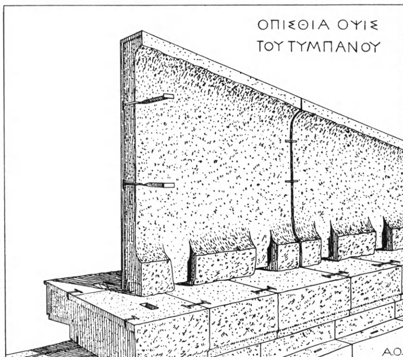
Εἰκ. 137. Στρεπτοὶ σύνδεσμοι σχήματος διπλοῦ ταῦ εἰς τὸν μέσον ὀρθοστάτην τοῦ Δυτικοῦ αἵετώματος τοῦ Παρθενῶνος (Ὁρλάνδος).
