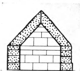
Εἰκ. 332. Ὁ ἀρχαῖος τάφος τοῦ Κιτίου Κύπρου. (Ohnefalsch-Richter)
