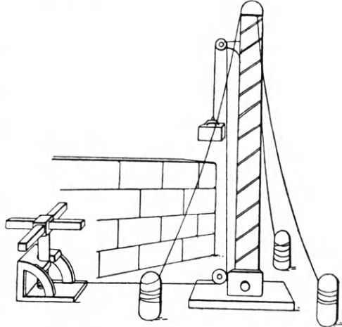
Εἰκ. 40. Ἀναπαράστασις μονοκώλου μηχανῆς κατὰ Ἡρώνα τὸν Ἀλεξανδρεῖα (Nix-Schmidt).
