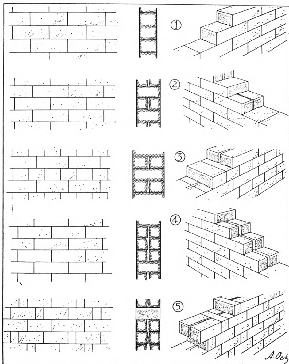
Είχ. 182. Διάφοροι παραλλαγαι του ὀρθογωνίου ἰσοδόμου συστήματος.
