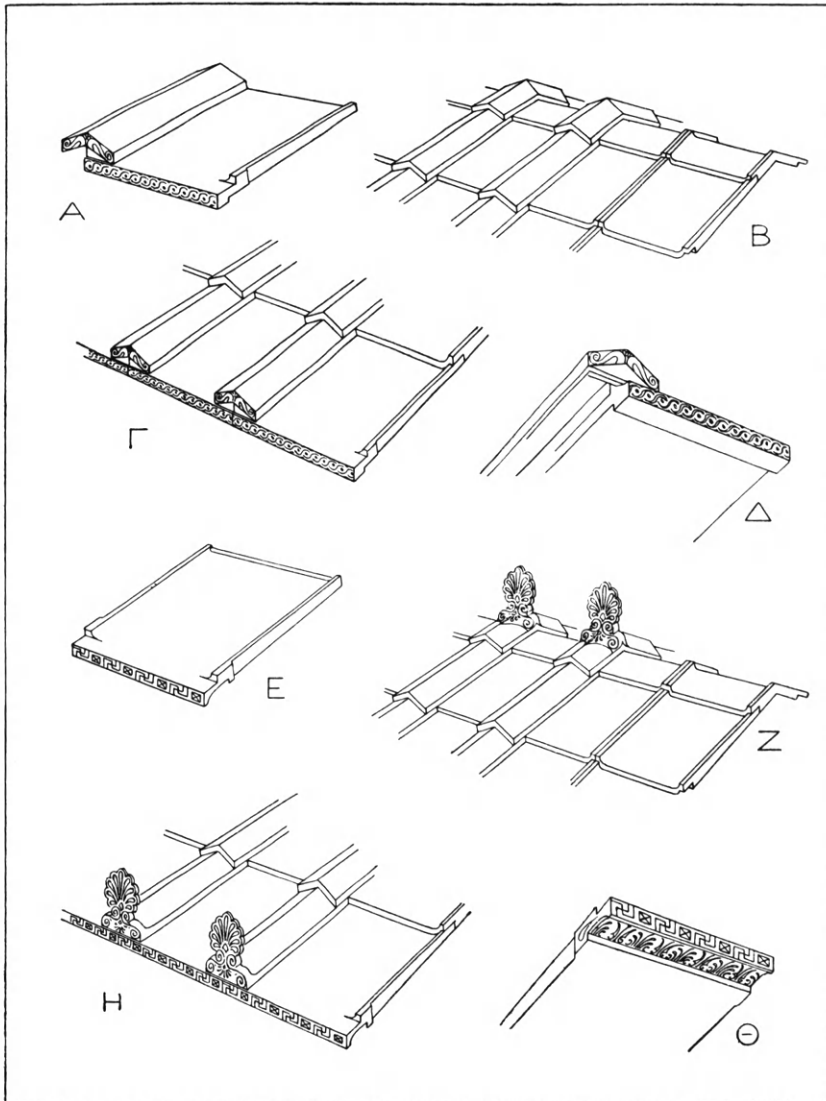
Εἰκ. 57. Πήλιναι κορινθιακοῦ τύπου κεραμίδες: Α, Γ ἀγελαῖαι, Β, Ζ κορυφαῖαι ἢ ἀμφίκυφοι καὶ Ε, Η, Θ ἡγεμόνες.
