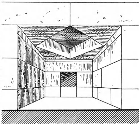
Εἰκ. 247. Προοπτικὴ ὄψις τῆς ὀροφῆς τοῦ προθαλάμου τοῦ τάφου τοῦ Μπελεβί (Weber).
