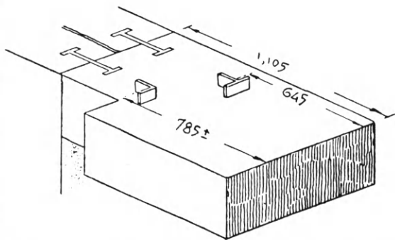
Εἰκ. 156. Γόμφοι σχήματος ταῦ καὶ γάμμα ἐπὶ λίθων τοῦ ἐν Δήλῳ ναοῦ τῶν Ἀθηναίων (Courby).
