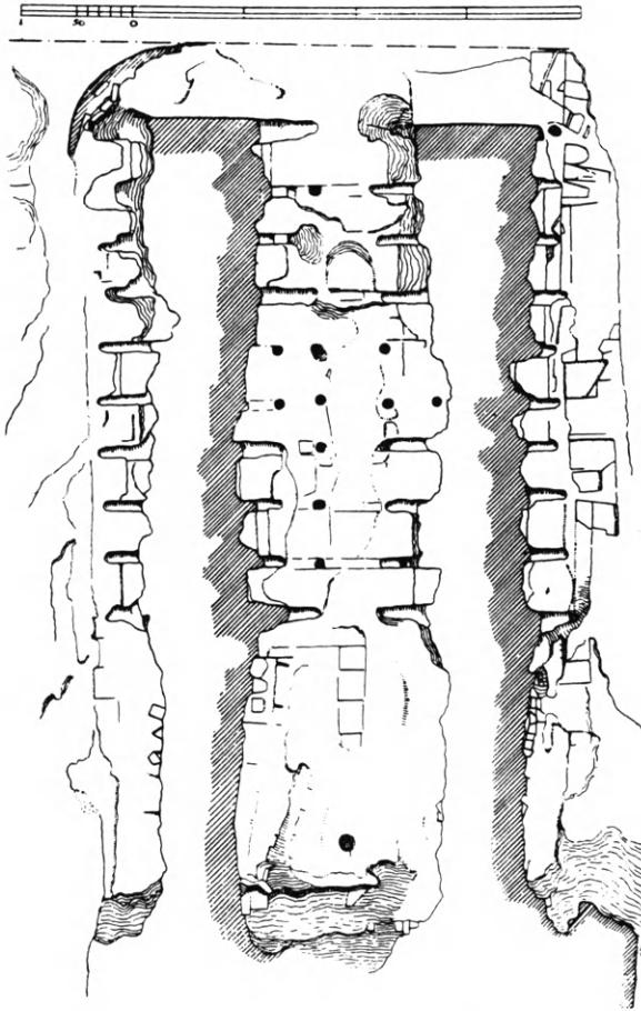
Εἰκ. 41. Κάτοψις κεραμικοῦ κλιβάνου τῆς ἀρχαίας Κορίνθου (Gl. Weinberg).
