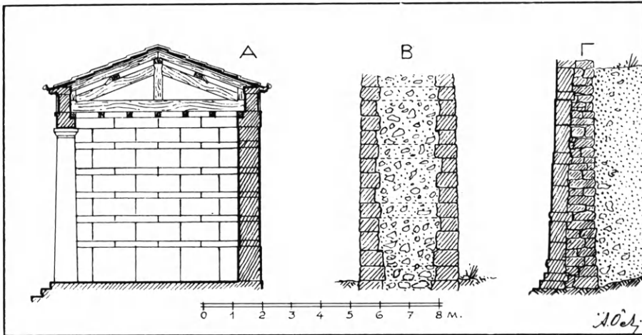
Εἰκ. 163. Συγκριτικὴ εἰκὼν πάχους : τοῖχου (Α), τείχους (Β) καὶ ἀναλήμματος (Γ).
