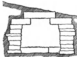
Εἰκ. 260. Τομὴ προμυκηναϊκοῦ τάφου τῆς Σύρου καλυπτομένου δι' ἐκφορικῶν πλακῶν (Bosanquet).
