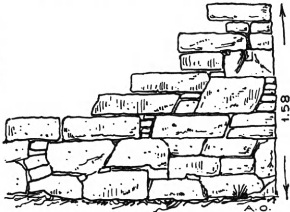
Εἰκ. 176. Δεῖγμα ἀκανονίστου τραπεζιοσχήμου συστήματος μετὰ ὀδοντώσεων καὶ βυσμάτων ἐκ Ραμνοῦντος (Ὁρλάνδος).
