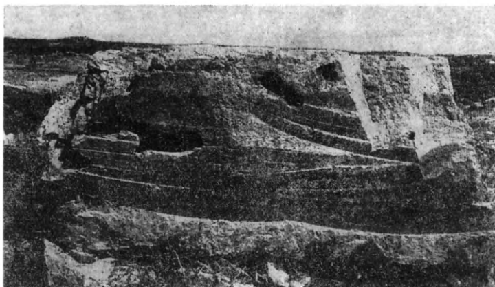
Εἰκ. 68. Ἴχνη τοῦ λιθοπρίονος ἐπὶ τῆς δυτικῆς παραστάδος τοῦ μεγάλου προπύλου τοῦ ἀνακτόρου τῆς Τίρυνθος (K. Müller).
