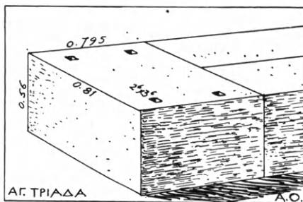
Εἰκ. 142. Τόρμοι γόμφων ἐπὶ παραστάδος τῆς 2 ας φάσεως τῆς μινωικῆς ἐπαύλεως Ἀγ. Τριάδας Κρήτης.
