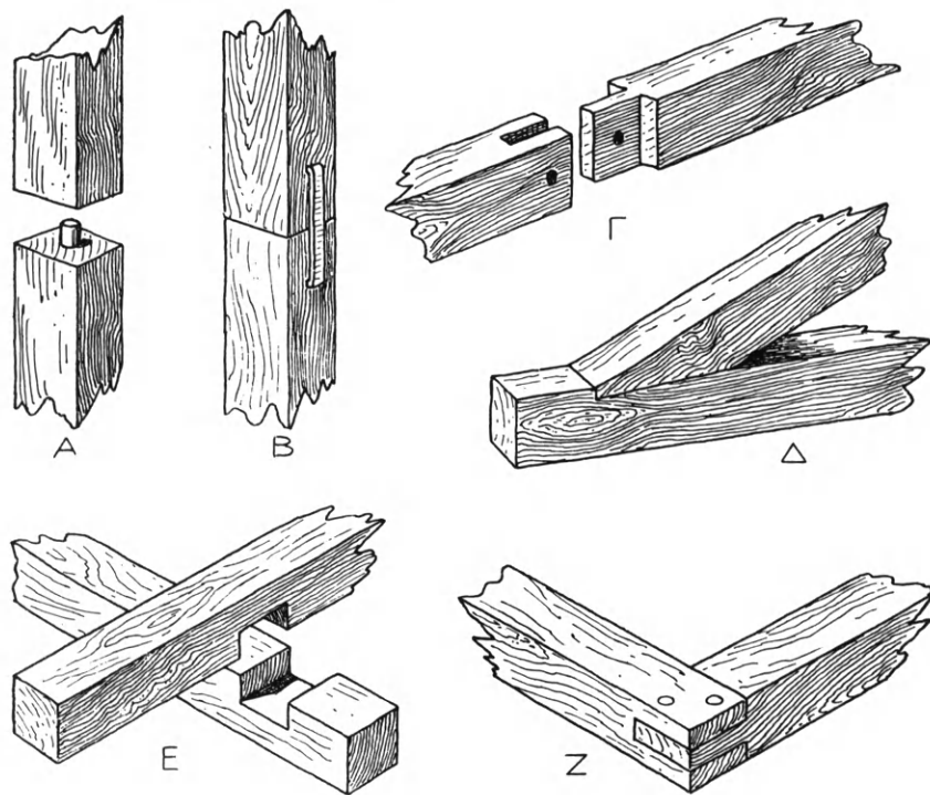
Εἰκ. 33. Διάφορα εἶδη συνδέσεως καὶ πήξεως τῶν ξύλων.
