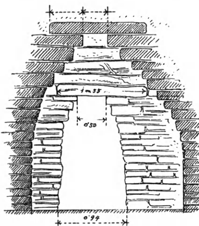
Εἰκ. 278. Τομὴ τοῦ τάφου τῆς Cortona (Durm).
