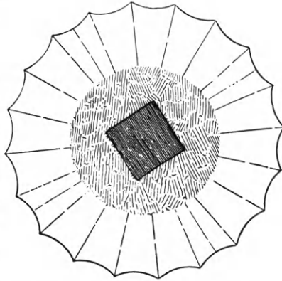
Εἰκ. 98. Σημεῖαι ἀξόνων καὶ ἀκτίνων τῶν ραβδώσεων ἐπὶ σφονδύλων τοῦ δωρικοῦ θησαυροῦ τῆς Μαρμαριᾶς τῶν Δελφῶν (Daux).
