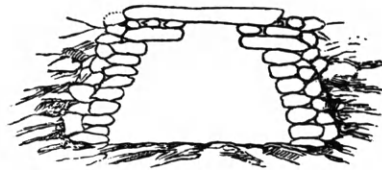
Εἰκ. 258. Τομὴ προμυκηναϊκοῦ τάφου τῆς Σύρου καλυπτομένου διὰ βαθμιδωτῶν ἐκφορικῶν πλακῶν ἐπὶ κεκλιμένων τοιχωμάτων (Τσοῦντας).
