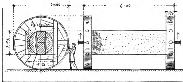
Εἰκ. 35. Τρόπος μεταφορᾶς τῶν ἐπιστυλίων τοῦ ἐν Ἐφέσῳ ναοῦ τῆς Ἀρτέμιδος ἐπινοηθεὶς ὑπὸ Χερσίφρονος καὶ Μεταγένους κατὰ Βιτρούβιον.
