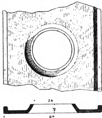
Εἰκ. 61. Πηλινὴ ὀπαία κεραμὶς ἐκ Πριήνης (Wiegand-Schrader).
