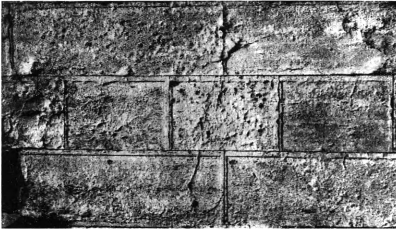
Εἰκ. 213. Τὸ Δ. ἀνάλημμα τοῦ θεάτρου τοῦ Διονύσου. Λίθοι μετὰ περιτενείας τοποθετημένοι ἐναλλάξ φορητὸν καὶ παρὰ μήκος (Ὁρλάνδος).
