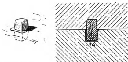
Εἰκ. 144. Ξύλινος γόμφος μετὰ μολυβδίνου μανδύου ἐκ τοῦ ἐν Δήλῳ ναοῦ τοῦ Ἀπόλλωνος (Courby).
