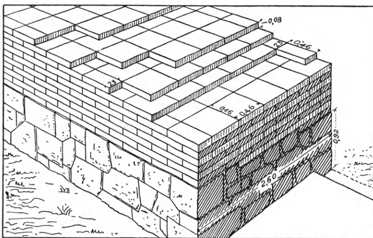
Εἰκ. 37. Ὡμαὶ πλίνθοι ἐπὶ λιθολογήματος ἐκ τοῦ ἀνατολ. περιβόλου τοῦ ἱεροῦ τῆς Ἐλευσίνος. Σύστημα δομῆς διὰ πλίνθων καὶ ἡμιπλινθίων (Ἀναπαράστασις Ὁρλάνδου).
