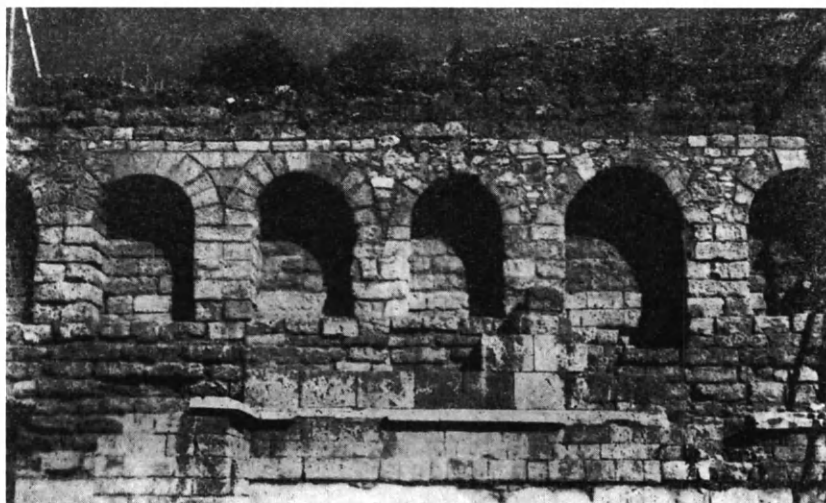
Εἰκ. 365. Ὁ ὀπισθεν τῆς ἐν Ἀθήναις στοᾶς τοῦ Εὐμένους τοξωτὸς ἀναλημματικὸς τοίχος.
