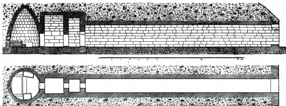
Εἰκ. 287. Κάτοψις καὶ τομὴ τοῦ θολωτοῦ τάφου τοῦ Μάλ-Τεπέ τῆς Θράκης (Filow).
