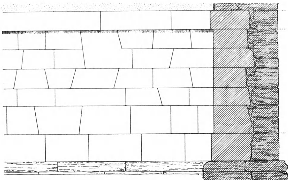
Εἰκ. 180. Δεῖγμα ἰσοδόμου τραπεζιοσχήμου συστήματος. Ὑπόστυλος αἵθουσα τῆς Δήλου (Leroux).
