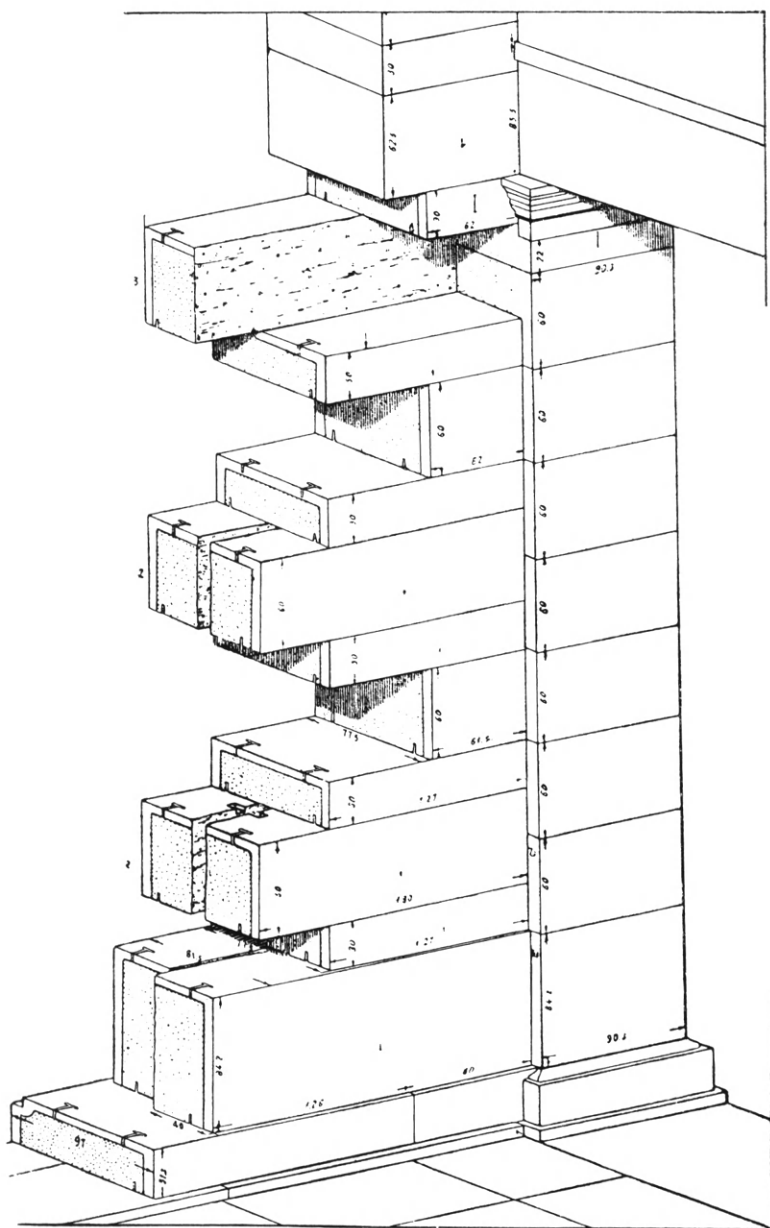
Εἰκ. 188. Μακροὶ τοῖχοι τοῦ σηκοῦ τοῦ ἐν Σουνίῳ ναοῦ τοῦ Ποσειδῶνος, συντεθειμένοι ψευδισοδόμῳ, κατ' ἰωνικὴν πιθανῶς ἐπίδρασιν. Περίπτωσις 1 τῆς εἰκόνης 187 (Ὁρλάνδος).
