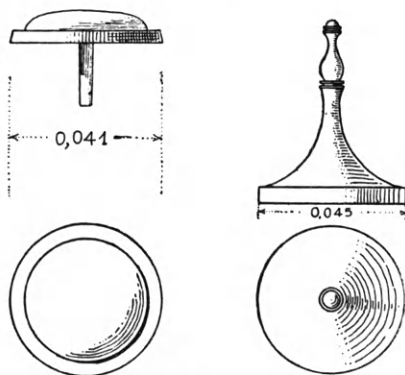
Εἰκ. 5. Ἐφηλίδες ἐκ Μεσσήνης καὶ Δήλου.
