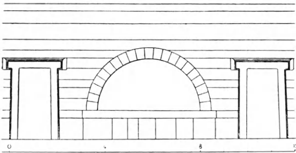
Εἰκ. 363. Τὸ ἡμικυκλικὸν παράθυρον τοῦ Ἐκκλησιαστηρίου τῆς Πριήνης (Wiegand - Schrader).
