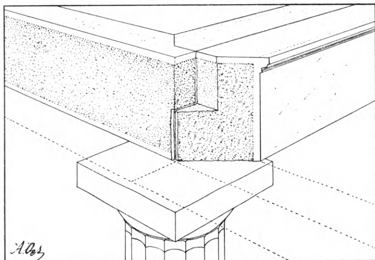
Εἰκ. 196. Προοπτικὴ ἄποψις τῆς συναντήσεως τῶν ἀντιθημάτων τῶν ἐξωτερικῶν ἐπιστυλίων τοῦ περὶ τοῦ ναοῦ τοῦ Ποσειδῶνος πρὸς τὸ καθέτως ἐπ' αὐτῶν βαῖνον διλιθικὸν ἐπιστύλιον, ὅπερ συνεχίζει τὸ ἐπιστύλιον τοῦ προνάου μέχρι τοῦ περὶ τοῦ (Ὁρλάνδος).
