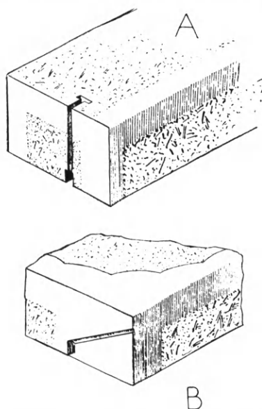
Εἰκ. 152. Α κατακόρυφος καὶ Β λοξὴ αὐλαξ μολυβδοχοΐας τοῦ 2ου ναοῦ τοῦ Ἀπόλλω- νος Δελφῶν (Courby).
