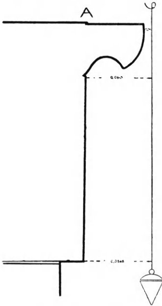
Εἰκ. 104. Δωρικὸν κυμάτιον τοῦ Παρθενῶνος δεικνύον ἐπὶ τῆς ἄνω αὐτοῦ ἐπιφανείας προφυλακτικὴν ταινίαν, Α. (Ὁρλάνδος)
