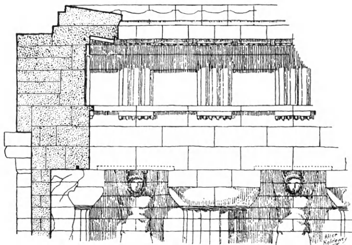
Εἰκ. 10. Ἐνίσχυσις τῶν ἐπιστυλίων τοῦ Ὀλυμπείου τοῦ Ἀκράγαντος διὰ σιδηρῶν δοκῶν (Koldewey - Puchstein).
