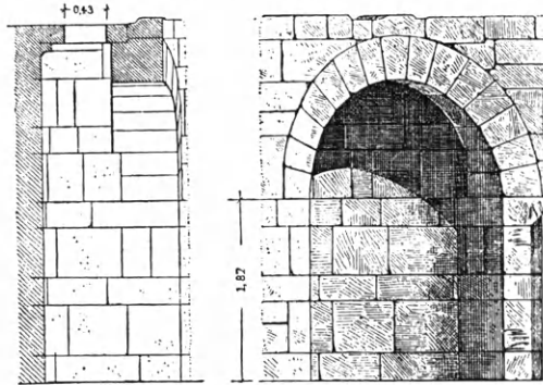
Εἰκ. 369. Μία τῶν τοξωτῶν ἀψίδων τῆς ὑπὸ τὸν μέγαν βωμὸν τοῦ Περγάμου μεγάλης ἡμικυκλῆς κόγχης (Schrammen).
