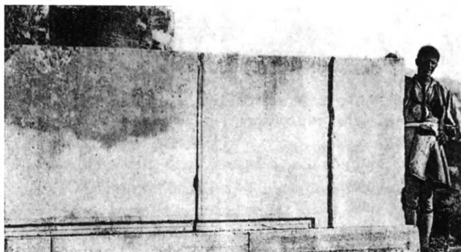
Εἰκ. 221. Ναὸς Διὸς Στράτου. Ὁρθοστάται τοῦ σηκοῦ μετὰ περιτενεῖας καὶ ὑποτομῆς (Φωτογρ. Γερμαν. Ἀρχαιολογικοῦ Ἰνστιτούτου Ἀθηνῶν).
