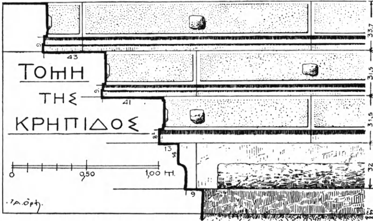
Εἰκ. 222. Ναὸς Διὸς Στράτου. Διαμόρφωσις τῶν λίθων τῆς κρηπίδος μετὰ περιτενείας, ὑποτομῶν καὶ ἀγκώνων (Ὁρλάνδος).
