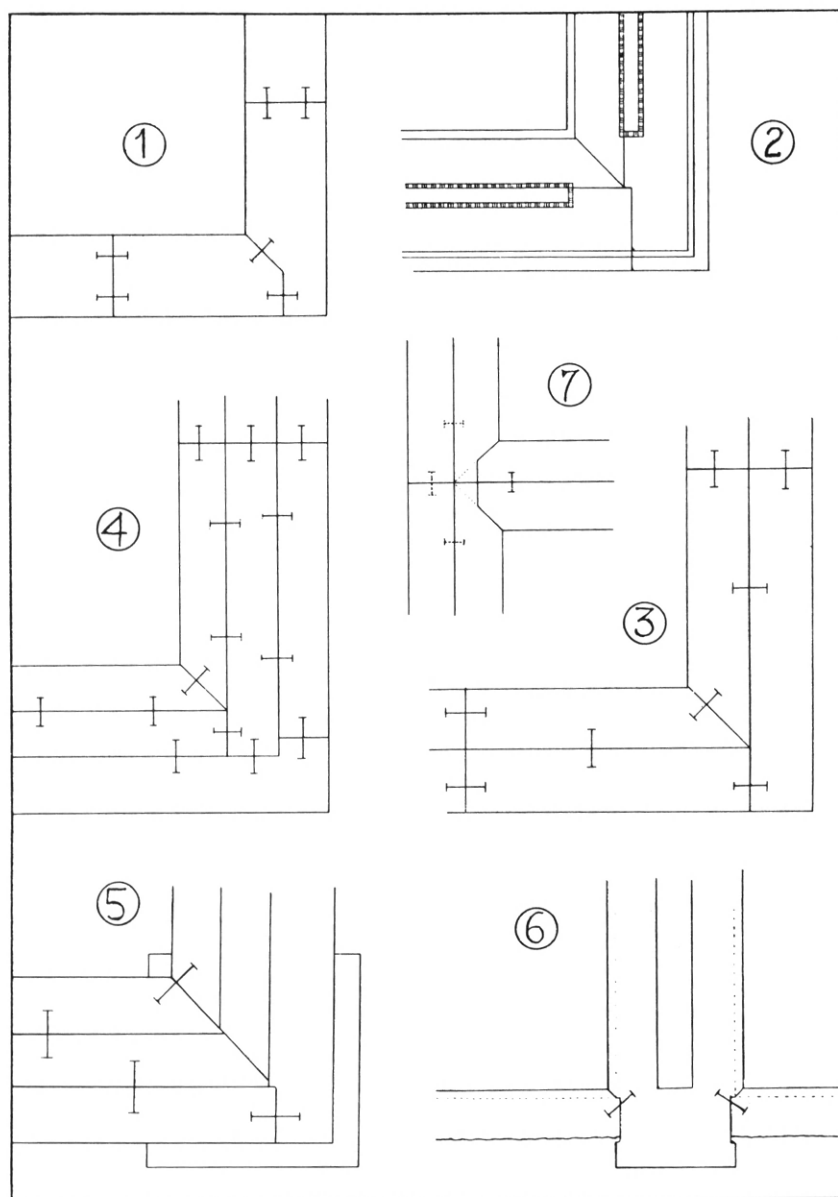
Εἰκ. 192. Τρόποι συναρμογῆς ἐπιστυλίων καὶ δοκῶν ὀροφῆς. 1 σηκοῦ μεγ. ναοῦ Ἀπόλλωνος Δήλου, 2 ναοῦ Ἀθηνᾶς Πριήνης, 3 ναοῦ Ἀφαίας, 4 Παρθενῶνος, 5 ναοῦ Διὸς Ὀλυμπίας, 6 δοκῶν ὀροφῆς Παρθενῶνος, 7 ἐπιστυλίων ναοῦ Ποσειδῶνος Σουνίου.
