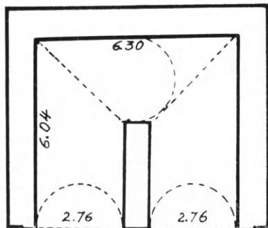
Εἰκ. 367. Κάτοψις τῆς ἐν Δελφοῖς θολωτοῦς ἐξέδρας Ἀττάλου τοῦ Α'.
