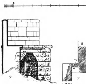
Εἰκ. 311. Τραπεζιόσχημον τόξον κόγχης θυρίδος τῶν τειχῶν τῆς Ἡρακλείας (Krischen).
