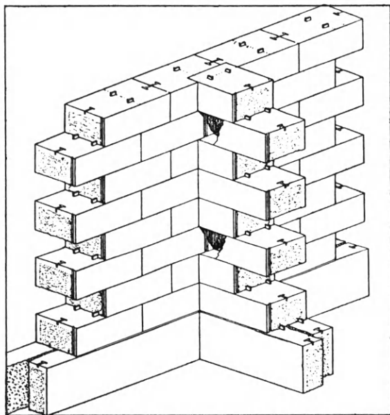
Εἰκ. 199. Συνένωσις μακροῦ πρὸς ἐγκάρσιον τοῖχον τοῦ «Θησείου» (Koch).
