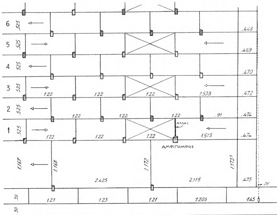
Εἰκ. 154. Σύστημα γομφώσεως τῆς ΒΔ. γωνίας τοῦ σηκοῦ τοῦ Παρθενῶνος. Τὰ βέλη δεικνύουσι τὴν φορὰν τοποθετήσεως τῶν λίθων, ἐξ ὧν οἱ μετὰ διαγωνίων γραμμῶν σημειούμενοι κατεβιβάζοντο τελευταῖοι (Ὁρλάνδος).
