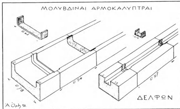
Εἰκ. 16. Μολύβδινα ἀρμοκαλύπτραι ἐκ Δελφῶν.
