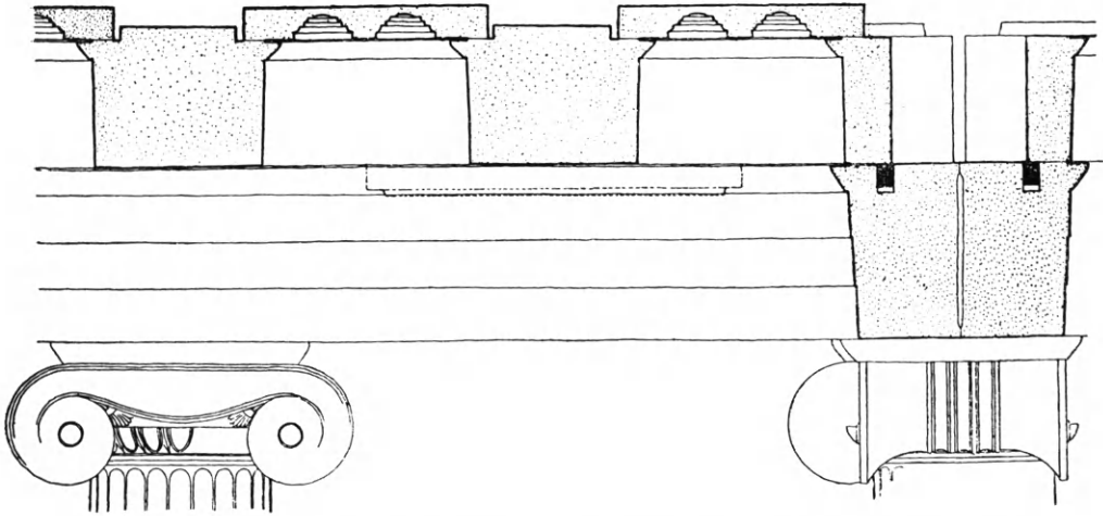
Εἰκ. 9. Σιδεραὶ δοκοὶ ἐνισχύσεως τῶν ἰωνικῶν ἐπιστυλίων τῶν Προπυλαίων τῆς Ἀκροπόλεως.
