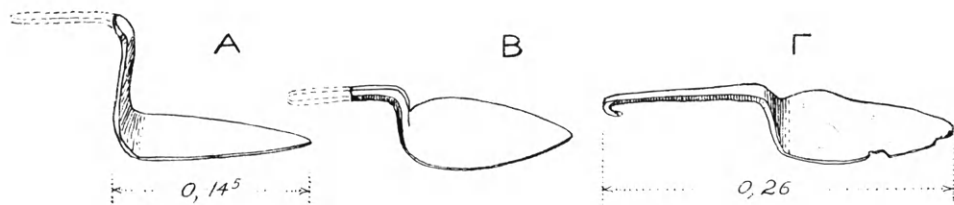
Εἰκ. 20. Τρία δείγματα ὑπαγωγέων (μυστρίων). Α ἐκ Λαυρίου, Β ἐκ Φθιωτίδων Θηβῶν, Γ ἐκ Τσαριτσίν Γκράδ (Ὁρλάνδος).
