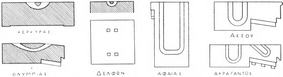
Εἰκ. 120. Διαμπερεῖς ὅπαι ἀνυψώσεως τῶν λίθων σχήματος ἀνοικτοῦ υ.
