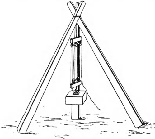
Εἰκ. 42. Ἀναπαράστασις τριβάλου μηχανῆς κατὰ Ἡρώνα τὸν Ἀλεξανδρεά (Nix-Schmidt).
