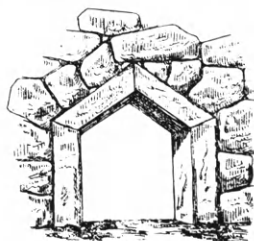
Εἰκ. 342. Ἡ πύλη τοῦ τείχους τῆς Ἀλέας (ἀριστερᾷ κατὰ Ραγκαβῆν, δεξιᾷ κατὰ Perrot).
