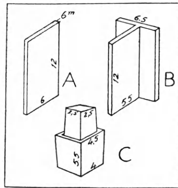
Εἰκ. 150. Διάφορα σχήματα γόμφων. A συνήθεις, B σχήματος ταῦ, C γόμφοι μετὰ χοινικίδος (Ὁρλάνδος).
