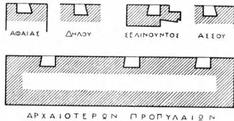
Εἰκ. 127. Ὅπαι ἀνελεύσεως τῶν λίθων διὰ λύκου.
