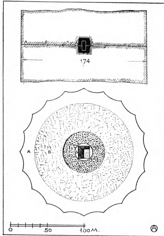
Εἰκ. 132. Κυκλικὴ ἀναθύρωσις σφονδύλων τοῦ Παρθενῶνος (Ὁρλάνδος).
