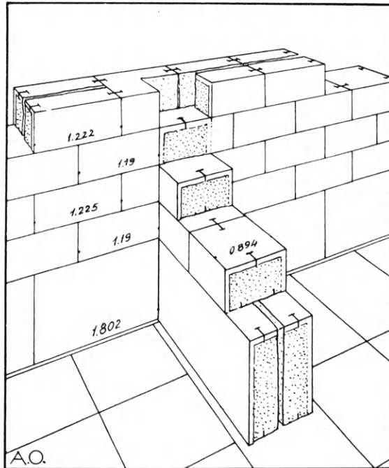
Εἰκ. 198. Συνάντησις τοῦ ἐγκαρσίου πρὸς τὸν μακρὸν τοίχον τοῦ σηκοῦ τοῦ Παρθενῶνος (Ὁρλάνδος).
