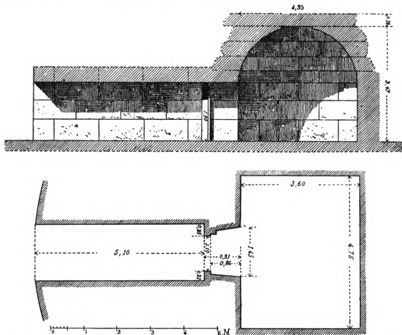
Εἰκ. 285. Κάτοψις καὶ κατὰ μῆκος τομὴ τοῦ παρὰ τὸ Γκερεσί τῆς Καρίας τάφου (Paton-Myres).
