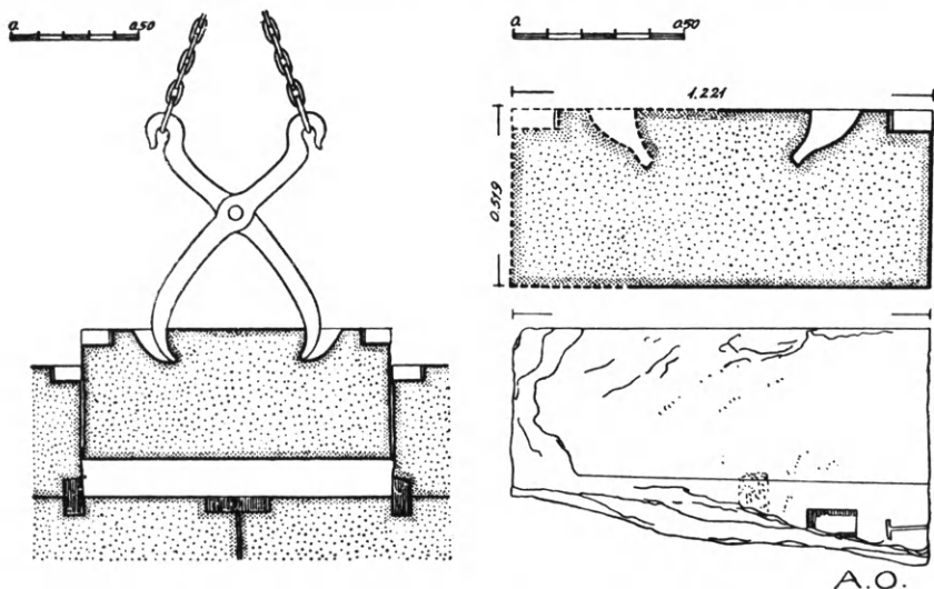
Εἰκ. 126. Καταβίβασις τοῦ τελευταίου λίθου στρώσεως τοῦ Παρθενῶνος τῇ βοηθείᾳ καρκίνου. (Ὁρλάνδος)
