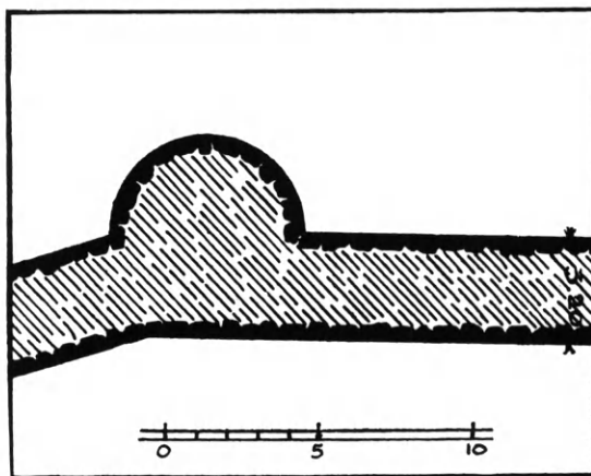
Εἰκ. 165. Ὀχυρωματικὸν τεῖχος τῆς ἀρχαίας Στυμ- φάλου μετὰ δύο παρειῶν (Ὁρλάνδος). (Ἀνασκαφὴ Ἀρχαιολ. Ἑταιρείας)
