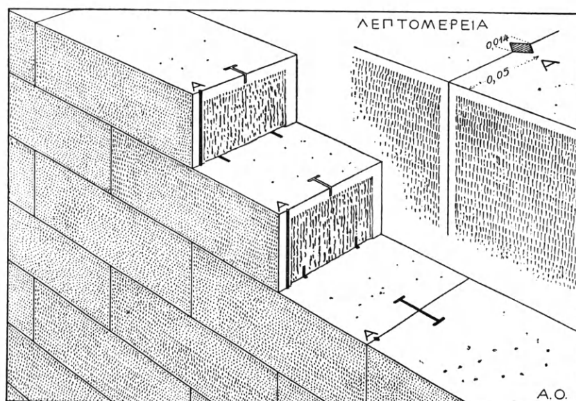
Εἰκ. 15. Οἱ μετὰ μονωτικῶν πλήρων μολύβδου αὐλάκων λίθοι τῶν τοίχων τοῦ σηκοῦ τοῦ «Θησείου» (Ορλάνδος).
