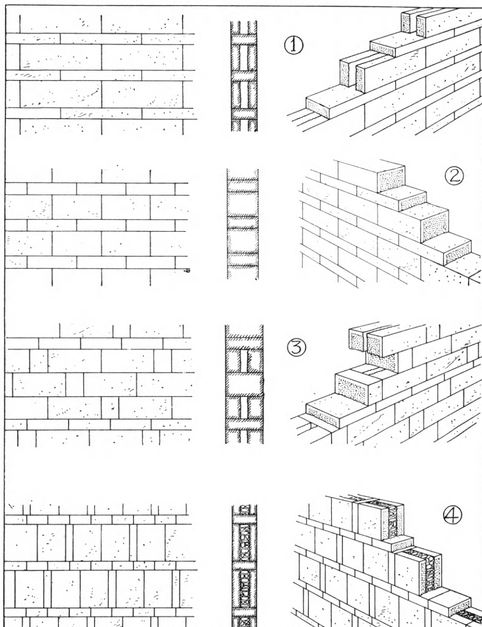
Είχ. 187. Διάφοροι παραλλαγὰι τοῦ ὀρθογωνίου ψευδοδομίου συστήματος (Όρθάνδος).
