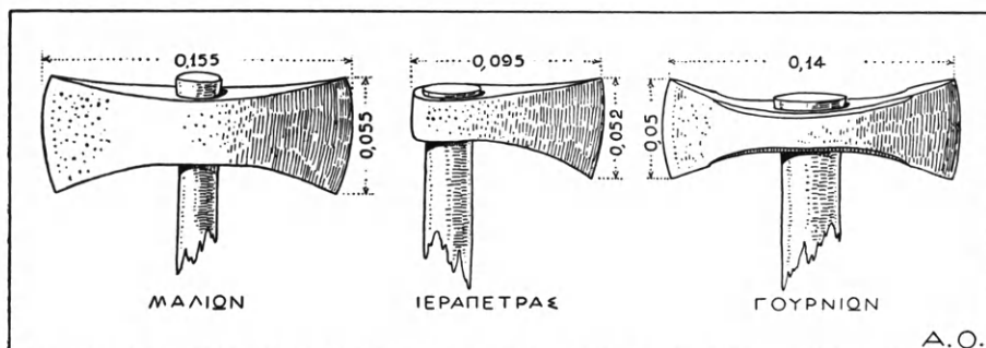
Εἰκ. 12. Χαλκοὶ, ὑστερομινωικοὶ, ἀπλοὶ καὶ διπλοὶ πελέκεις ἐκ Μάλλιων, Ἱεραπέτρας καὶ Γουρνιῶν τῆς Κρήτης. Οἱ στελεοὶ τῶν ἐν ἀναπαραστάσει ἐντὸς τῶν ὑπαρχουσῶν ὀπῶν.
