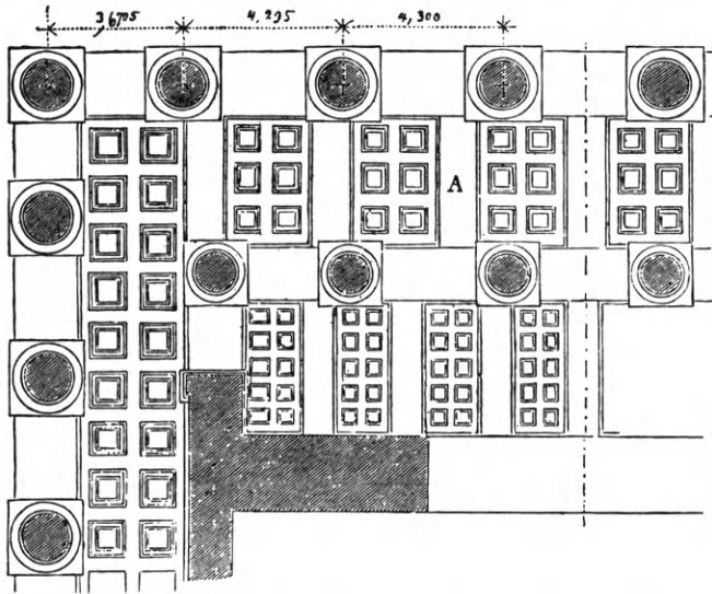
Εἰκ. 244. Ἀνοψις τῶν ὀροφῶν τοῦ Παρθενῶνος. Ἀριστερᾷ συνεχεῖς πλακοδοχοὶ μετὰ φατνωμάτων, δεξιᾷ δοκοὶ (A) μετ' ἐνδιαμέσων φατνωματικῶν πλακῶν.
