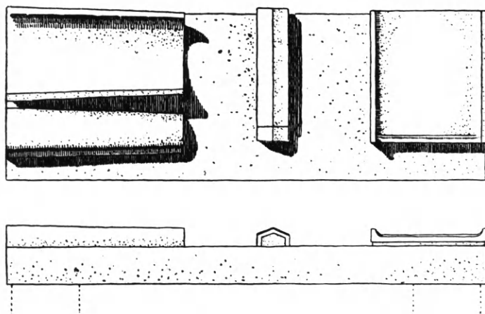
Εἰκ. 63. Μαρμαρίνον παράδειγμα πηλίνων λακωνικοῦ καὶ κορινθιακοῦ τύπου κεραμίδων ἐξ Ἀσσοῦ (Bacon).
