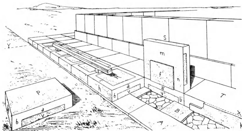
Εἰκ. 82. Ἀναπαράστασις ξυλίνου κανόνος βαίνοντος ἐπὶ κύβων στηριζομένου ἐπὶ τῆς περιτενεΐας τῶν καταστροφικῶν τοῦ παρὰ τὴν Λεβάδειαν ναοῦ τοῦ βασιλέως Διὸς (Choisy).
