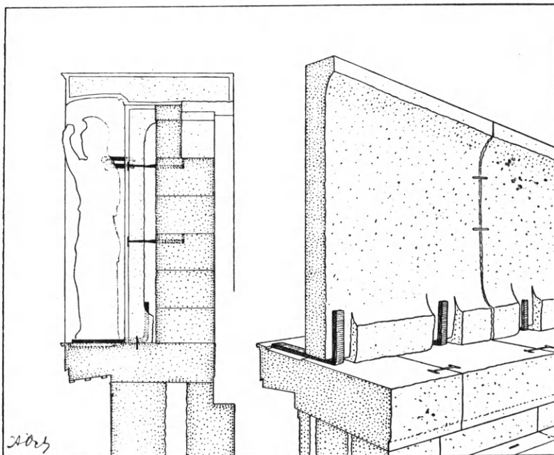
Εἰκ. 11. Σιδηραὶ δοκοὶ στηρίξεως τῶν ἐναετίων ἀγαλμάτων τοῦ Παρθενῶνος (Δυτ. ἀέτωμα) (Ὁρλάνδος).
