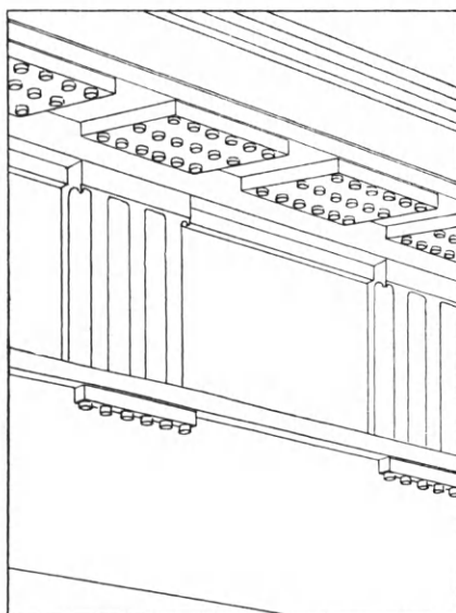
Εἰκ. 9. Κανόνες δωρικοῦ ἐπιστυλίου καὶ πρόμοχοι δωρικοῦ γείσου μετὰ σταγόνων.
