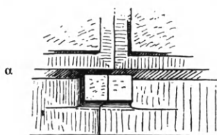
Εἰκ. 103. Προφυλακτικά τῶν ἀκμῶν ἐξογκώματα διακοσμητικῶς λαξευμένα εἰς τήν κρηπίδα τοῦ ἀρχαιότερου Παρθενῶνος (α), και τοῦ ναοῦ τῆς Ποσειδωνίας (β). (Durrm)
