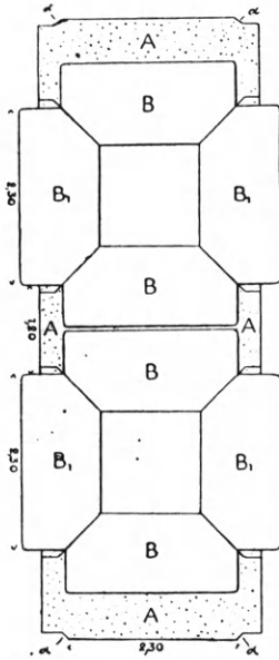
Εἰκ. 197. Φατνώματα τοῦ ἐν Πριή- νῃ ναοῦ τῆς Πολιάδος Ἀθηνᾶς (Wiegand - Schrader).
