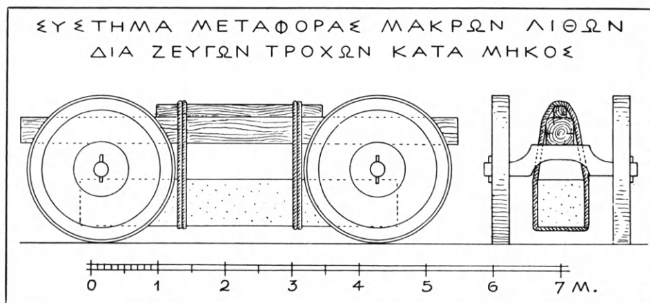
Εἰκ. 38. Πιθανὸς τρόπος μεταφορᾶς μακρῶν λίθων διὰ ζευγῶν τροχῶν τοποθετουμένων κατὰ μήκος.
