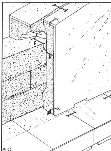
Εἰκ. 153. Τύμπανον ἀετώματος τοῦ Παρθε- νῶνος. α λοξὴ αὐλαξ μολυβδοχοΐας, β στρε- πτὸς σύνδεσμος σχήματος διπλοῦ ταῦ.
