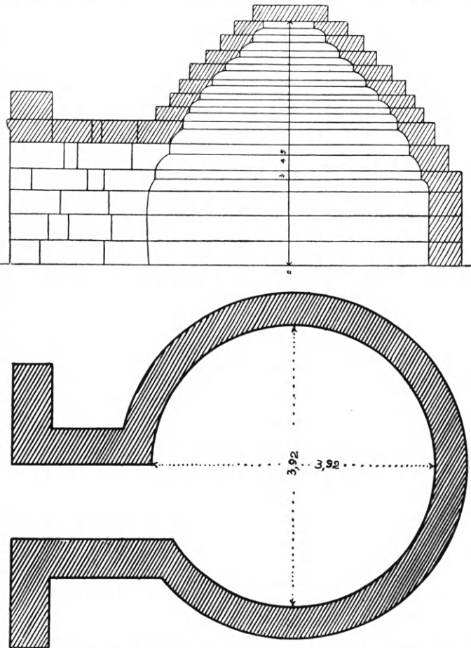
Εἰκ. 286 Κάτοψις καὶ κατὰ μῆκος τομὴ τοῦ ἐν Θράκῃ περιγκιπικοῦ τάφου τοῦ Κιρκ-Κιλησέ (Hasluck).
