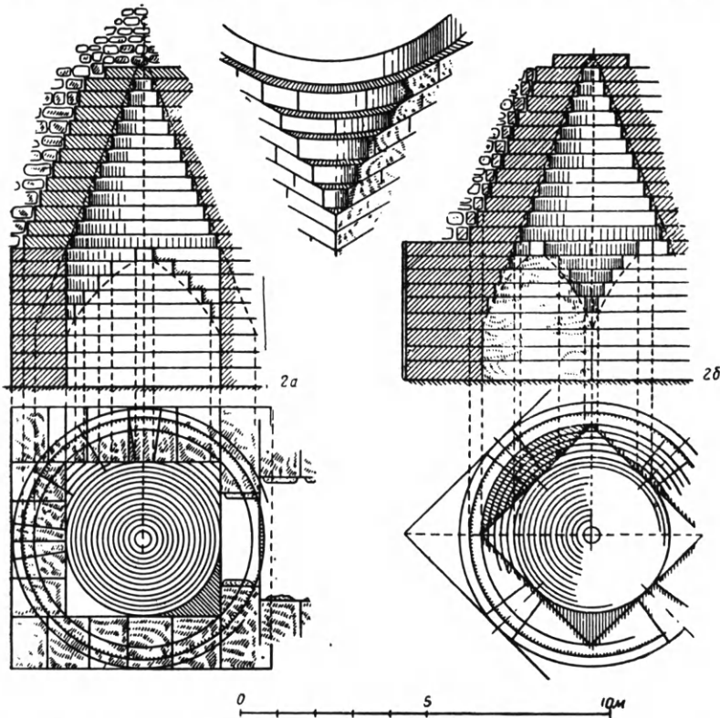
Εἰκ. 294. Ἀριστερᾶ: ὀριζοντία καὶ κατακόρυφος τομὴ τοῦ βασιλικοῦ τάφου τοῦ Παντικαπαίου βαίνουσα παραλλήλως πρὸς μίαν τῶν πλευρῶν τοῦ βασικοῦ τετραγώνου. Δεξιᾶ: Ὁριζοντία καὶ κατακόρυφος τομὴ τοῦ αὐτοῦ τάφου κατὰ τὴν διαγώνιον. Ἐν τῷ μέσῳ προοπτικὴ ἄποψις τοῦ λοφίου (Durm).
