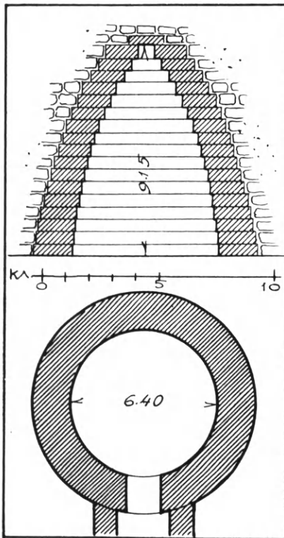
Εἰκ. 292. Κάτοψις καὶ κατακόρυφος τομὴ τοῦ παρὰ τὸ Παντικάπαιον χρυσοῦ τάφου.
