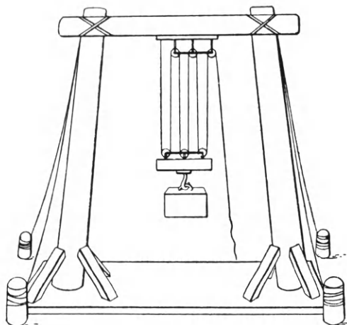
Εἰκ. 41. Ἀναπαράστασις δικώλου μηχανῆς κατὰ Ἡρώνα τὸν Ἀλεξανδρεῖα (Nix-Schmidt).
