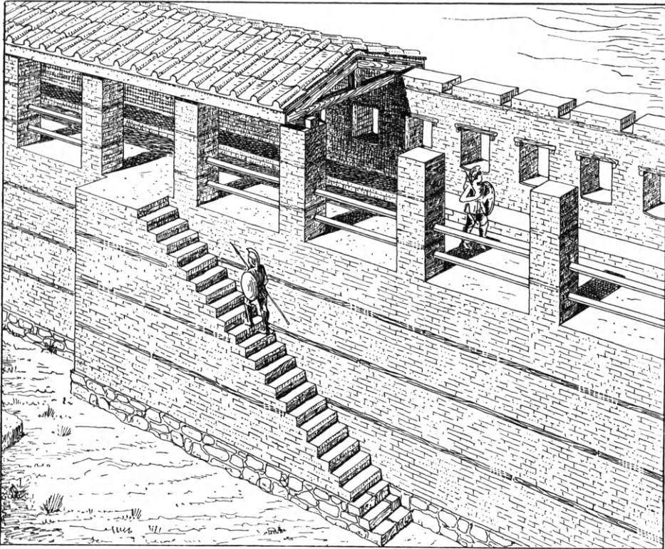
Εἰκ. 38. Ἀναπαράστασις τοῦ πλινθίνου τείχους τῶν Ἀθηνῶν μετὰ τῶν ἀναβασμῶν καὶ τοῦ στεγάσματος (Ὁρλάνδος).
