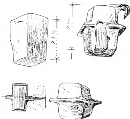
Εἰκ. 145. Ξύλινοι γόμφοι μετὰ μολυβδίνου μανδύου ἐκ τοῦ Διδυμείου τῆς Μιλήτου, νῦν ἐν τῷ μουσεῖῳ τοῦ Λούβρου (Durtm).
