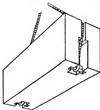
Εἰκ. 123. Ἰδιον σύστημα ἀνυψώσεως λίθων ναοῦ τοῦ Σελινοῦντος. (Koldewey)
