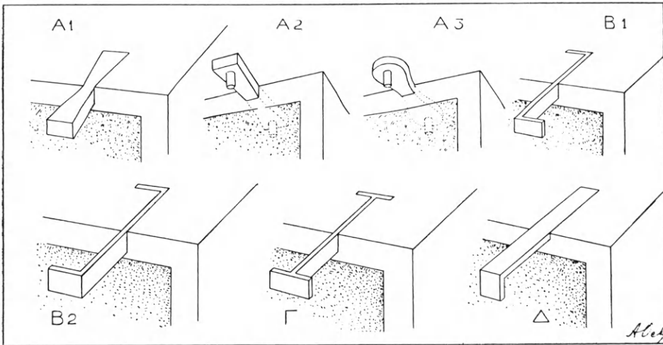
Εἰκ. 135. Σχήματα ὀριζοντίων συνδέσεων (Οῤολάνδος).
