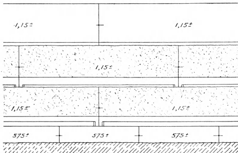
Εἰκ. 215. Ἡ κρητὶς τοῦ ἐν Δήλῳ μεγάλου ναοῦ τοῦ Ἀπόλλωνος (Courby).
