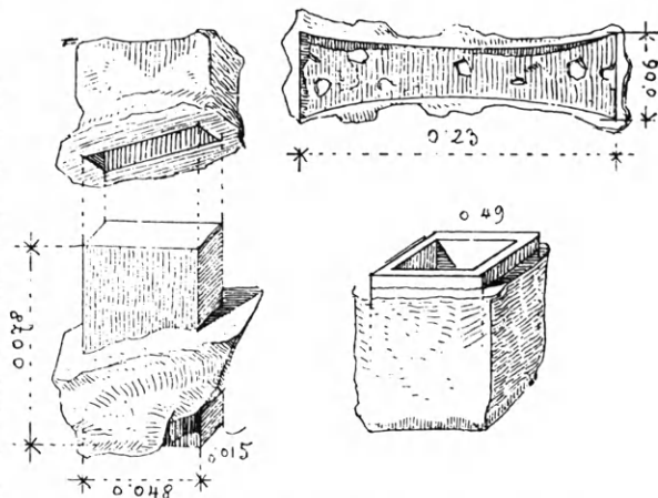
Εἰκ. 157. Ὁρειχάλκινοι γόμφοι μετὰ μολυβδίνου μανδύου ἐκ Σαμοθράκης (Durm).
