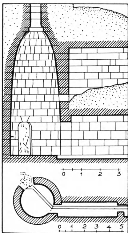
Εἰκ. 309. Ἡ ἐν Κῷ κρήνη Βούρινα. Κάτοψις καὶ κατακόρυφος τομή (Ross).
