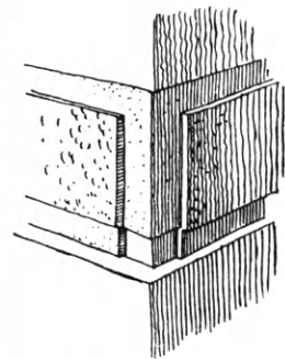
Εἰκ. 217. Γωνία μετὰ περιτενείας ναοῦ Ἡρας.
