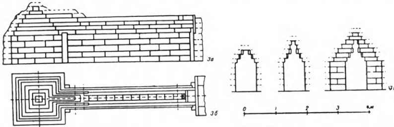
Εἰκ. 291. Τάφος Μελέκ-Τσεσμένσκ παρὰ τὸ Παντικάπαιον (4 ον ἢ 3 ον π.Χ. αἰ.). Ἀριστερᾶ: κάτοψις καὶ κατὰ μῆκος τομή. Δεξιᾶ: ἐγκάρσιαι τομαὶ τοῦ δρόμου τοῦ.
