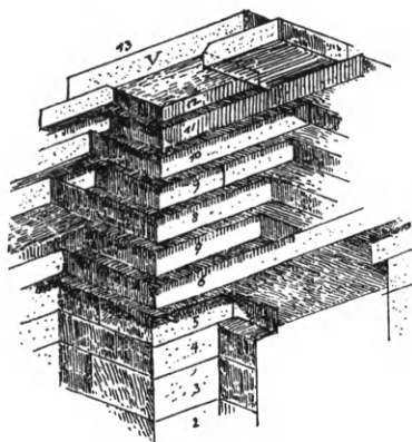
Εἰκ. 296. Προοπτικὴ ἀποψις ἐσωτερικῆς γωνίας τῆς πυραμιδοειδοῦς θόλου τοῦ τάφου Μελέκ - Τσεσμένσκ (Durm).
