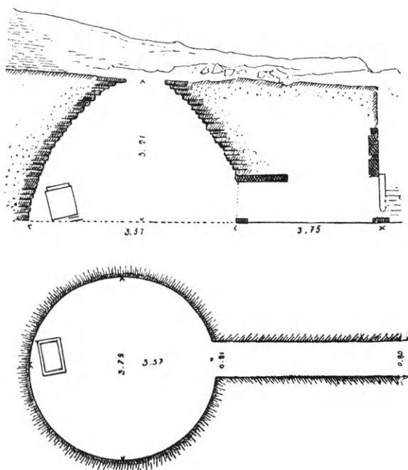
Εἰκ. 273. Κάτοψις καὶ τομὴ τῆς ἐκφορικῆς θόλου τοῦ τάφου τῶν Ἀρχάδων Κρήτης (8 ου αἰ.) (Levi).
