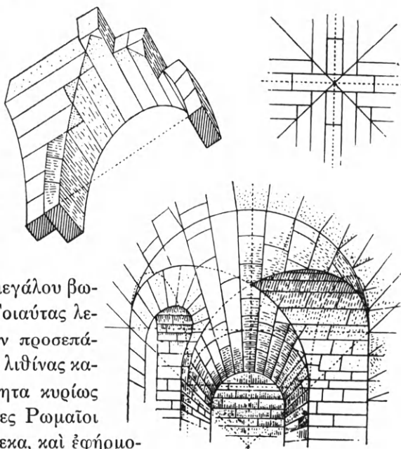
Εἰκ. 370. Θολωταὶ ὀροφαὶ τοῦ Περγάμου ἐκ λαξευτῶν λίθων. Διεισδύσεις καὶ ἡμισταυροθόλια (Durm).
