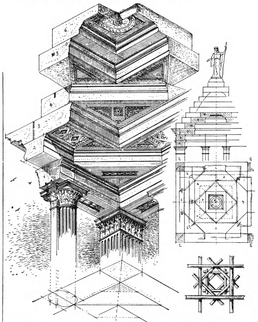
Εἰκ. 251. Ἐπιτύμβιον μνημεῖον Μυλάσων Καρίας. Ἀριστερᾷ: Προοπτικὴ ἄποψις τῆς ἐσωτερικῆς ὀροφῆς (Durtm). Ἀνω δεξιᾷ: Ἀνοψις καὶ τομὴ τῆς ὀροφῆς τοῦ αὐτοῦ μνημεῖου κατὰ Perrot. Κάτω δεξιᾷ: Ὁμοίου συστήματος διάταξις ξυλίνης ἀρμενικῆς ὀροφῆς.
