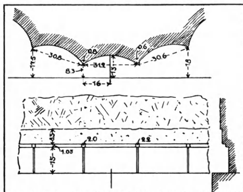
Εἰκ. 94. Ἡμιτελής σφόνδυλος τῆς Φιλωνίου στοᾶς τῆς Ἐλευσίνος.
