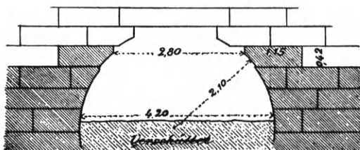
Εἰκ. 325. Ὑπόνομος τοῦ Ἡριδανοῦ Ἀθηνῶν (Ziller).
