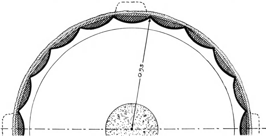
Εικ. 91. Ὄψω: φωτογραφικὴ ἀπόψις ἡμιτελοῦς κατωτάτου σφονδύλου τοῦ Παρθενῶνος II. Κάτω: ὁριζοντία τομὴ καὶ δευτέρα προβολὴ τοῦ ἡμίσεος τοῦ αὐτοῦ σφονδύλου. (Ὁρλάνδος)
