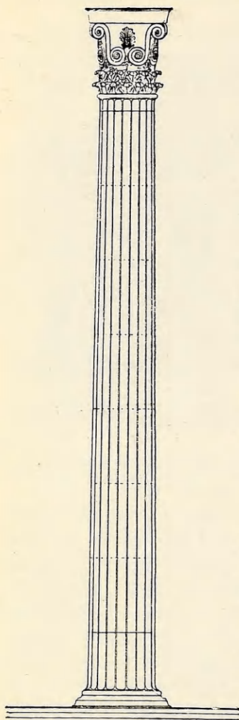
Εἰκ. 51. Κορινθιακὸς ἡμικίλιον ἐσωτερικὸς τῆς θόλου.
