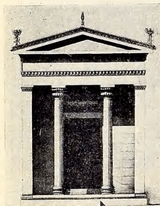
Εἰκ. 49. Ὁ αἰολικὸς ναῖσκος κατ' ἄλλην ἀναπαράστασιν.
