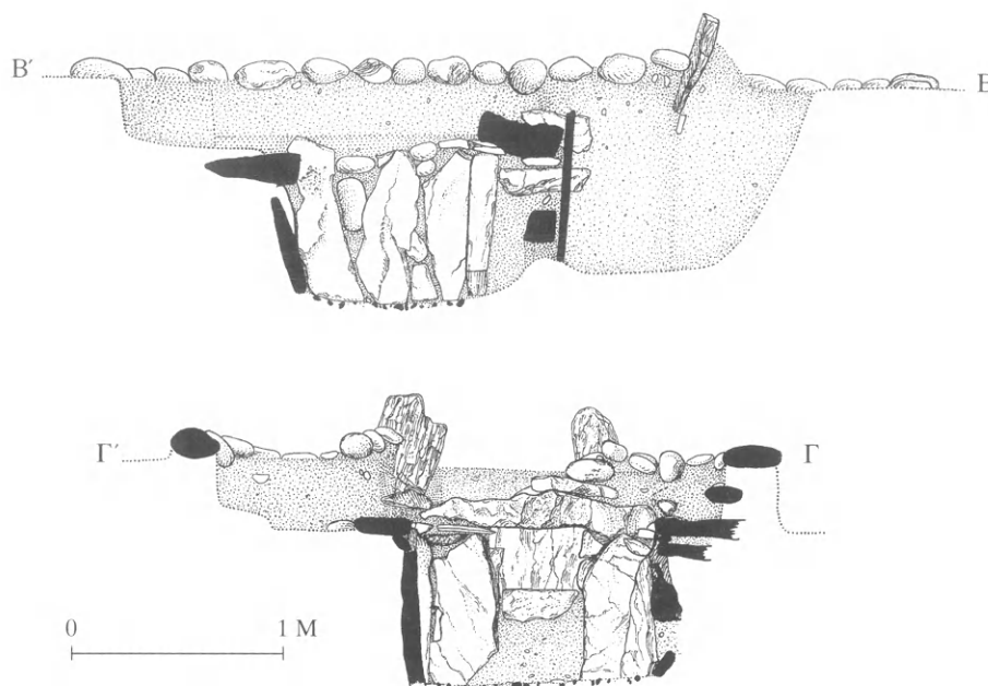
29. Τομή Β'-Β και τομή Γ'-Γ με ὄψη τῆς ἀνατολικῆς πλευρᾶς τοῦ τάφου 4.
