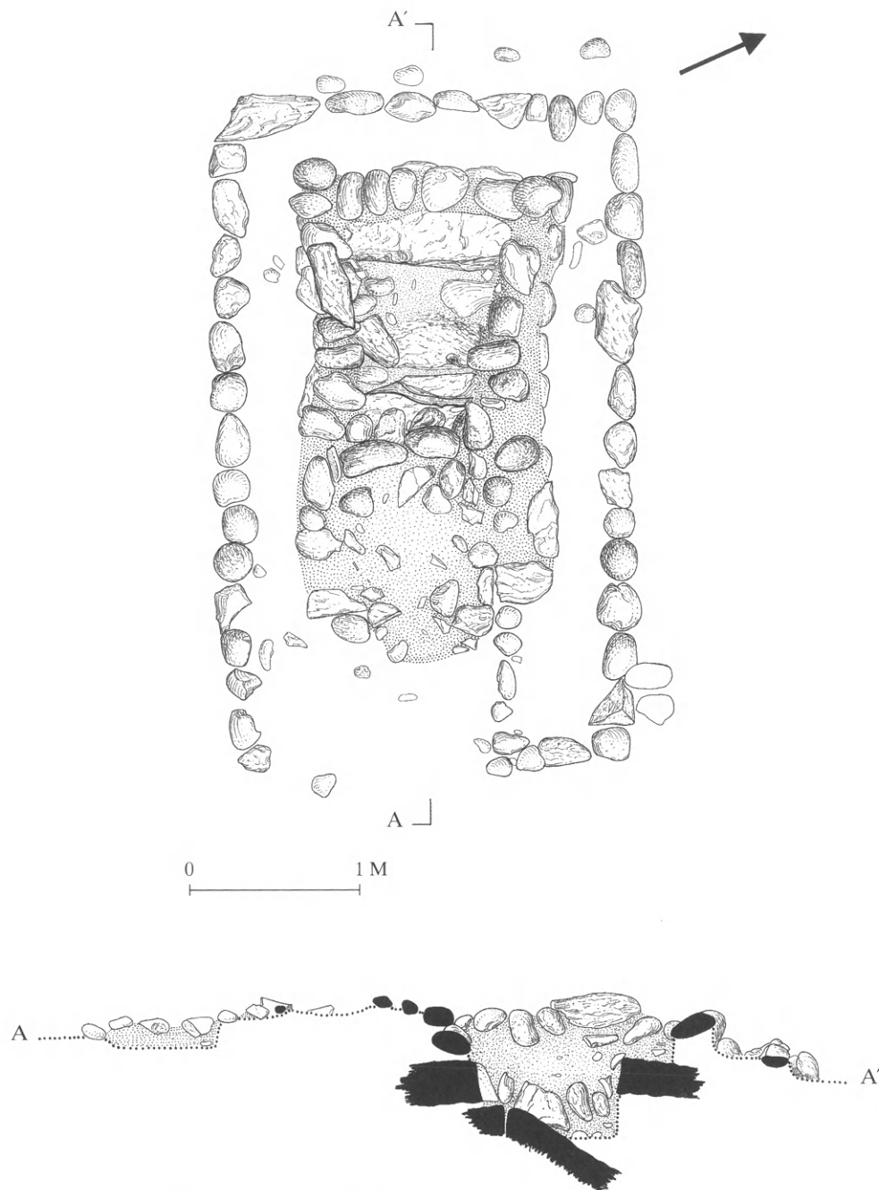
188. Κάτοψη και τομή Α-Α' τοῦ τάφου 30.
