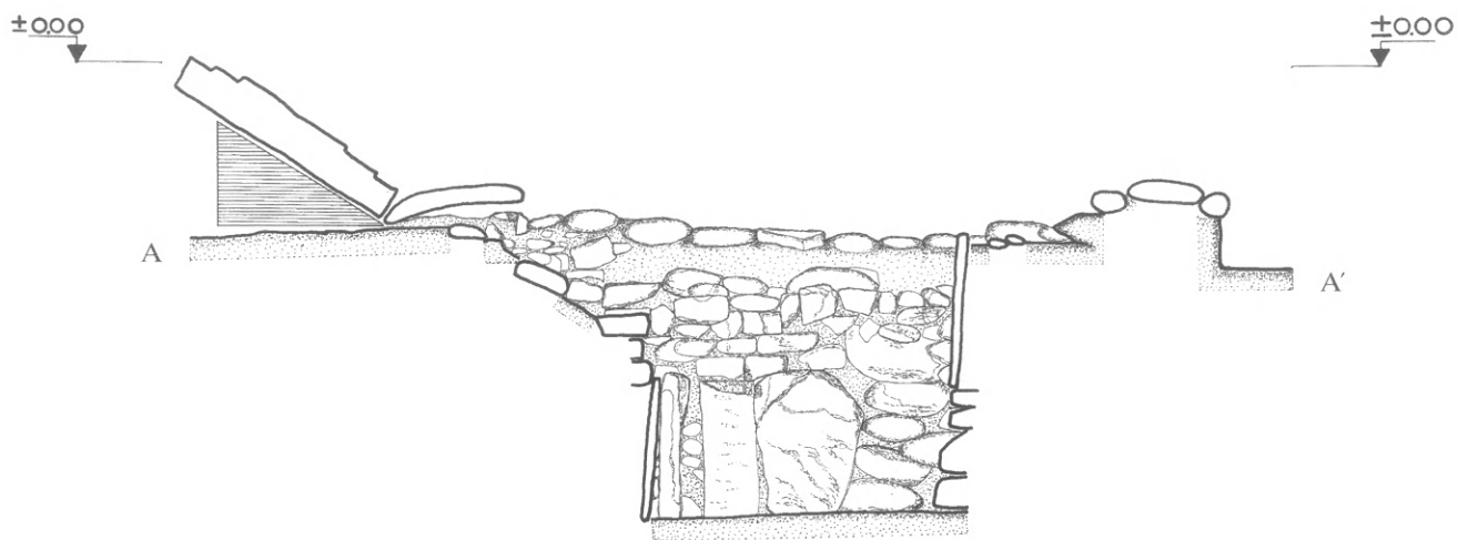
109. Τομή Α-Α' του τάφου 16.
