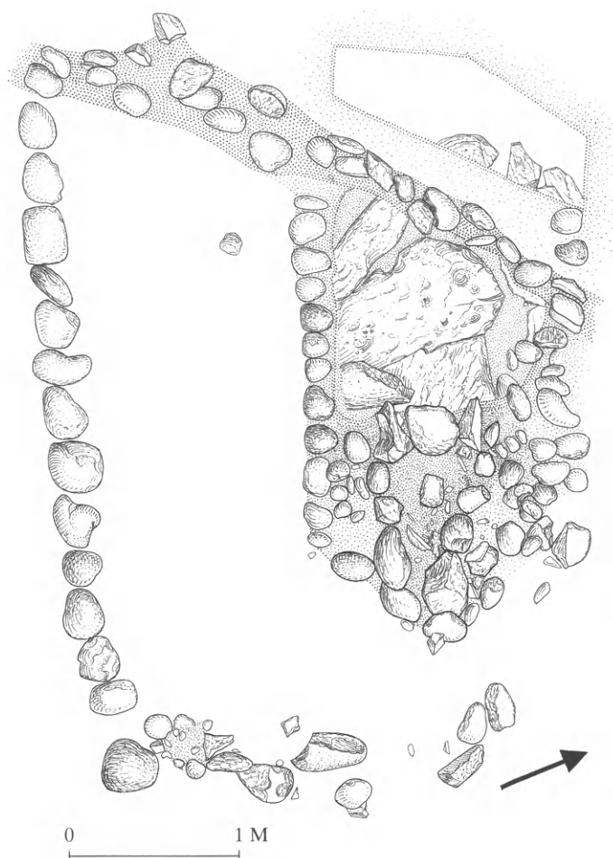
277. Κάτοψη του τάφου 57.
