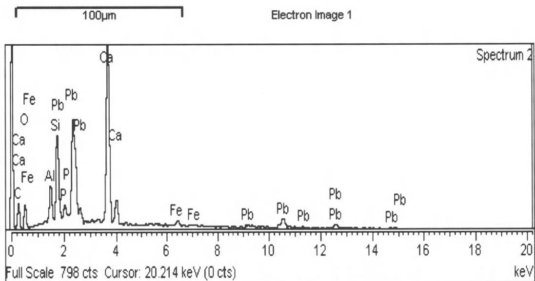
Εἰκ. 2. Σημειακή ἀνάλυση τῆς σκοτεινότερης φάσης, στὴν ὁποία συννύπάρχουν ἀργιλοπυριτικές ἐνώσεις καὶ λιθάργυρος σὲ λεπτὴ διασπορά.
