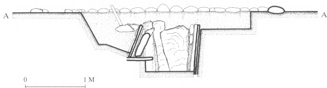
26. Τομή του τάφου 3 με άνεσκαμμένο πρόθυρο και την είσοδο κλειστή.
