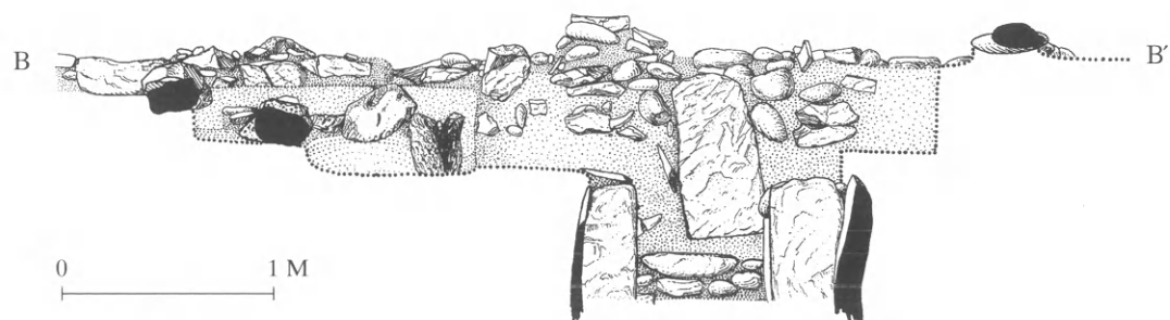
178. Τομὴ B-B' τῶν τάφων 27 καὶ 26.
