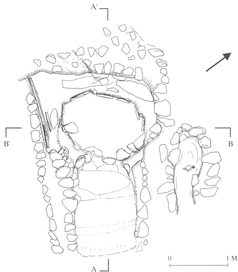
129. Κάτοψη τοῦ τάφου 19 καὶ τοῦ λάγκκου 19α μετὰ τὴν πλήρη ἀνασκαφὴ τους.
