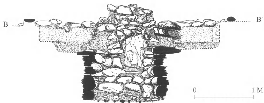
36. Ὁ λάκκος τοῦ τάφου 5. Ἐγκάρσια τομὴ B-B' μετὰ ὀψιν τῆς ἀνατολικῆς παρειᾶς.
