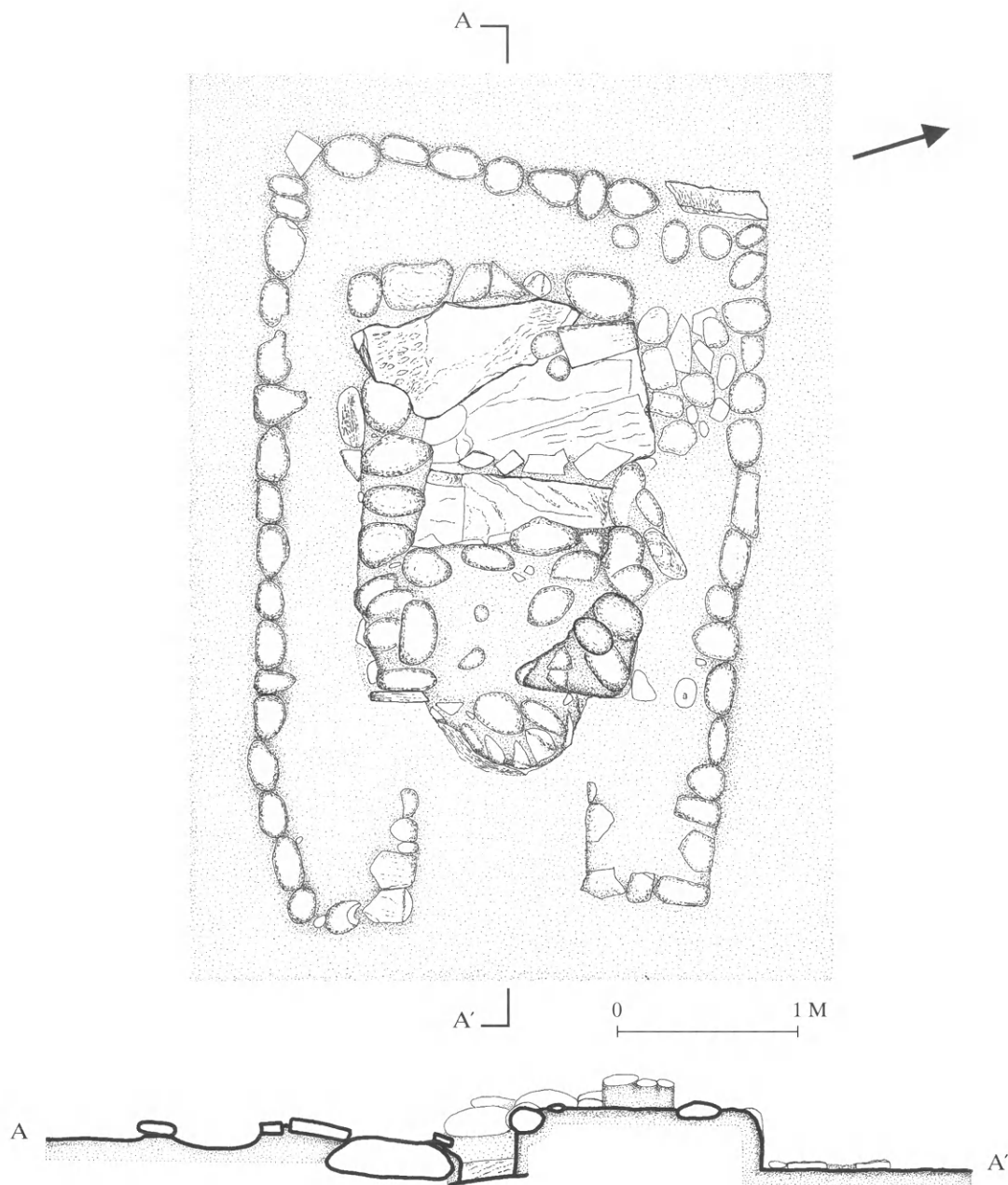
193. Κάτοψη και τομή Α-Α' του υπέργειου όρατου τμήματος του τάφου 33.
