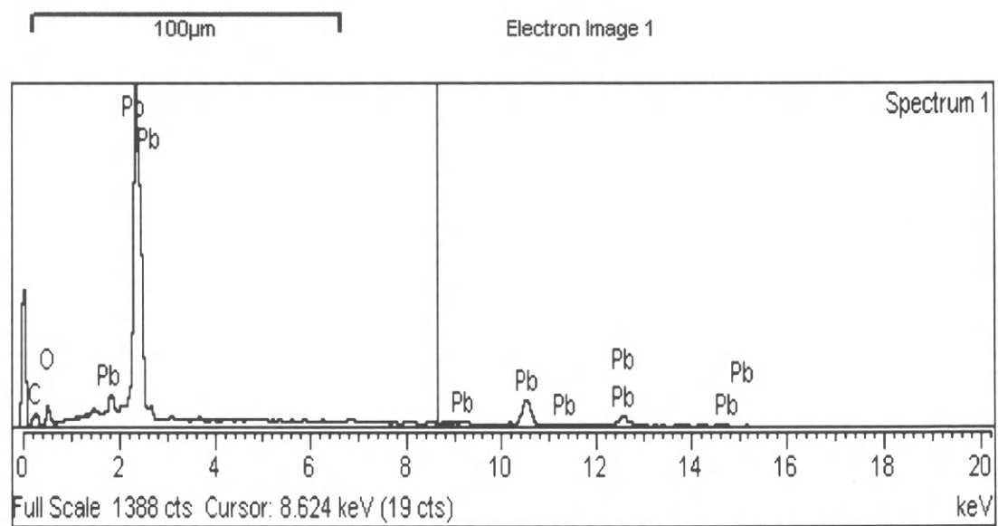
Εἰκ. 1. Σημειακή ἀνάλυση λιθαργύρου στὸ ἠλεκτρονικὸ μικροσκόπιο.
