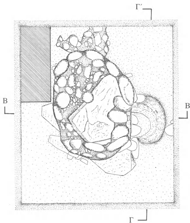
299. Κάτοψη τοῦ ἀνεσκαμμένου τμήματος τοῦ τάφου 65 καὶ τομὲς B-B' καὶ Γ-Γ'.
