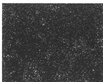
Silicon Ka1
