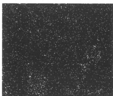
Aluminum Ka1
