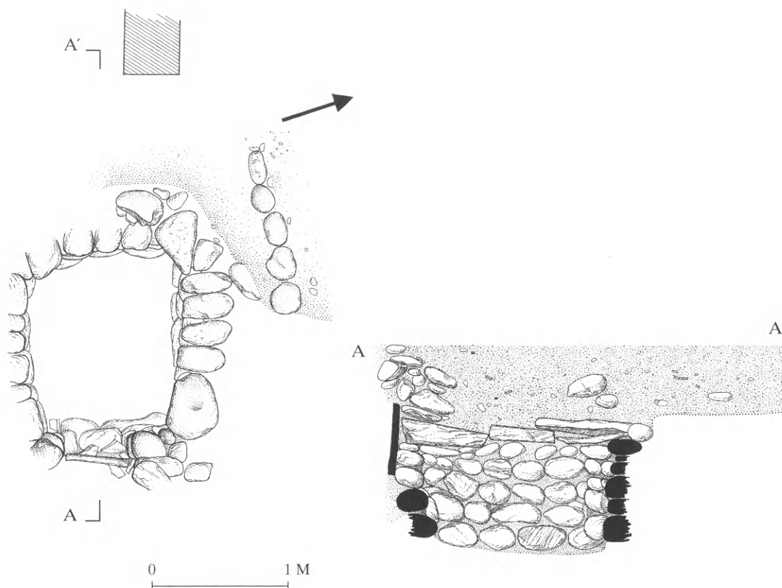
121. Κάτοψη και τομή τοῦ ἀνεσκαμμένου τμήματος τοῦ τάφου 17.
