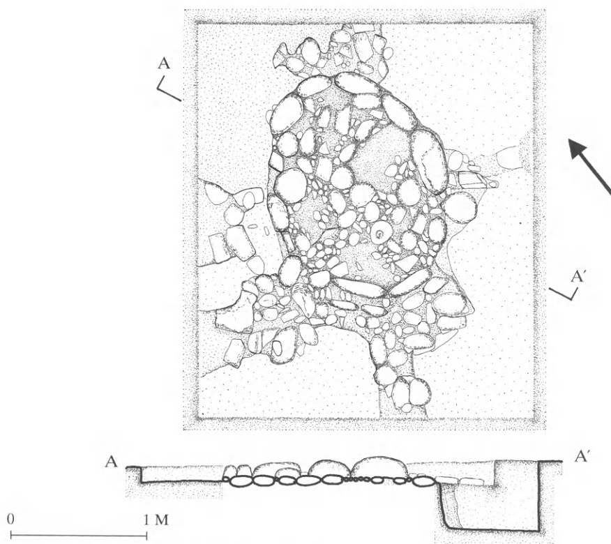
297. Κάτοψη καὶ τομὴ Α-Α' τοῦ ἐπιφανειακοῦ στρώματος τοῦ τάφου 65.
