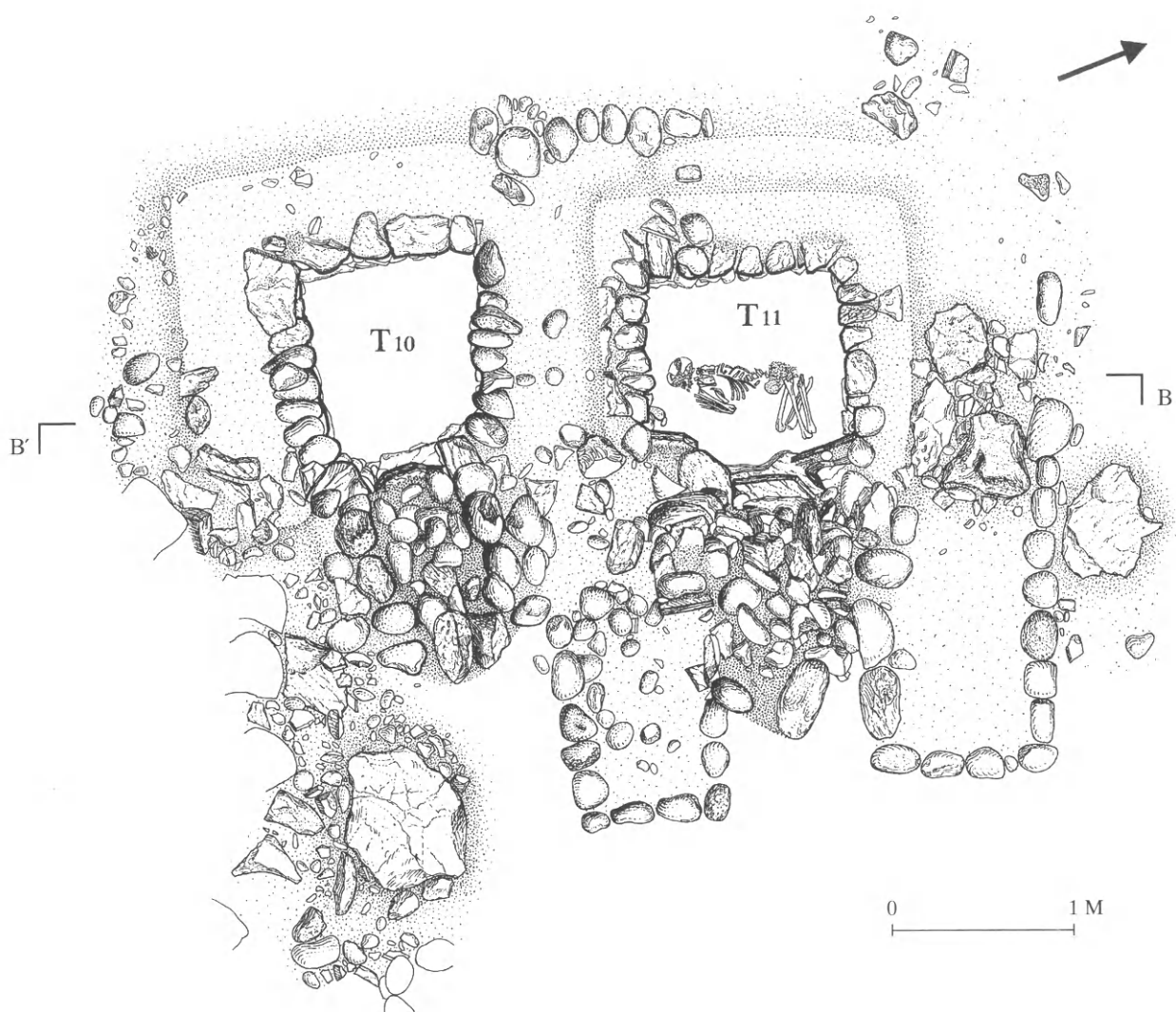
67. Κάτοψη τῶν παραπλεύρων τάφων 10 καὶ 11.
