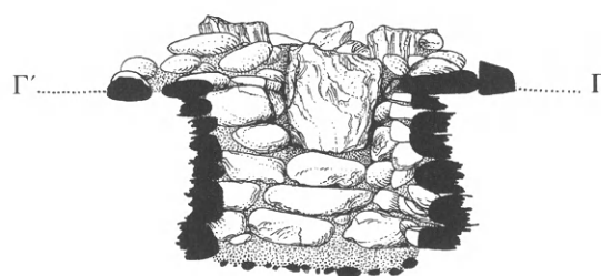
61. Τομή Γ-Γ του τάφου 9 και όψη της ανατολικής πλευράς με την είσοδο στο μέσον.
