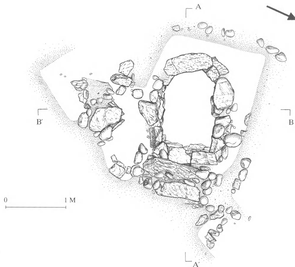
90. Κάτοψη του τάφου 13. Άριστερά, μεγάλες πέτρες με άγνωστη χρήση.
