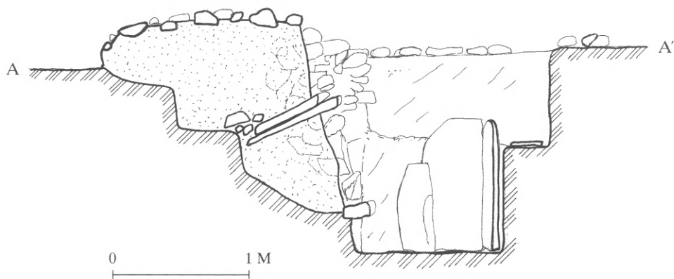
128. Κατὰ μῆκος τομὴ τοῦ ἀνεσκαμμένου προθύρου καὶ τοῦ λάκκου τοῦ τάφου 19.
