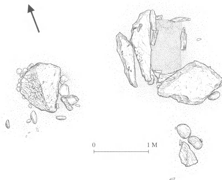
310. Κάτοψη τοῦ τάφου 68 καὶ τῆς περιοχῆς του.
