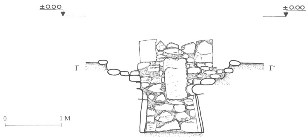
111. Τομή Γ-Γ' και ὄψη τῆς ἀνατολικῆς πλευρᾶς τοῦ τάφου 16.
