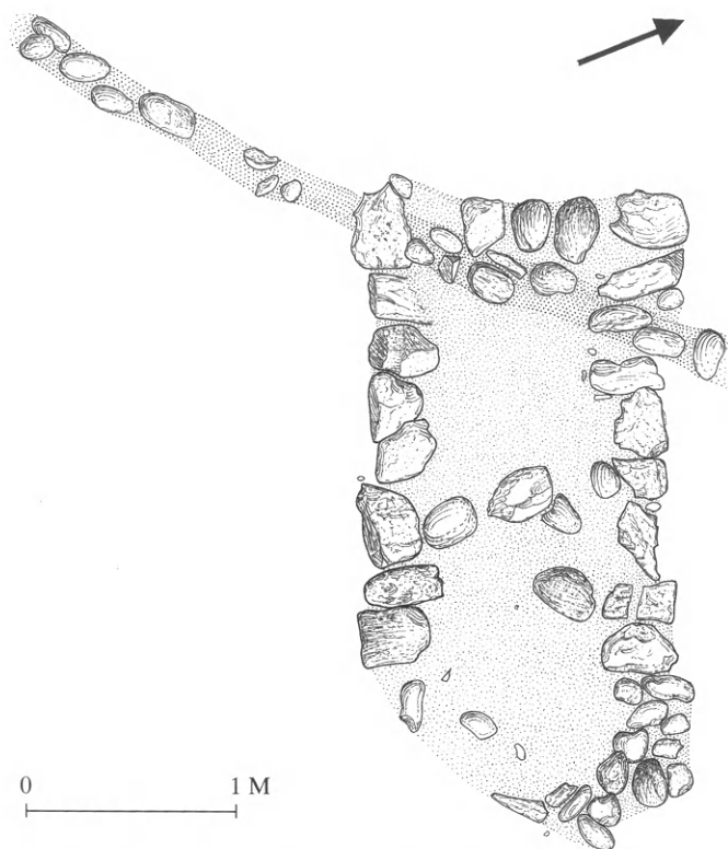
273. Κάτοψη του τάφου 55 και της διερχόμενης λοξῆς σειρᾶς λίθων.
