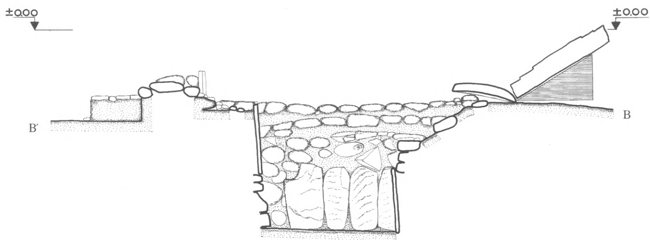
110. Τομή Β'-Β του τάφου 16.
