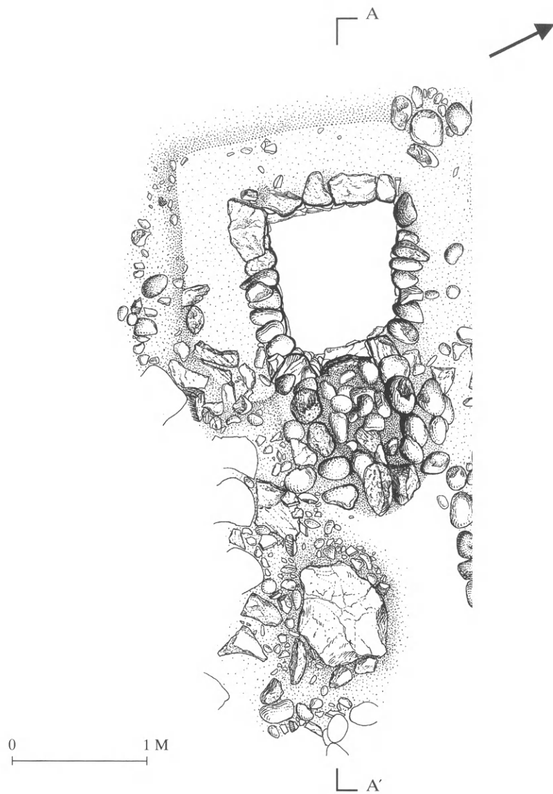
70. Κάτοψη τοῦ τάφου 10. Ἐμπρός, μεγάλη πλάκα κατὰ χώραν.
