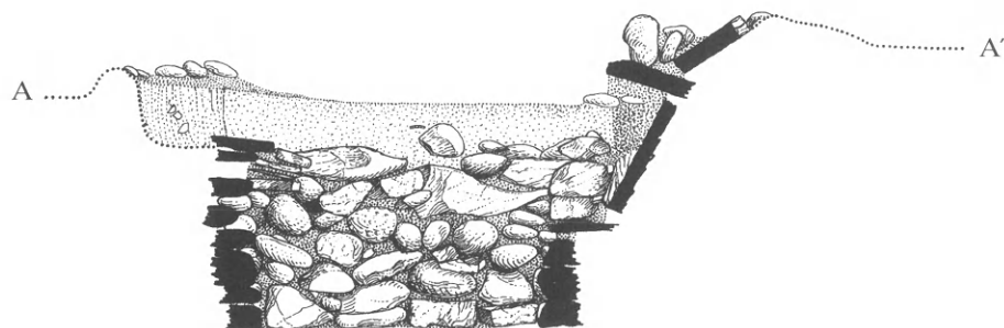
91. Τομή A-A' του τάφου 13.
