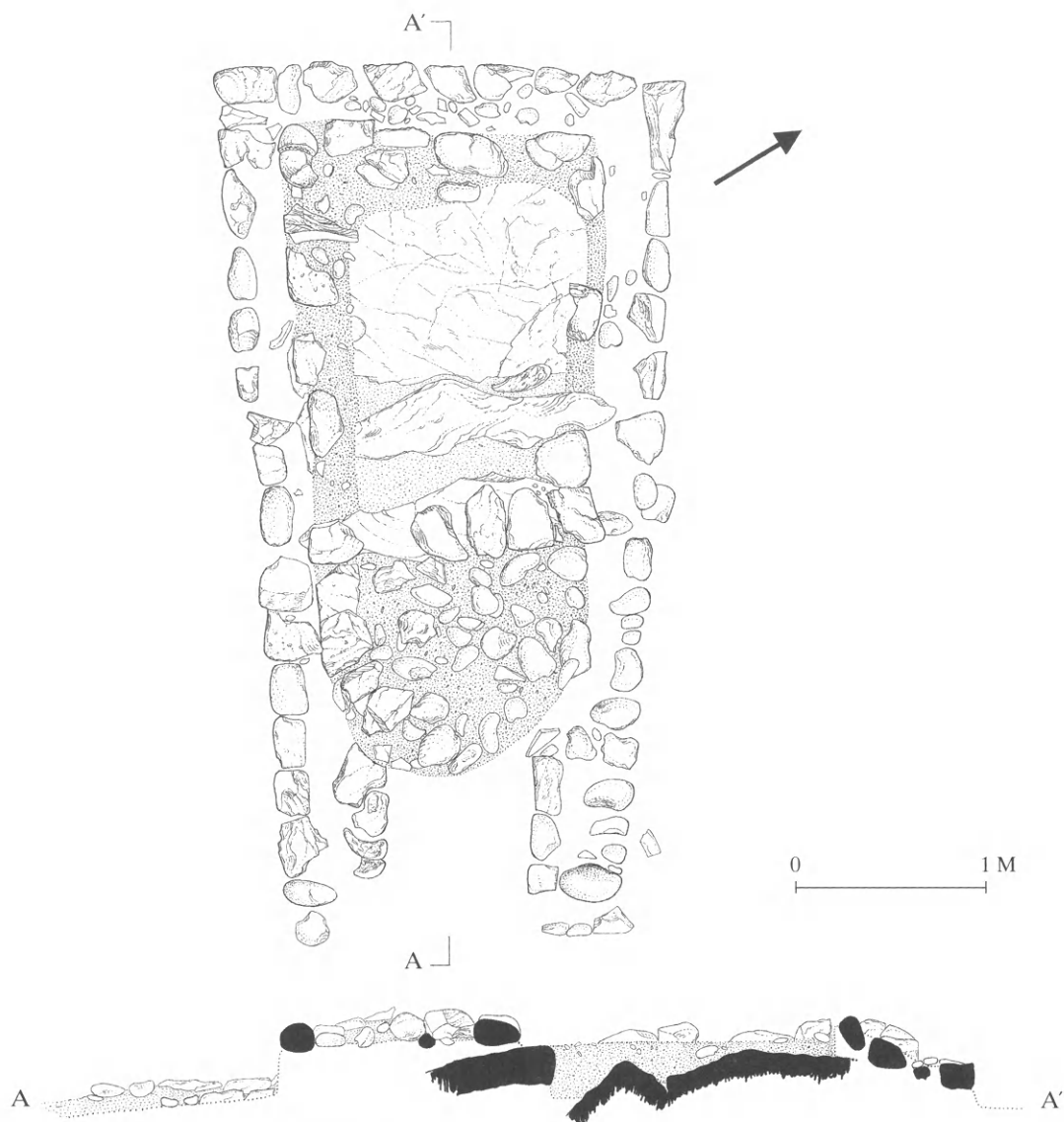
211. Κάτοψη και τομή Α-Α' του τάφου 35.
