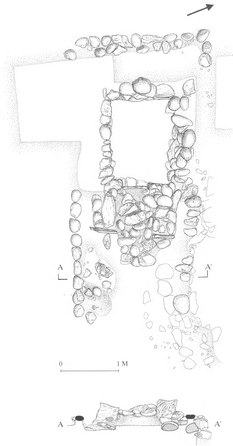
85. Κάτοψη και τομή A-A' τοῦ τάφου 12.
