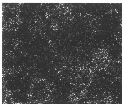
Calcium Ka1
