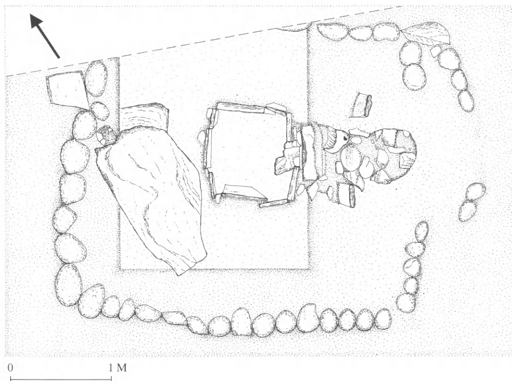
15. Κάτοψη του τάφου 3 με ἄσκαφο προόθυρο.
