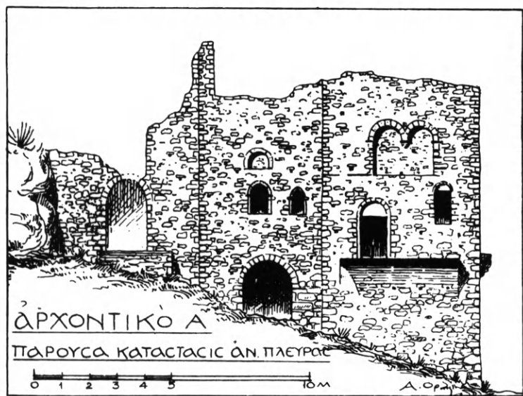
Εἰκ. 89. Ἀνατολικὴ πλευρὰ τοῦ ἀρχοντικοῦ Α.
