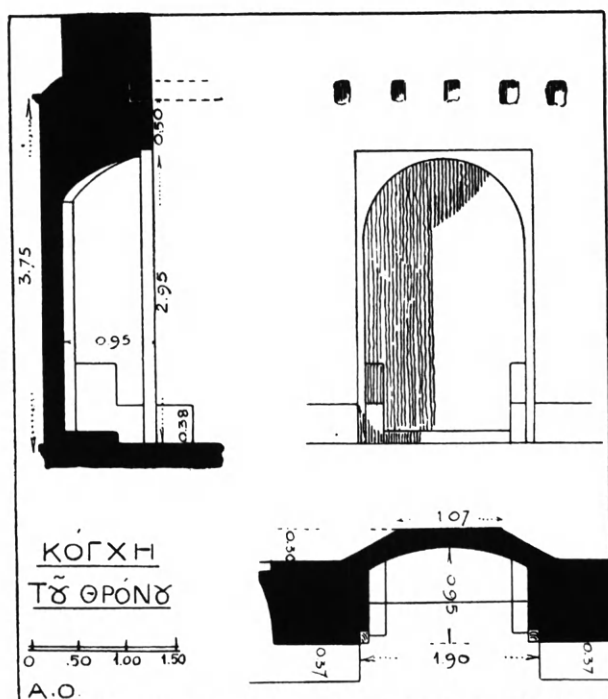
Εἰκ. 42. Ἡ κόγχη τοῦ θρόνου. Κάτοψις, τομὴ καὶ ὀρθωσις.
