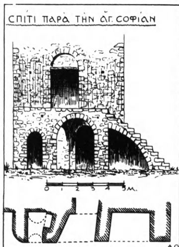
Εἰκ. 51. Ἐξωτερικὴ κλίμαξ ἐπὶ τόξων (Ἄνω Χώρα).
