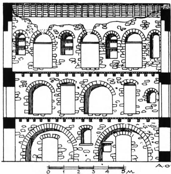
Εἰκ. 94. Σπίτι Γ. Τομή κατακόρυφος.
