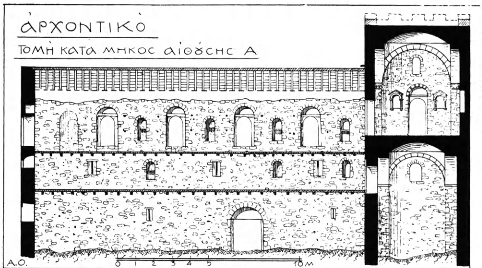
Εἰκ. 87. Τομή κατὰ μῆκος τῆς αἰθούσης Α τοῦ ἀρχοντικού.
