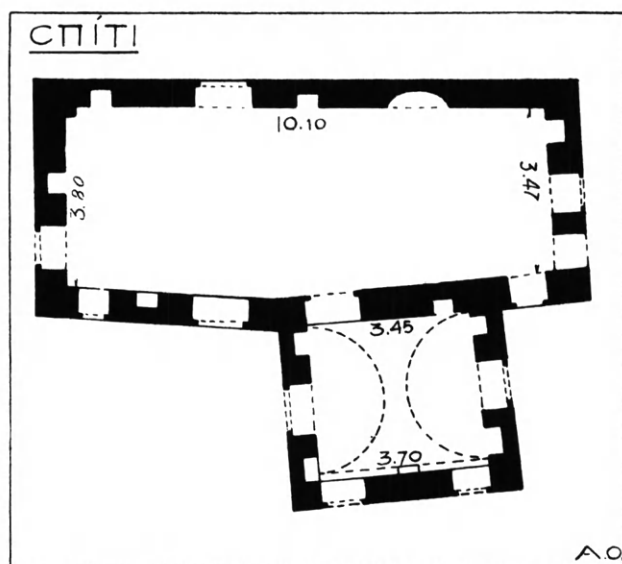
Εἰκ. 91. Κάτοψις τοῦ σπιτιοῦ Β.
