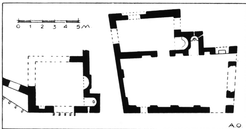
Εἰκ. 68. Αἶθουσαι μετ' ἀποχωρητηρίων.
