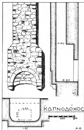
Εἰκ. 32. Ὅφεις καὶ τομαὶ καπνοδόχου τῆς νοτίας πτέρυγος (Ε).
