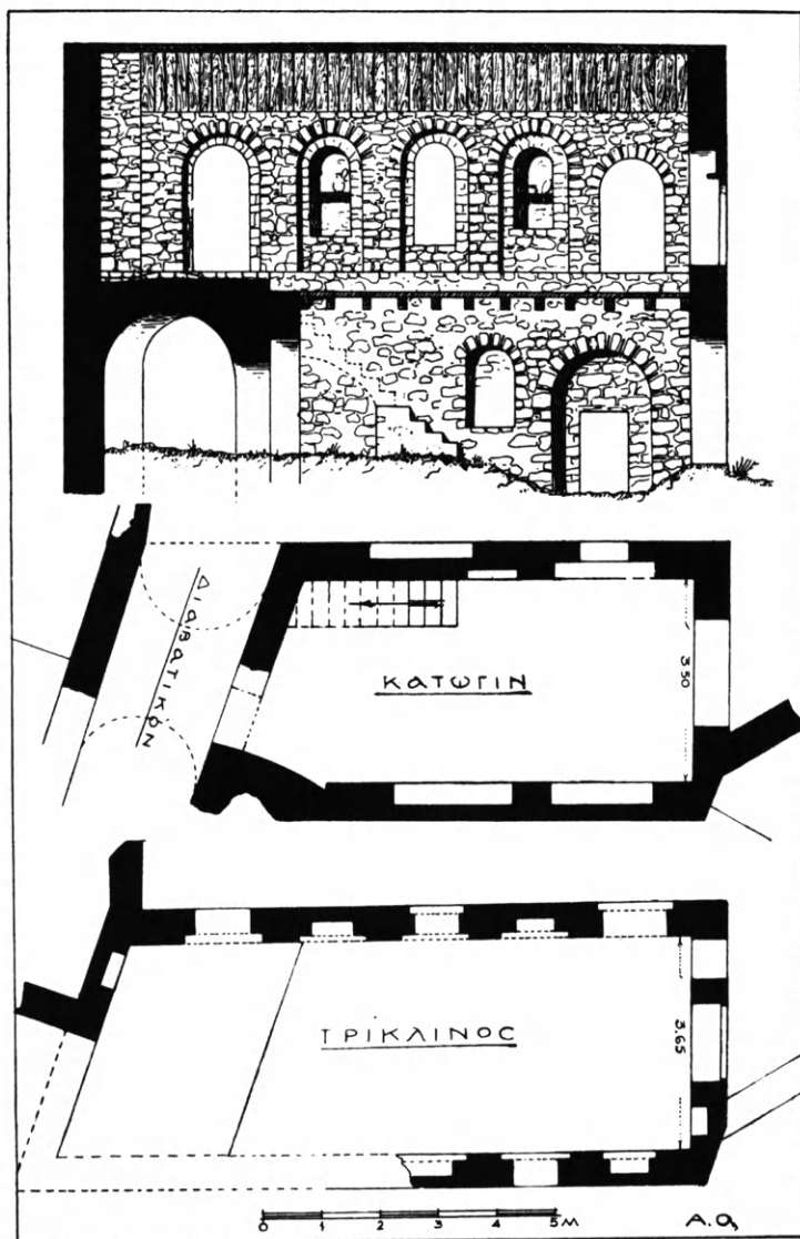
Εικ. 49. Σπίτι άνωγοκάτωγον (Ε) φέρον κάτωθεν λοξόν διαβατικόν.
