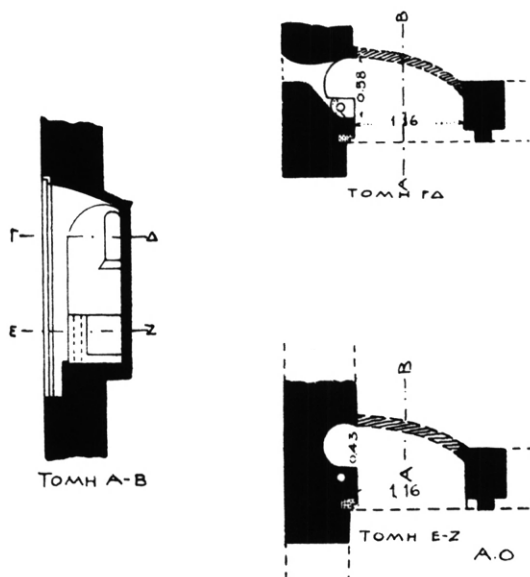
Εἰκ. 19. Κατακόρυφος καὶ ὁριζόντιοι τομαὶ τοῦ παρεκκλησίου.
