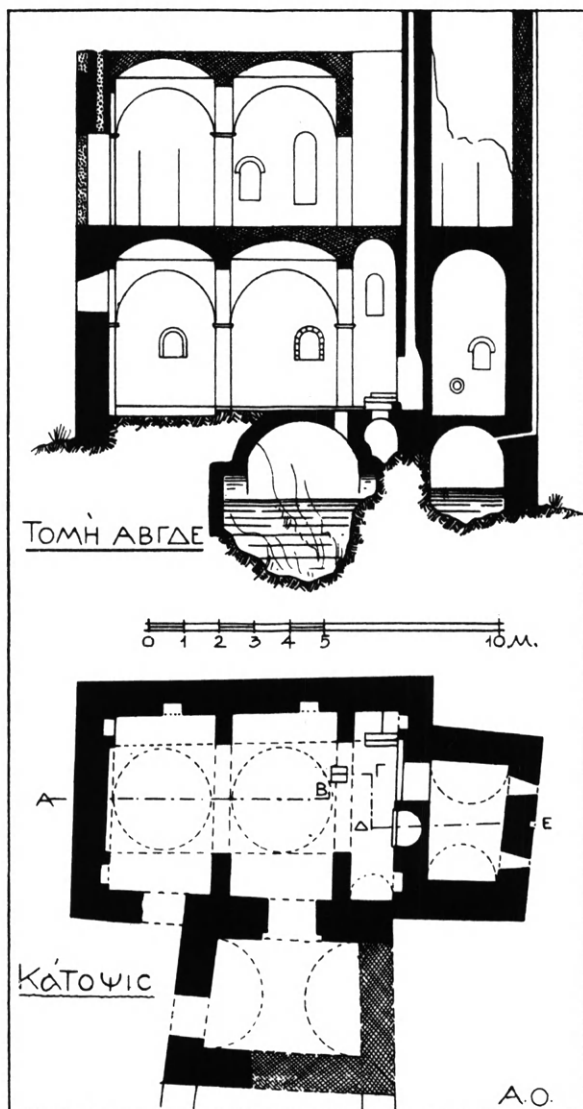
Εἰκ. 14. Κάτοψις καὶ τομὴ τοῦ διαμερίσματος Β.
