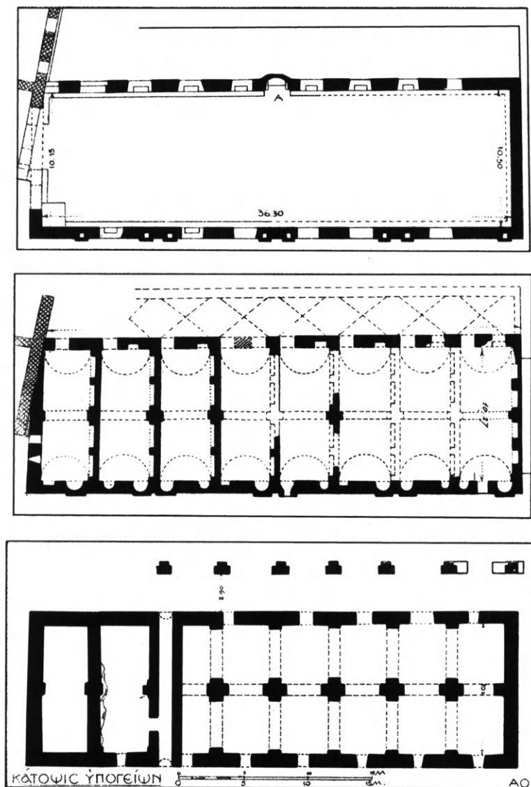
Είχ. 28. Κατόψεις υπογείου και όρόφων της νοτίας πτέρυγος (Ε).
