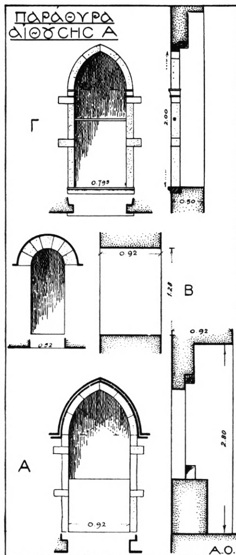
Εικ. 11. Παράθυρα της αίθουσας Α και του ὑπερθέν αὐτῆς ὀρόφου.
