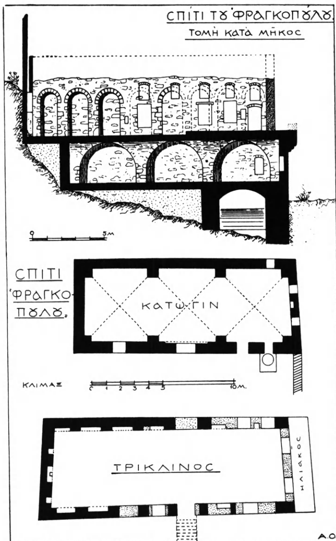
Εἰκ. 98. Κατόψεις καὶ τομὴ τοῦ σπιτιοῦ τοῦ Φραγκοπούλου.
