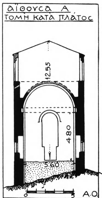
Εἰκ. 12. Κατὰ πλάτος τομὴ τῆς αἰθούσης Α καὶ τοῦ ὑπερθεῖν ὀρόφου.
