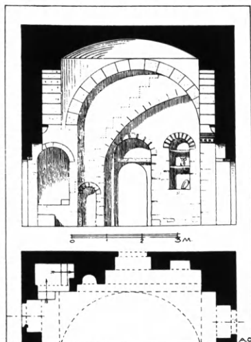
Εἰκ. 52. Κλίμαξ εὐθεῖα ἐντὸς τοίχου τοῦ ἀρχοντικοῦ Α.
