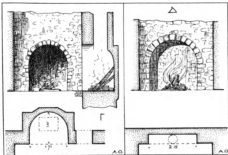
Εἰκ. 65. Ἑστίαι σπιτιῶν τοῦ Μυστρά.
