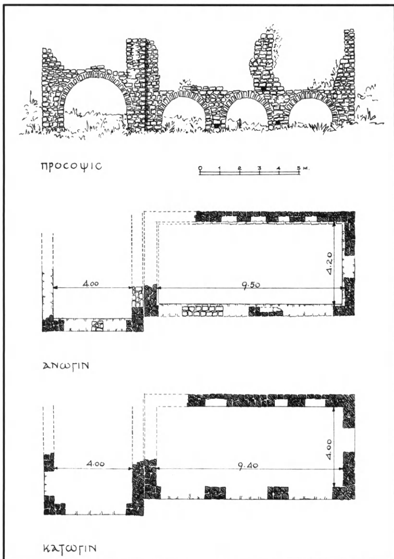
Εἰκ. 114. Σχέδιον ὀρόφων καὶ πρόσοψις σπιτιοῦ εἰς Κάτω Χώραν.
