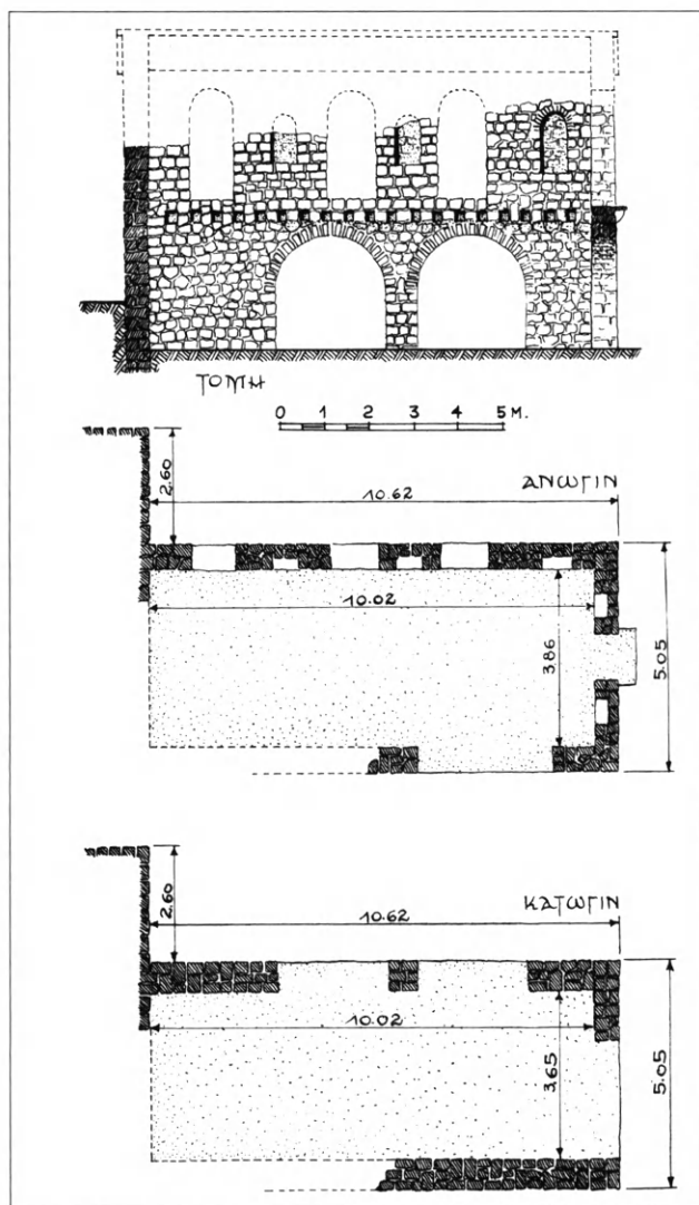
Εἰκ. 111. Σχέδιον ὀρόφων καὶ τομῇ σπιτιοῦ τῆς συνοικίας Ἁγίας Σοφίας, νοτιοδυτικῶς τοῦ ἀρχοντικοῦ.
