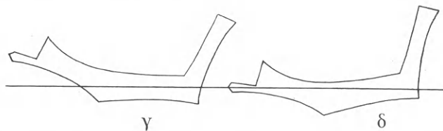
90. α. Έγχρωμη ἀπεικόνιση πλοίου σὲ πρωτοκυκλαδικὸ σκεῦος, β. Σχέδιο τοῦ πλοίου, γ. Ἴσαλος γραμμὴ κατὰ τὸ σχέδιο, δ. Ἴσαλος γραμμὴ κατὰ τὴν ὀρθὴ θέσιν τοῦ πλοίου.
