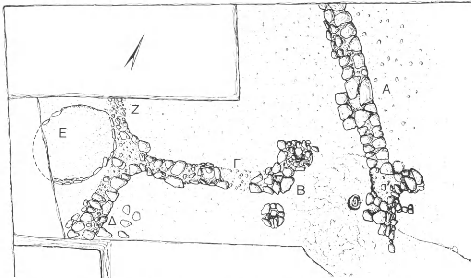
25. Κάτοψη τοίχων οικίας της Μέσης Νεολιθικής στη Νέα Μάκρη (κάτω) και αναπαράσταση της οικίας με ενδείξεις κατασκευής (άνω).
