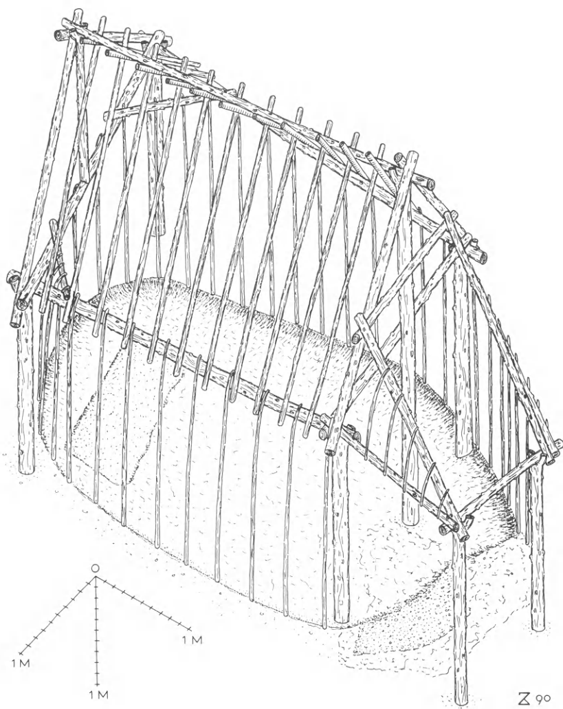
56. Αναπαράσταση του ξύλινου σκελετού της καλύβας, εικ. 53-54.
